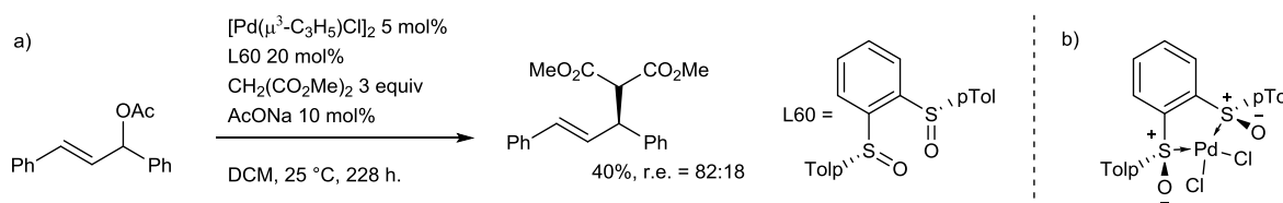
Figure III-86 : ligand bis-sulfoxyde énantiopur dans une réaction de Tsuji-Trost
