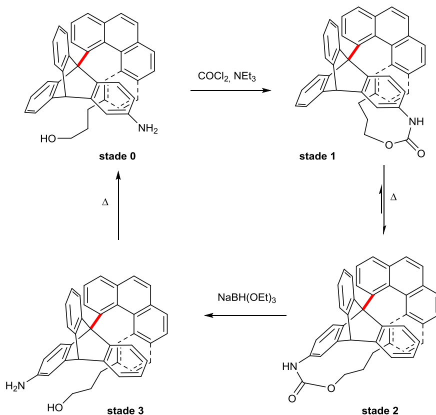
Figure III-81 : premier moteur moléculaire atropisomérique
