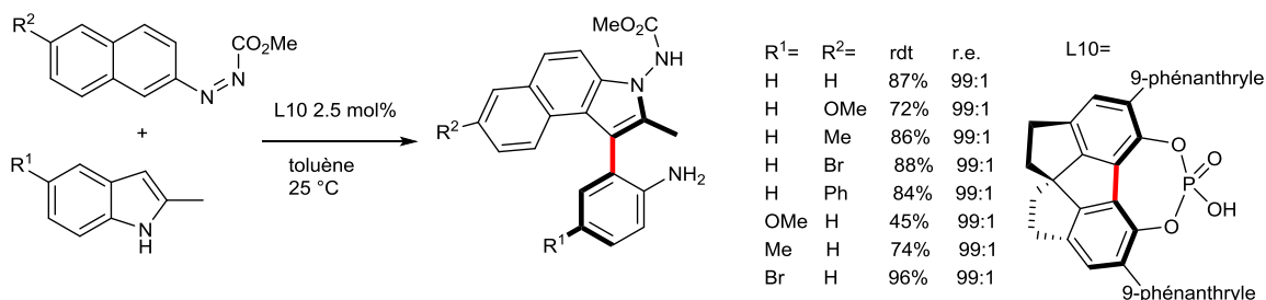
Figure III-28 : arylation organocatalytique utilisant des indoles
