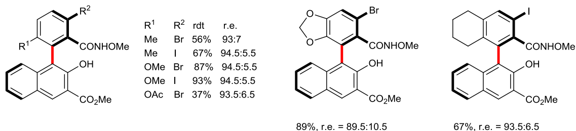
Figure III-31 : couplage intermoléculaire atroposélectif
