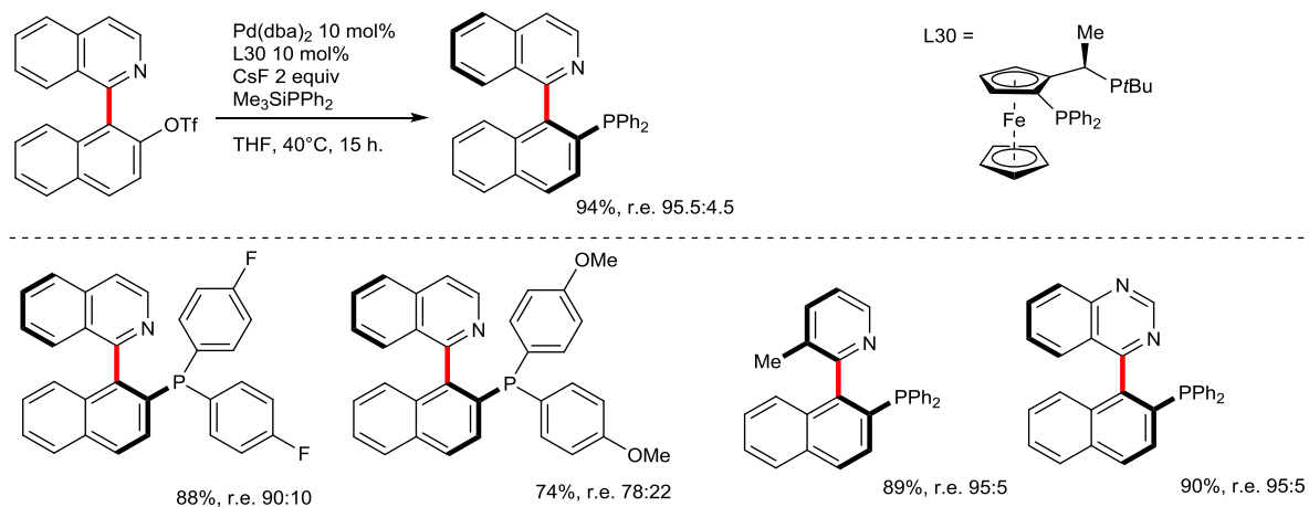
Figure III-59 : phosphination atropoénantiosélective par DKR dans le groupe Lassaletta
