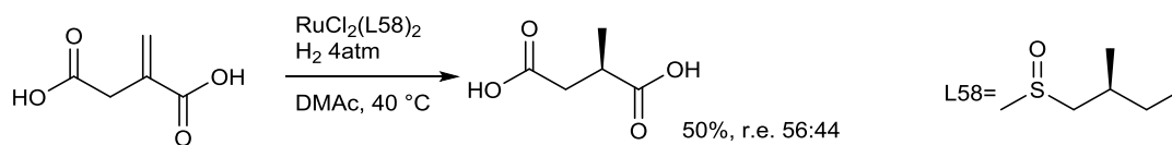
Figure III-84 : première réaction énantiométrique utilisant un ligand sulfoxyde
