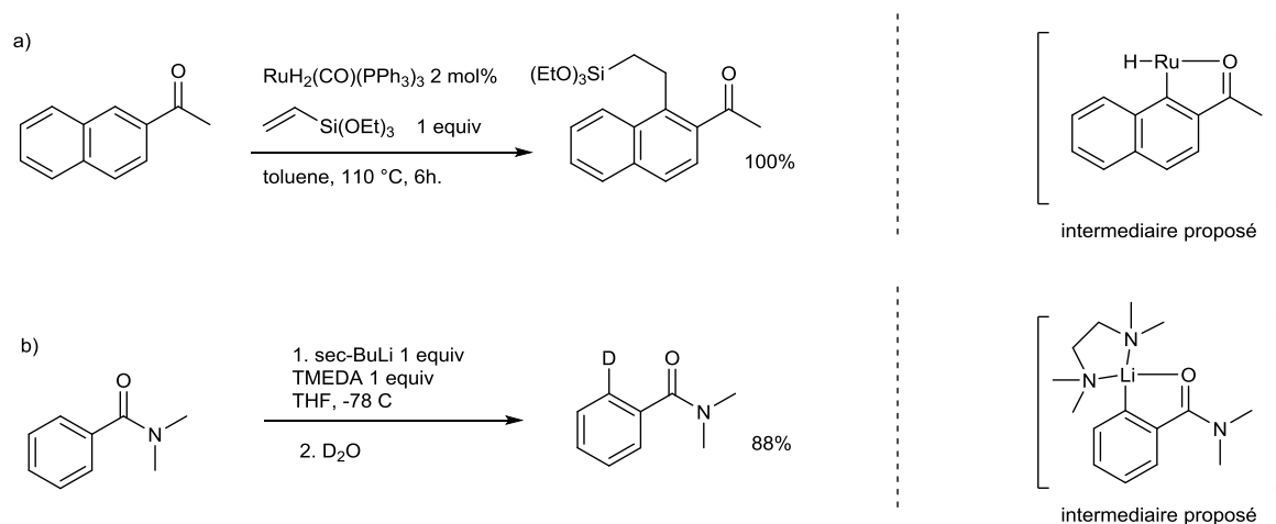
Figure III-1 activation C-H et métallation dirigée en ortho
