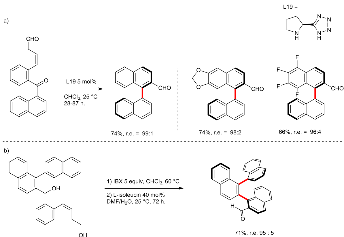
Figure III-42 : condensations aldoliques atroposélectives organocatalytiques
