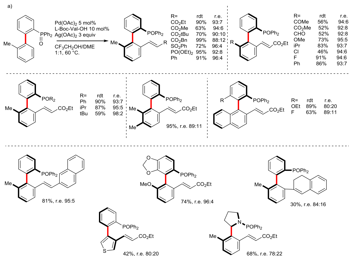
Figure III-53 : oléfination atropénantiosélective avec un oxyde de phosphine comme DG
