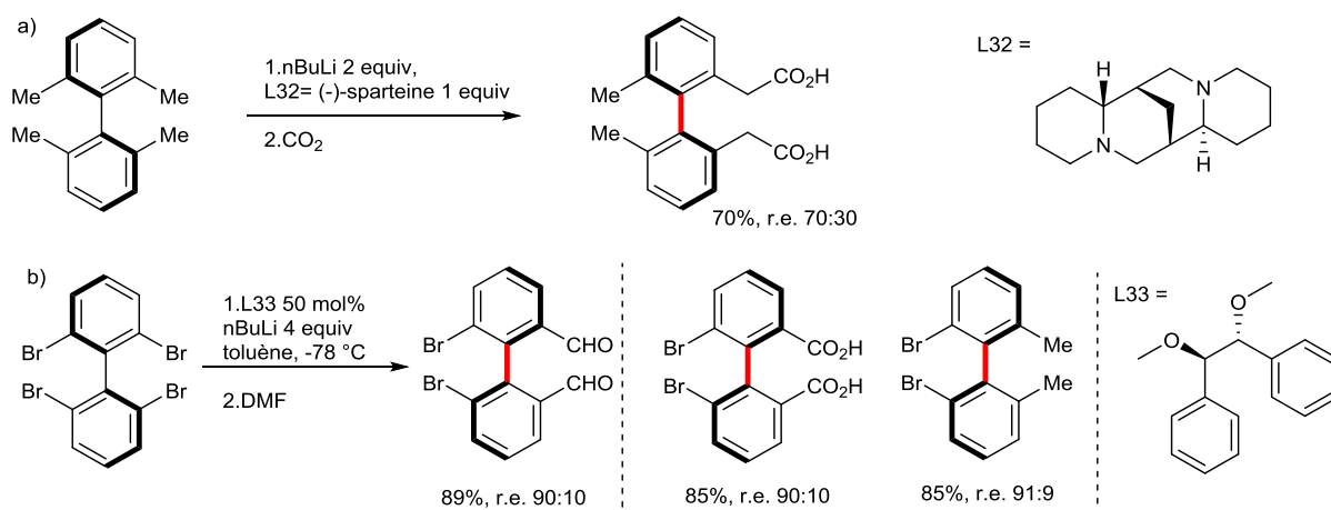
Figure III-63 : désymétrisation atroposélective par des bases lithiées
