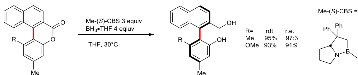
Figure III-64 : concept « de la lactone »
