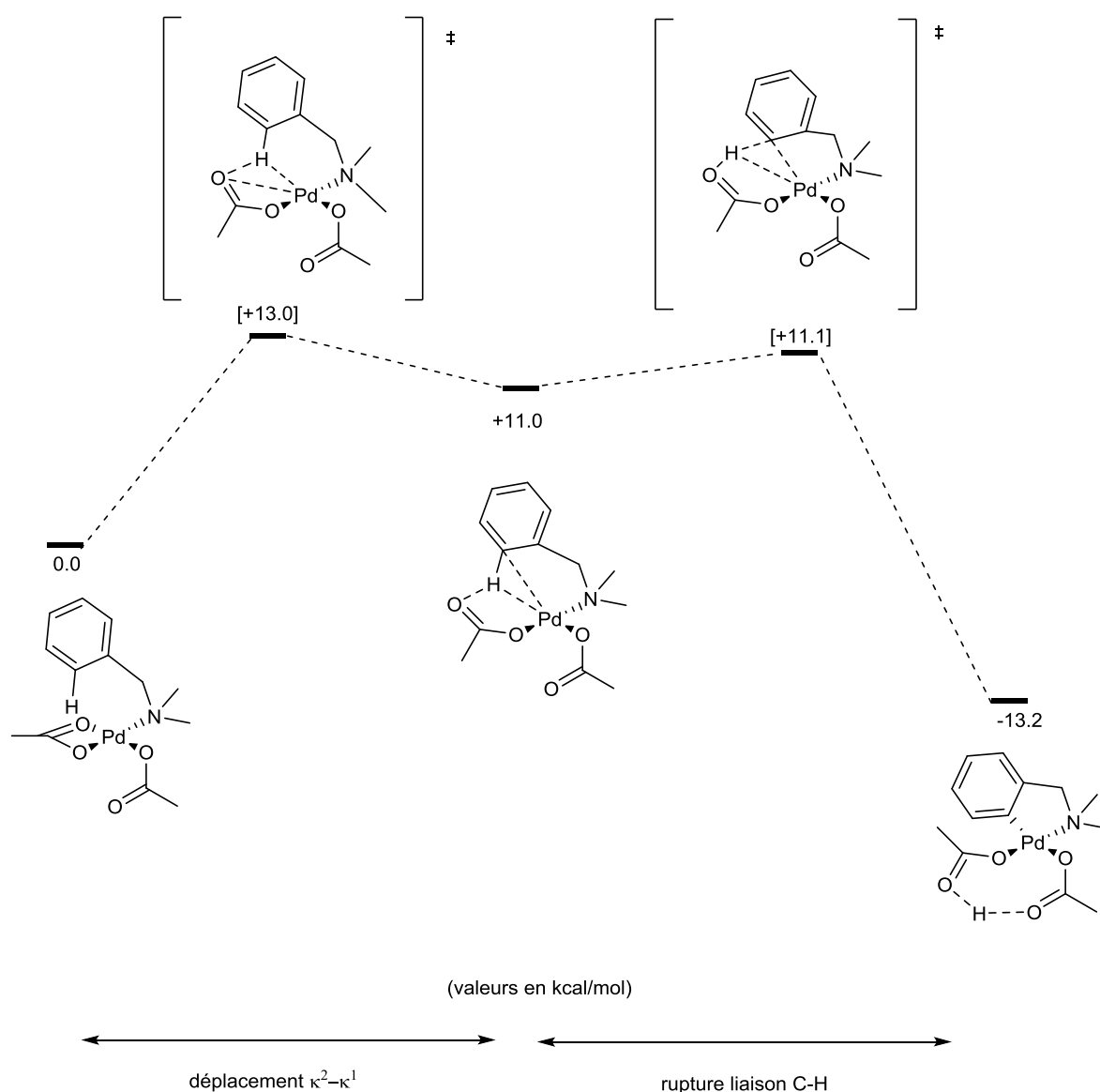
Figure III-8 : mécanisme de la cyclopalladation de la N,N -diméthylbenzylamine
