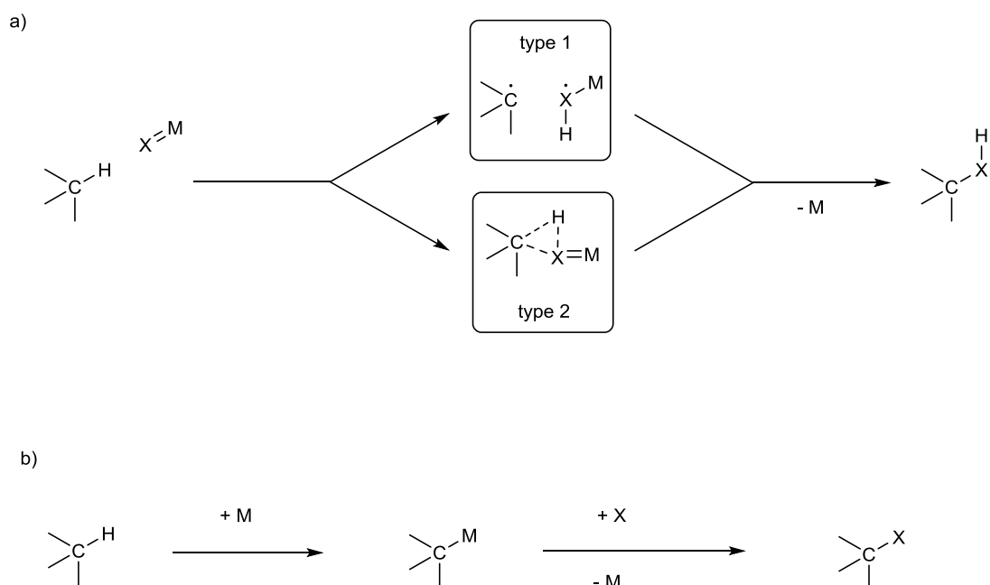
Figure III-2 : mécanismes par sphère interne et externe
