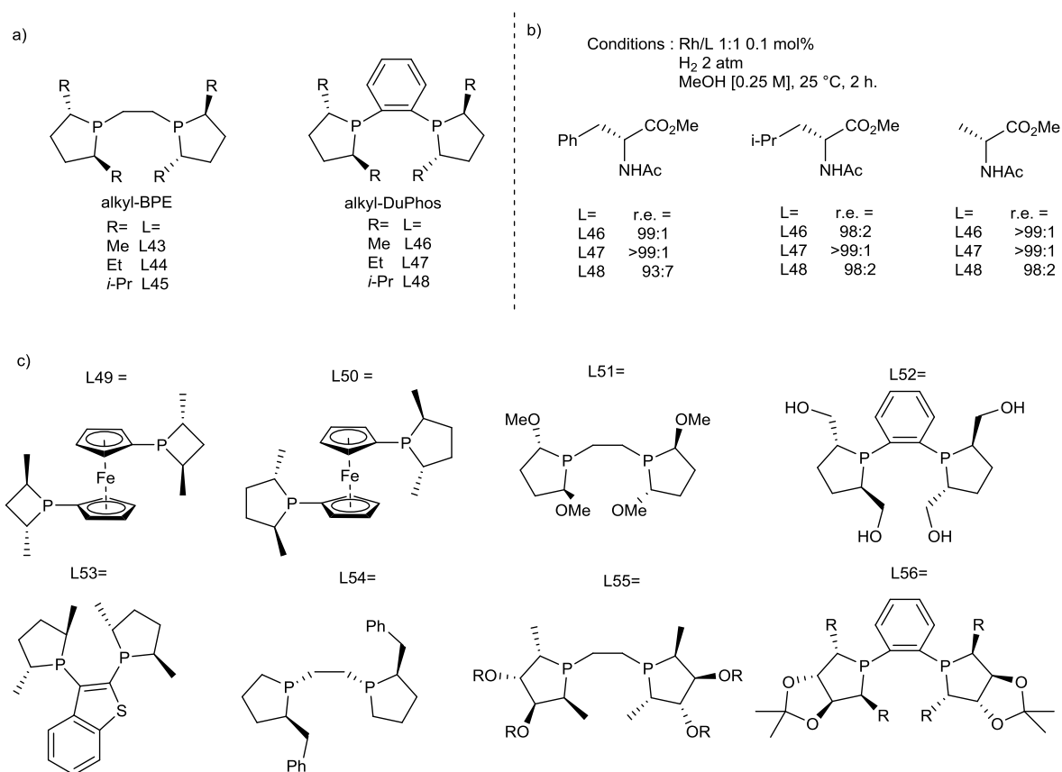
Figure III-79 : première apparition et famille de ligands de type « DuPhos »
