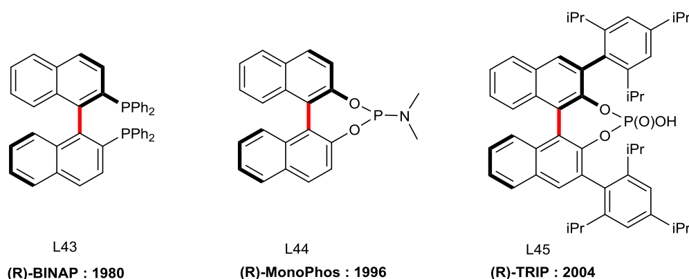
Figure III-78 : famille de ligands dérivés de la BINAP
