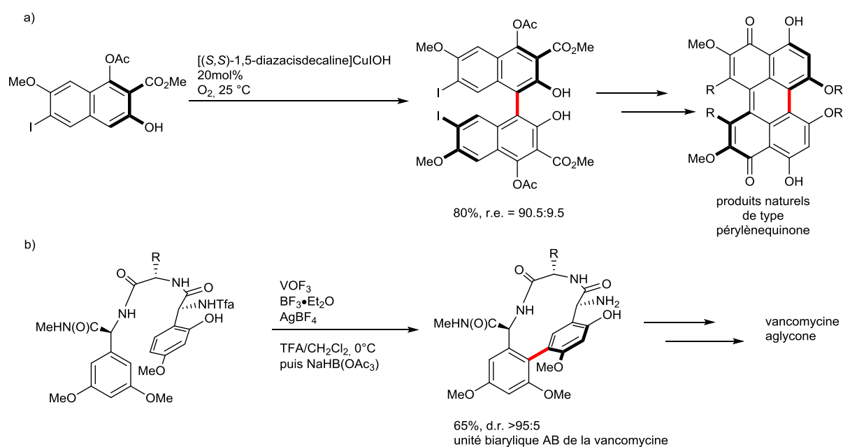
Figure III-25 : produits naturels obtenus par couplage oxydant
