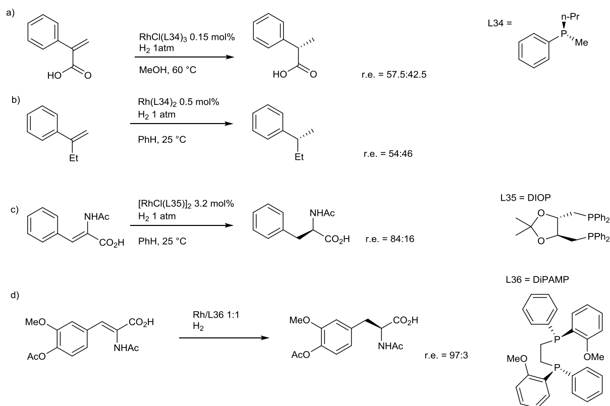
Figure III-73 : exemples précoces de catalyse homogène asymétrique avec des phosphines
