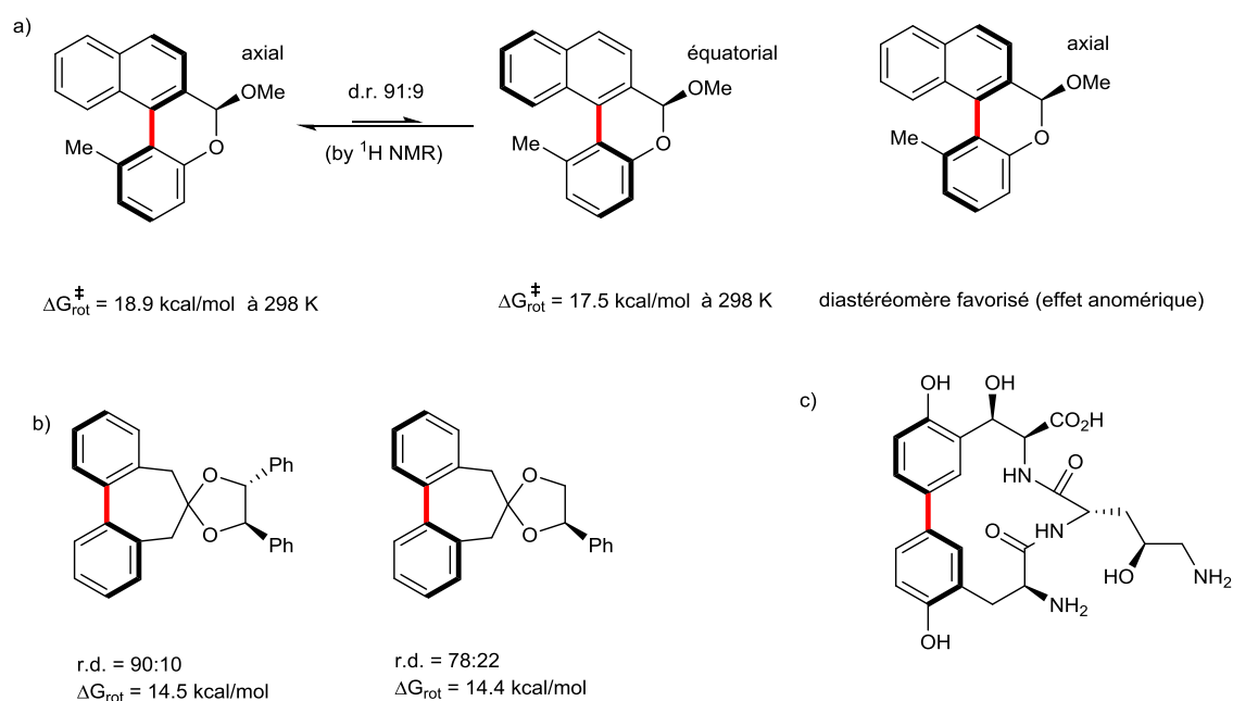
Figure III-22 : influence des substituants pontants stéréogènes
