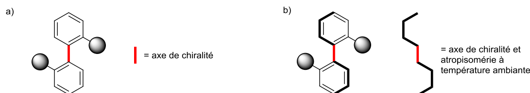
Figure III-16 : formalisme graphique concernant l'atropisomérisation
