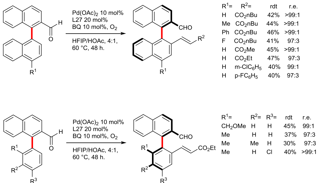
Figure III-55 : oléination atropoénantiosélective par KR grâce à un groupe directeur transitoire
