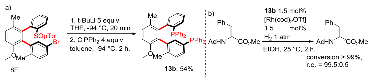
Figure IX-8 : synthèse de ligands originaux et test catalytique
