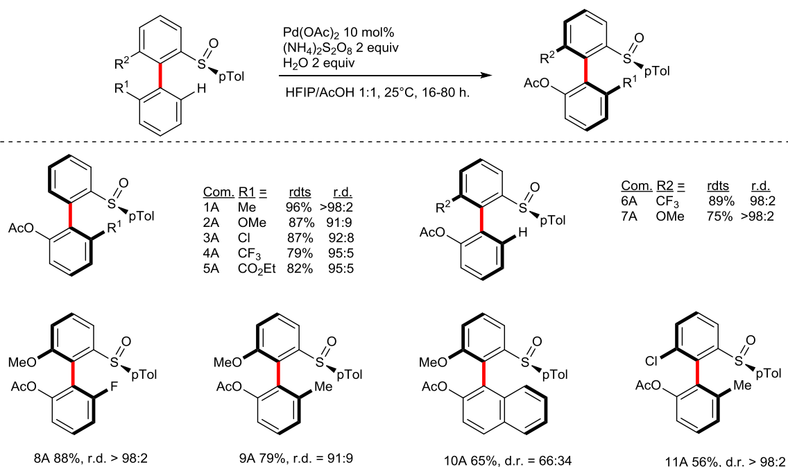
Figure IX-3 : portée de la réaction d'acétoxylation
