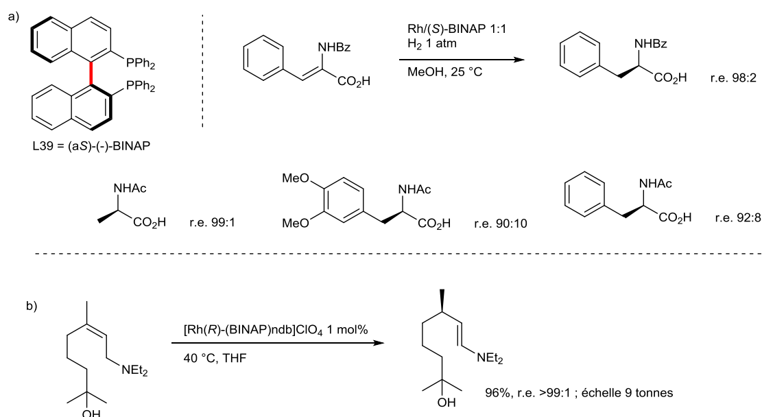
Figure III-75 : première utilisation académique et industrielle de la BINAP
