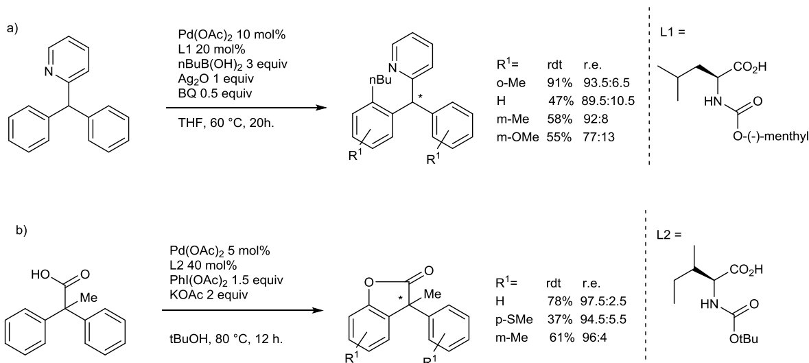
Figure III-11 : activation C-H énantiosélective par désymétrisation
