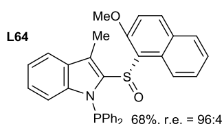
Figure III-87 : exemples de ligands efficaces comportant un sulfoxyde énantiopur
