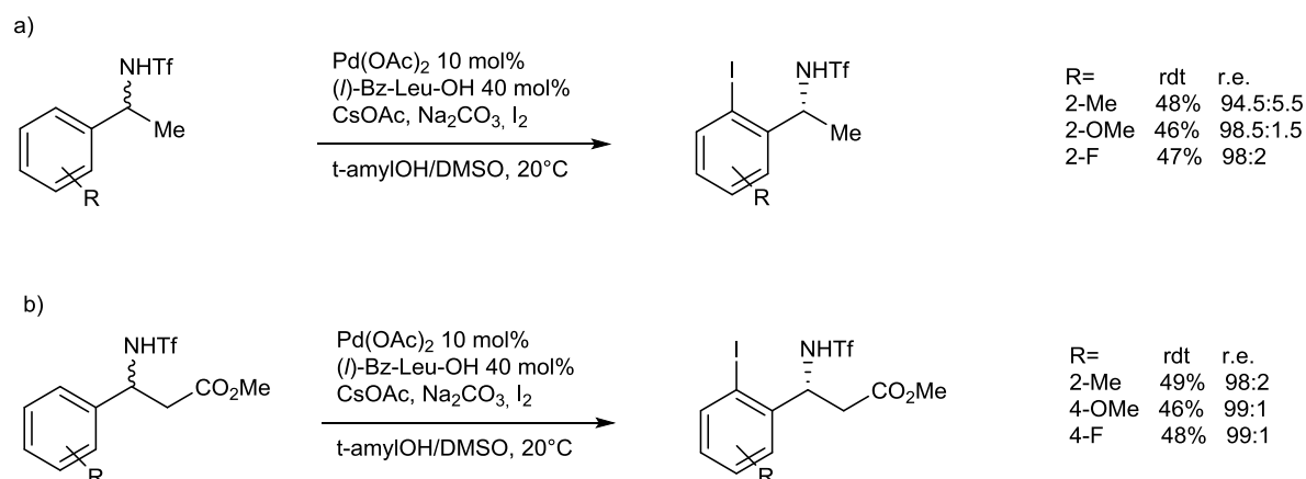
Figure III-13 : déboulement cinétique par C-H activation
