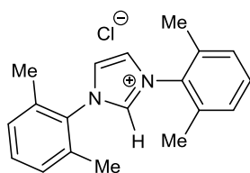
IMeHCl
