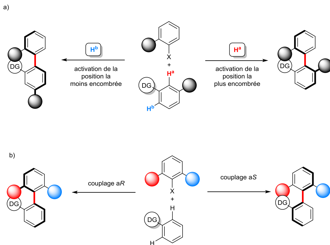
Figure III-32 : défis spécifiques du couplage Ar-Ar atroposélectif
