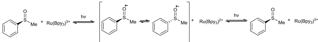
Figure III-105 : racémisation photochimique
