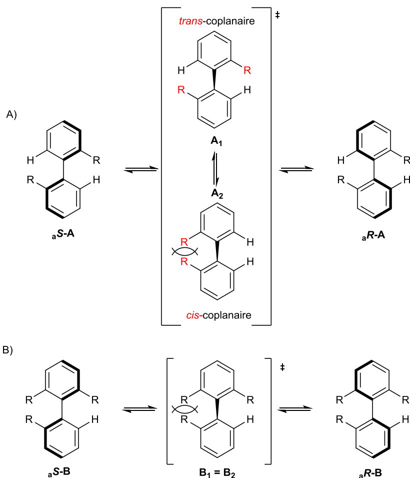
Figure III-18 : mécanisme d'atropisomérisation
