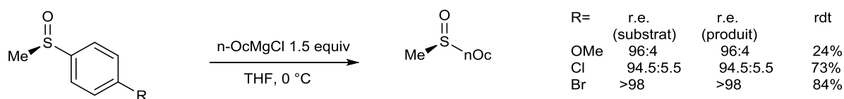
Figure III-112 : échange sulfoxyde/magnésium
