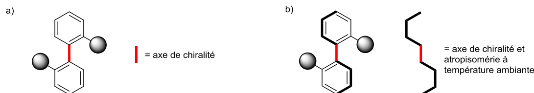
Figure III-16 : formalisme graphique concernant l'atropisomérisation
