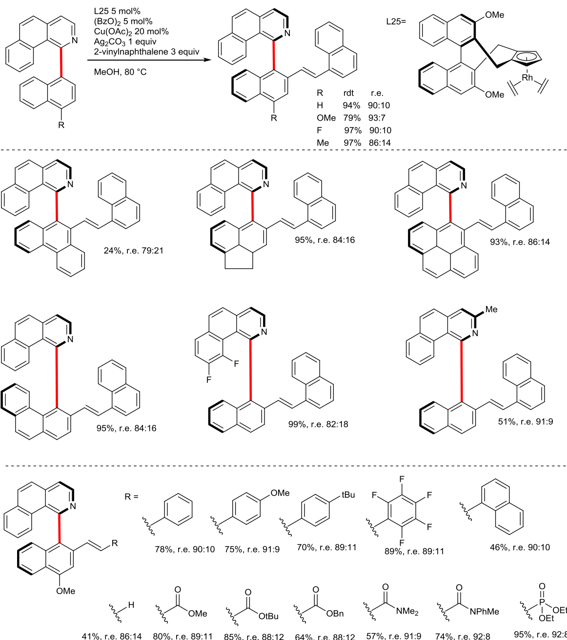
Figure III-50 : oléination aropéantiosélective
