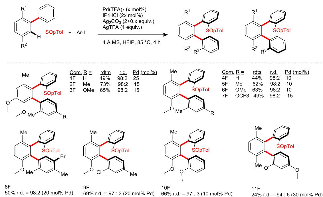
Figure IX-7 : portée de la réaction d'arylation avec double contrôle de chiralité axiale
