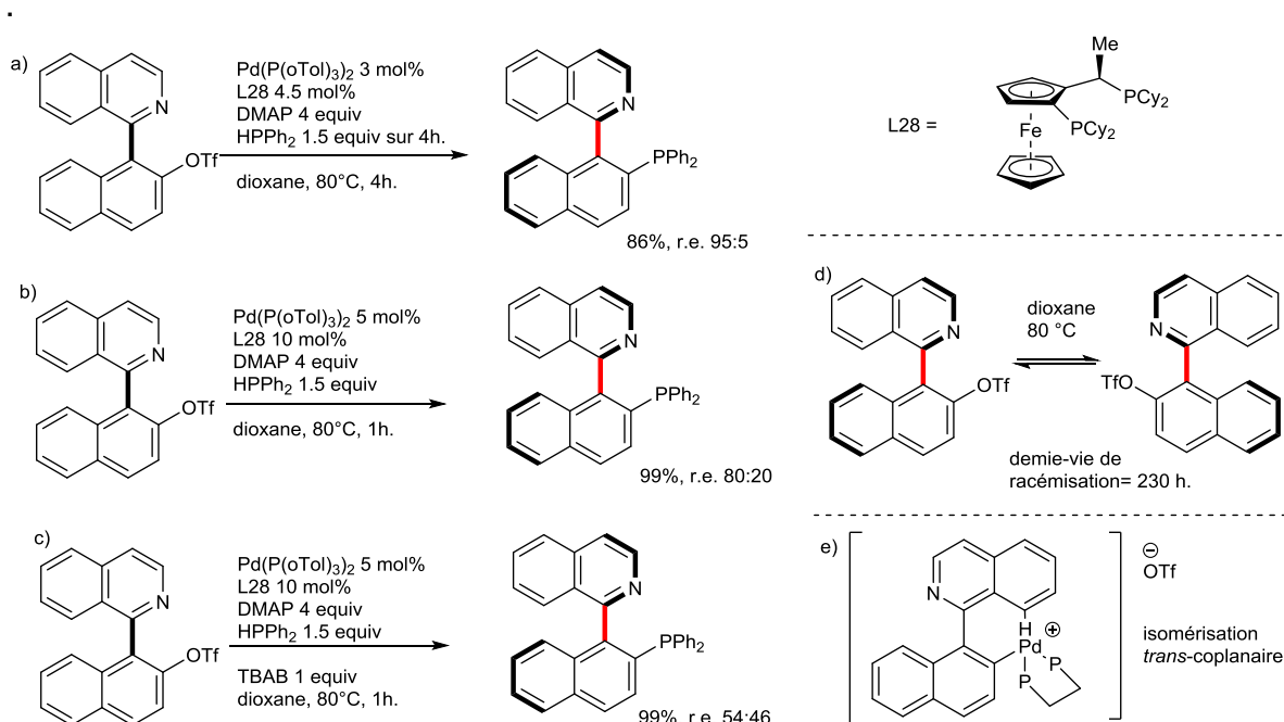
Figure III-57 : phosphination atropoénantiosélective par DKR
