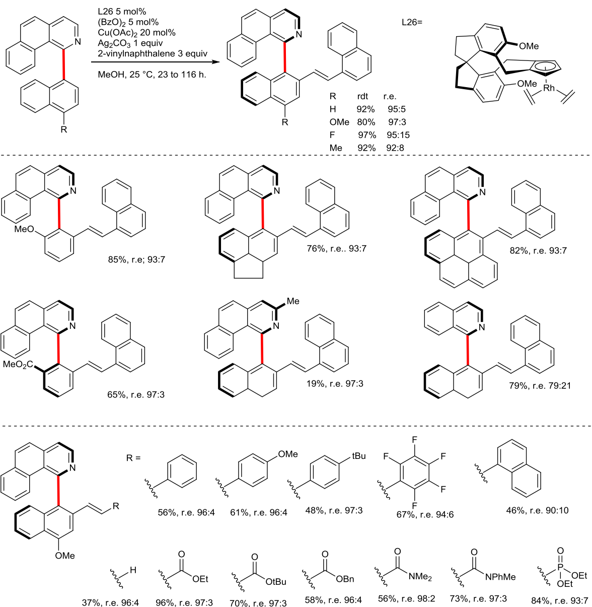
Figure III-52 : oléfination atropoénantiosélective
