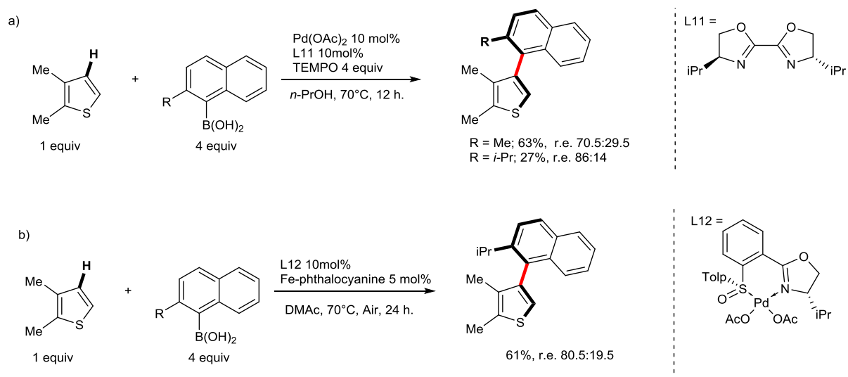
Figure III-30 : arylation directe atroposélective
