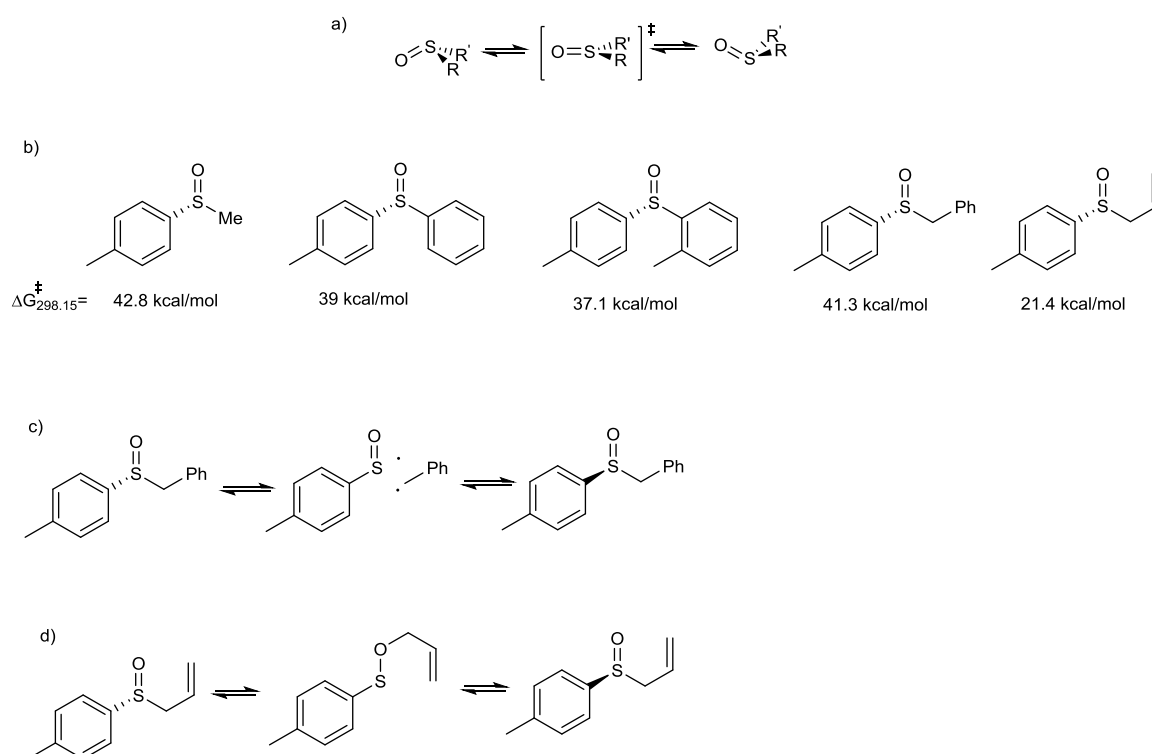
Figure III-103 : inversion pyramidale, barrières d'inversions et autres mécanismes d'épimérisation
