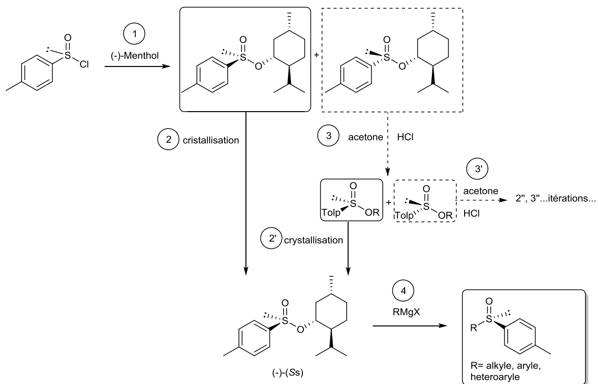
Figure III-100 : schéma générale de la méthode d'Andersen
