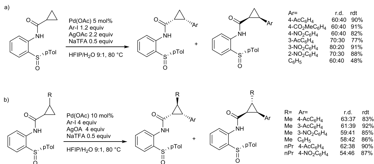
Figure III-96 : arylation diastéréosélective de cyclopropanes
