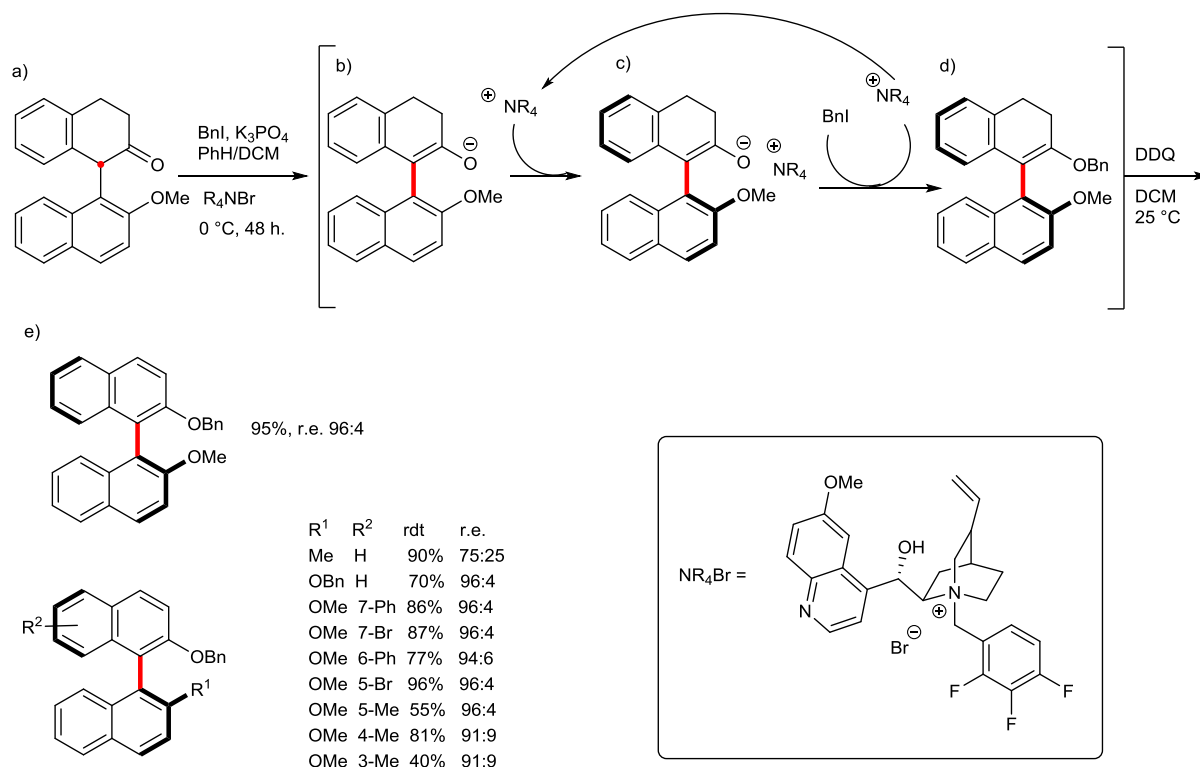
Figure III-44 : O-alkylation atroposélective
