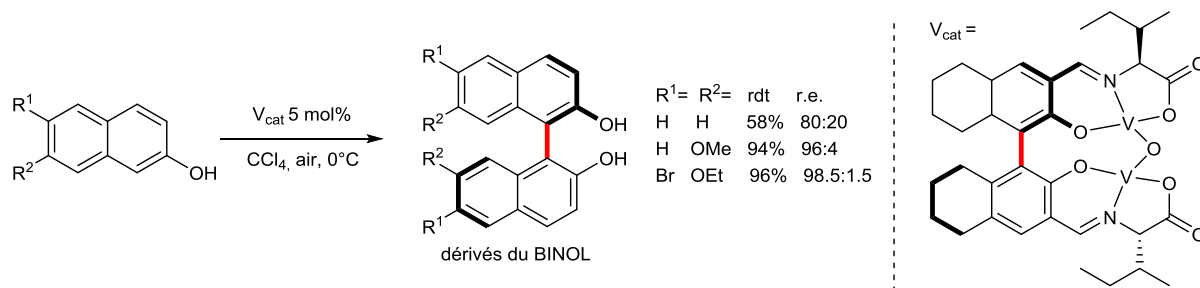
Figure III-26 : couplage oxydant utilisant l'air comme oxydant terminal
