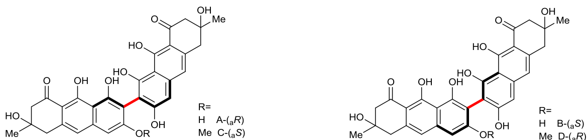
Figure III-71 : isomères des flavomannins A, B, C et D
