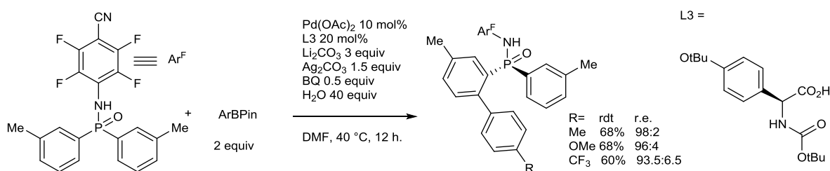
Figure III-12 : obtention de phosphinamides énantioenrichis par activation C-H
