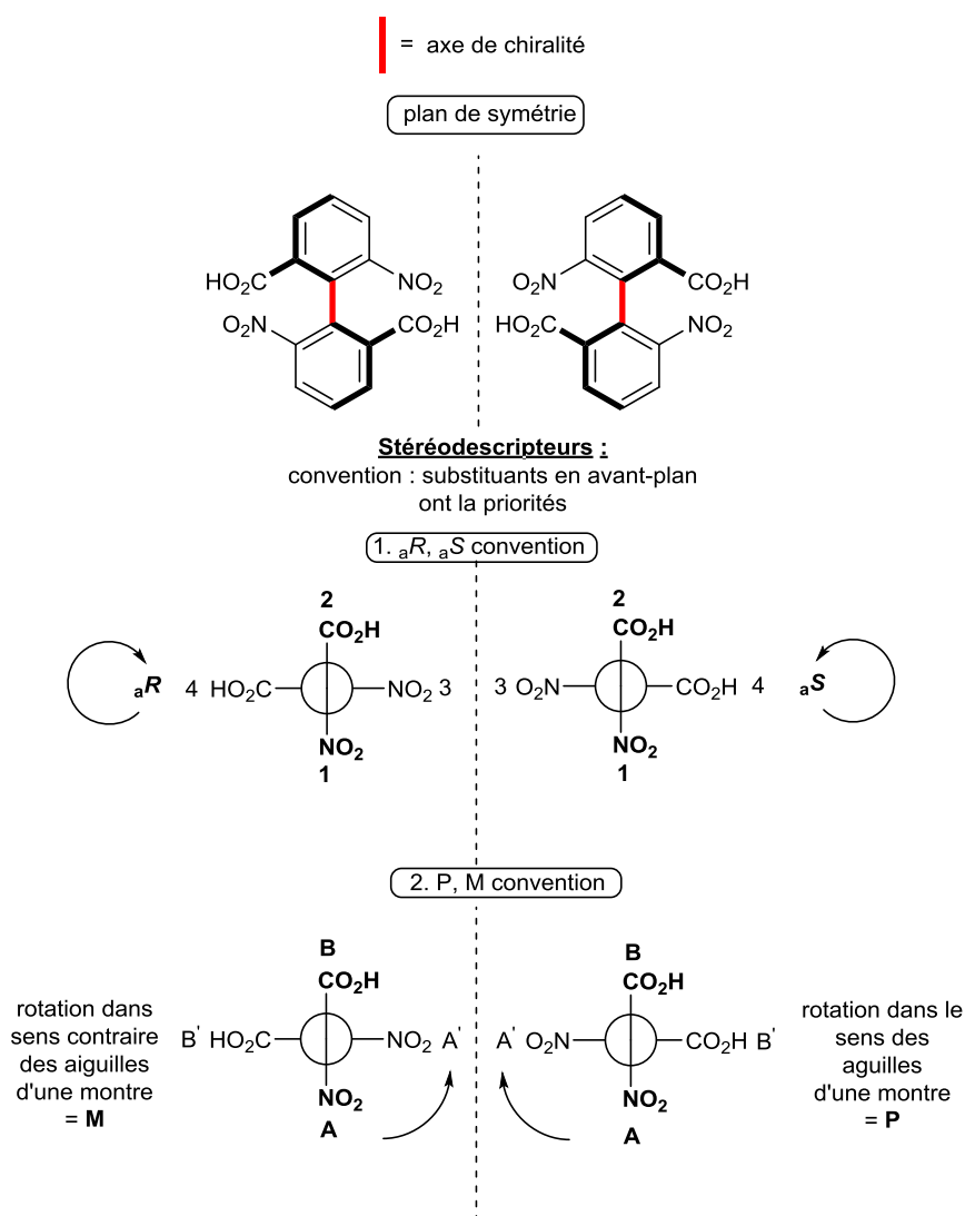
Figure III-15 : convention de chiralité axiale
