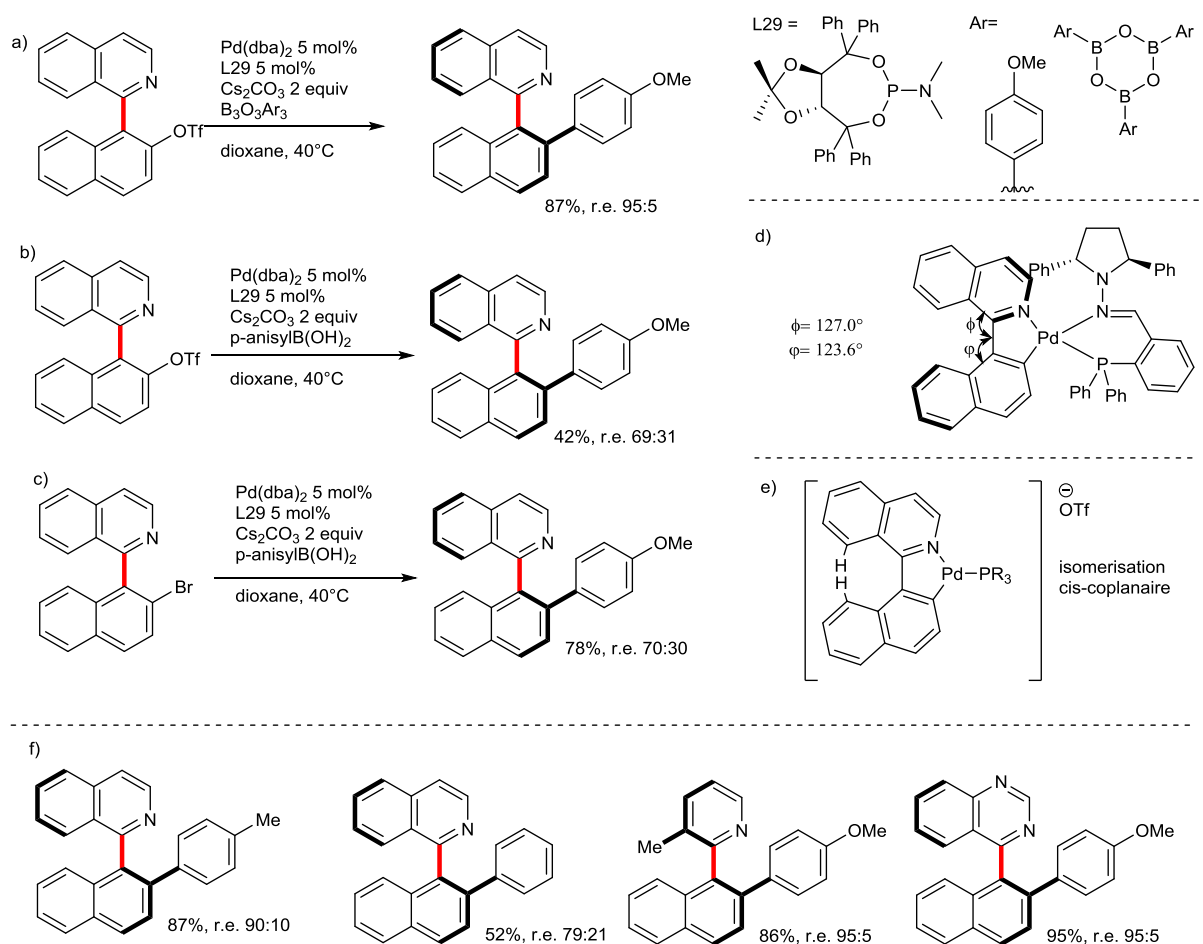
Figure III-58 : arylation atropoénantiosélective par DKR
