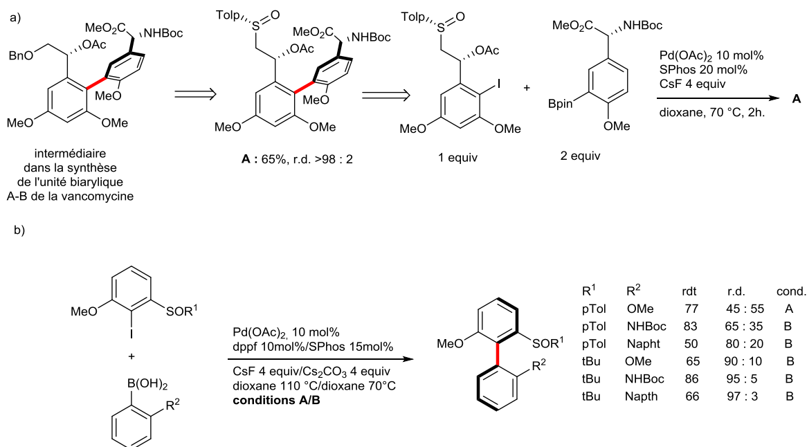
Figure III-33 : couplage atropodiasélectif utilisant un sulfoxyde énantiopur
