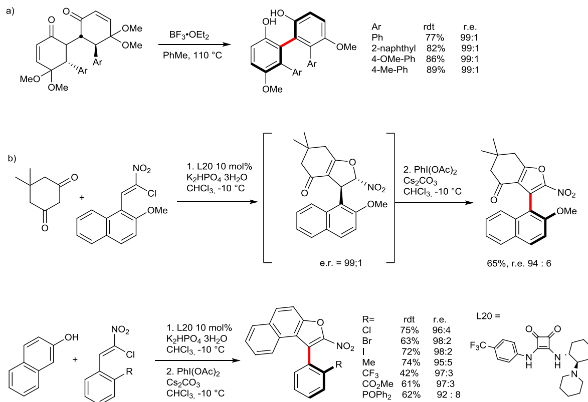
Figure III-43 : transfert de chiralité centrale à axiale.
