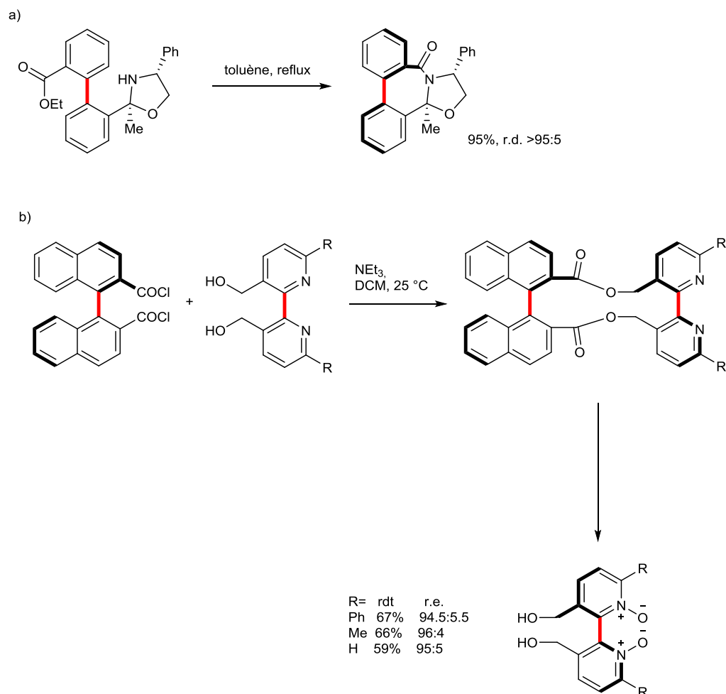
Figure III-66 : formation atroposélective d'un pont
