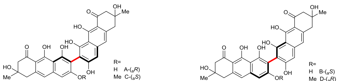
Figure III-71 : isomères des flavomannins A, B, C et D
