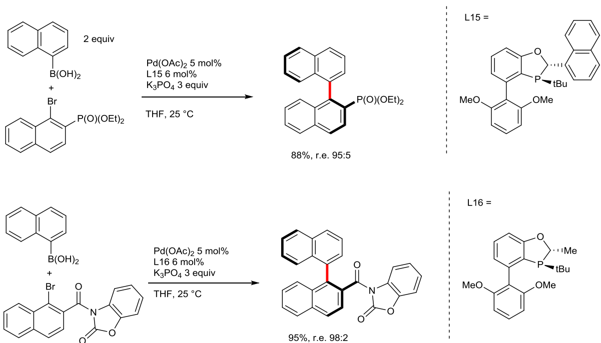
Figure III-36 : couplage atropéantiosélectif avec des ligands monodentates
