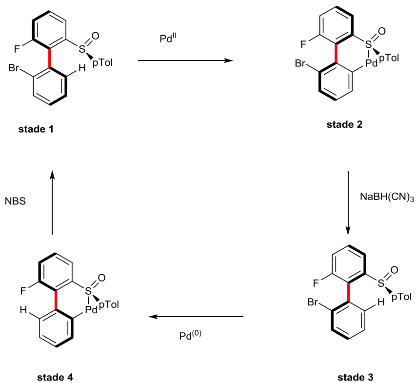
Figure III-83 premier moteur moléculaire fonctionnant sur le cycle red/ox d'un métal de transition
