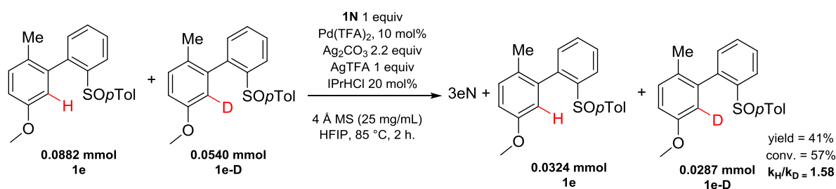
FigureVII-74 : KIE of arylation of 1e into 3eN
