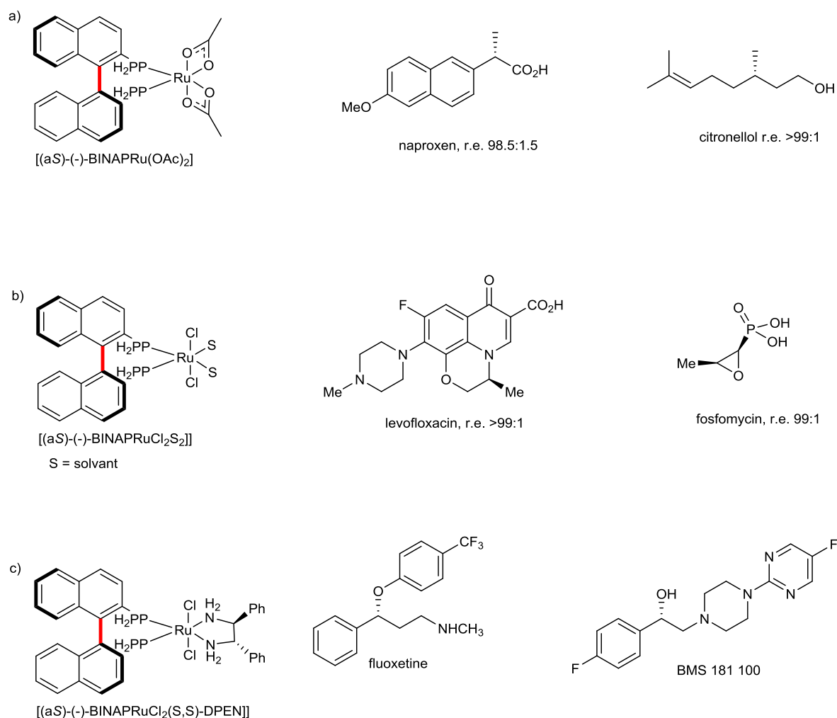
Figure III-76 : complexes BINAP/ruthenium et exemples d'applications industrielles
