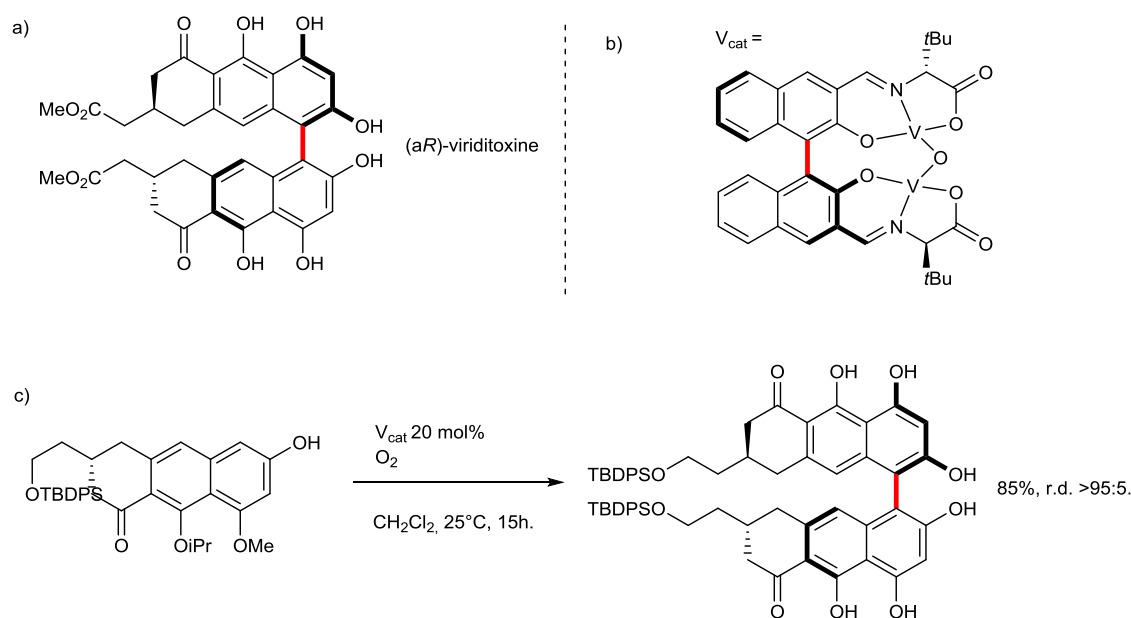
Figure III-72 : construction atroposélective de l'unité biarylique de la viriditoxine
