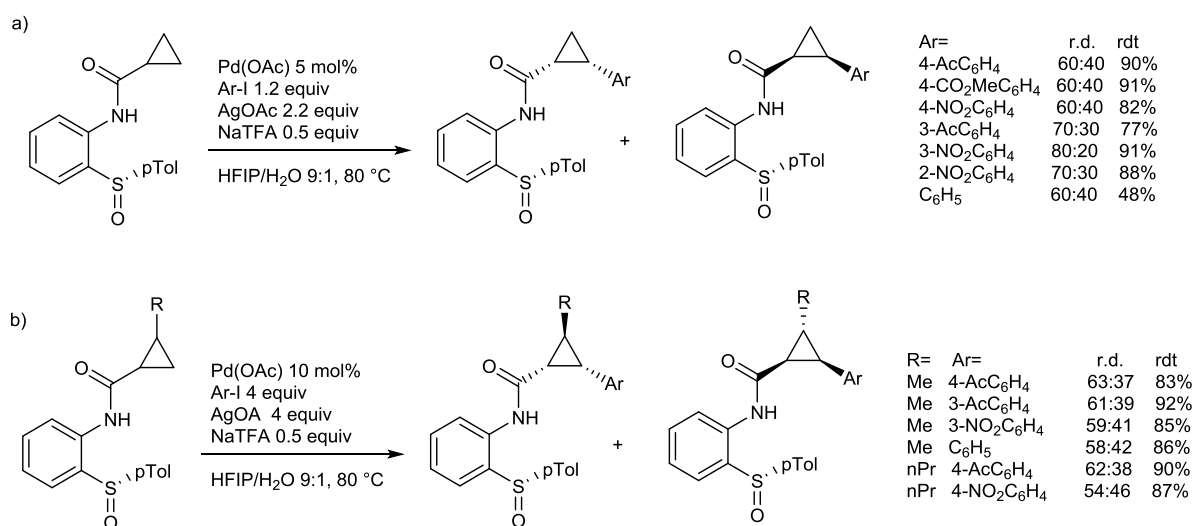
Figure III-96 : arylation diastéréosélective de cyclopropanes
