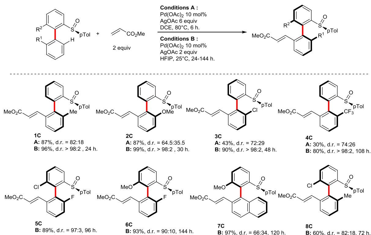
Figure IX-1 : portée de la réaction de Fujiwara-Moritani avec des acrylates
