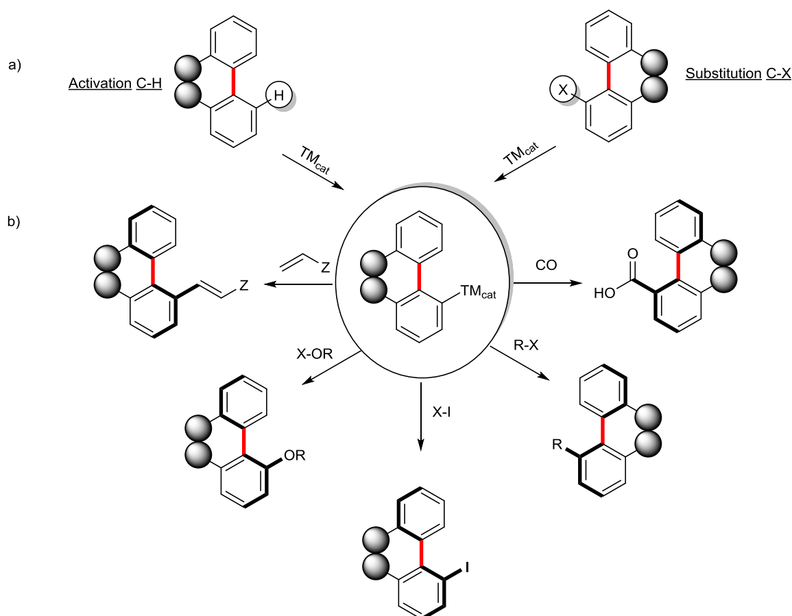
Figure III-45 : possibilités d'insertion d'un nouveau substituant offertes par les métaux de transition
