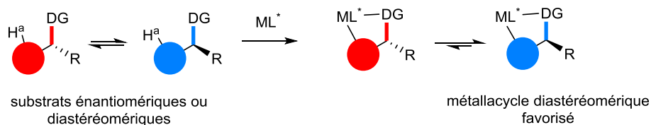
Figure III-10 : cycloméallation diastéréomérique
