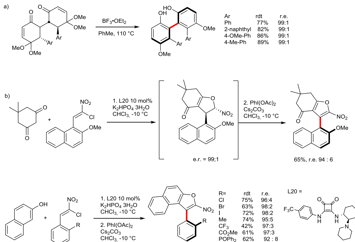
Figure III-43 : transfert de chiralité centrale à axiale.
