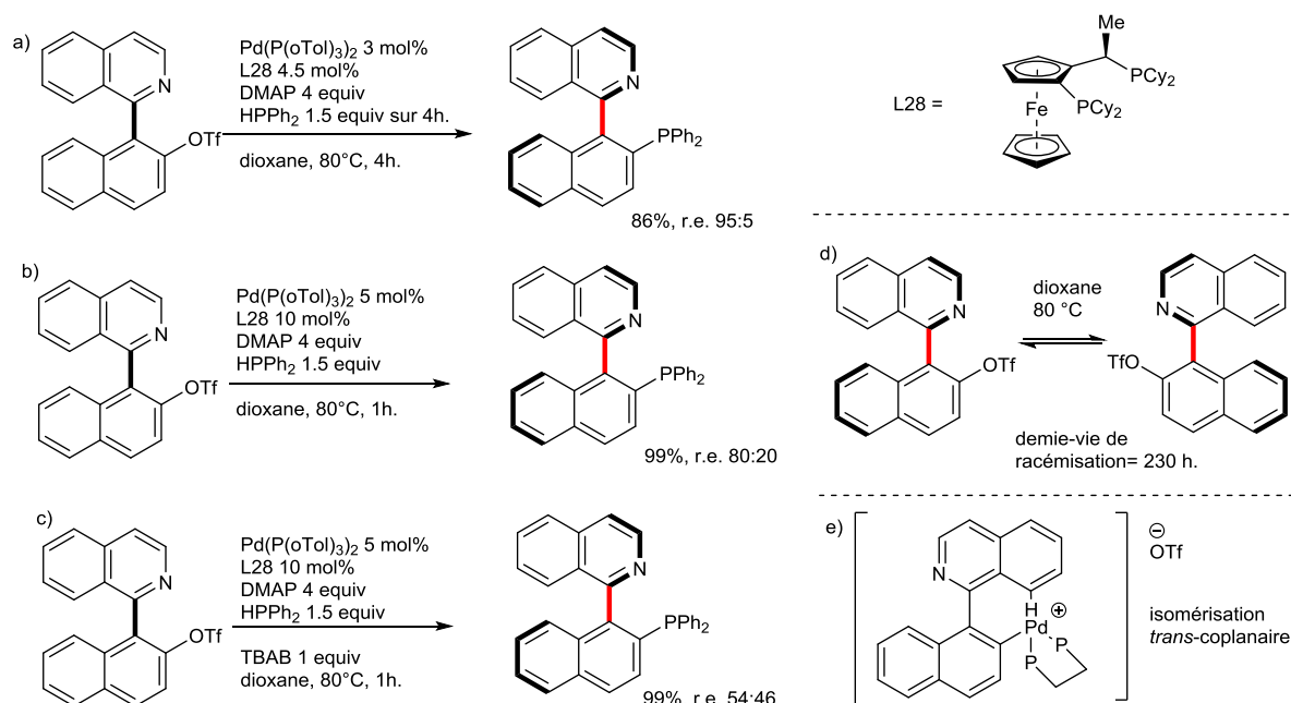
Figure III-57 : phosphination atropoénantiosélective par DKR
