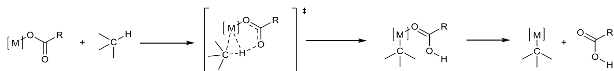
Figure III-5 : mécanisme CMD/AMLA
