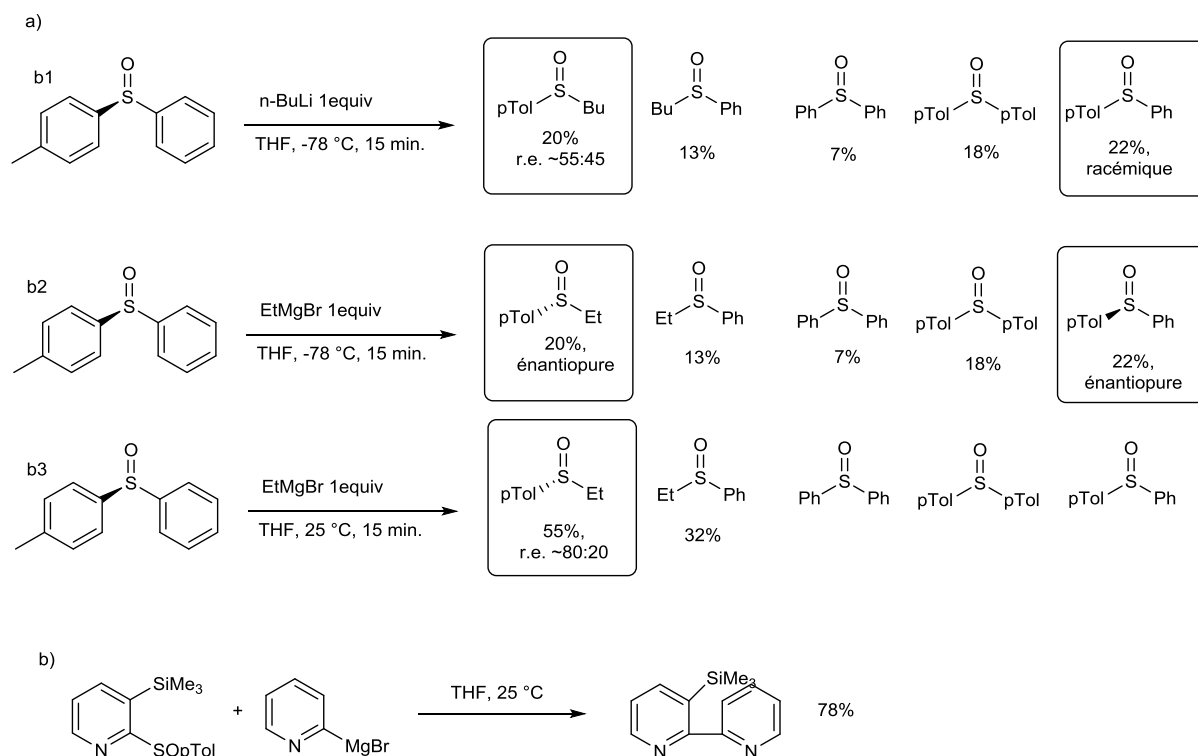
Figure III-109 : comportement des sulfoxydes en présence d'organométalliques
