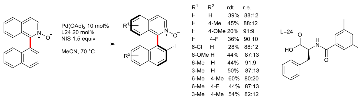
Figure III-49 : iodation atroposélective par KR
