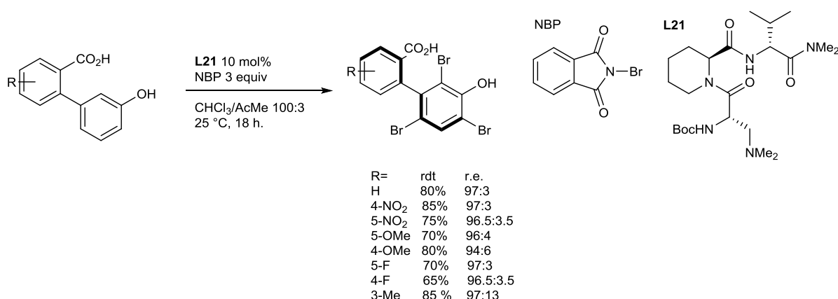
Figure III-47 : bromation atropoénantiosélective
