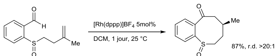
Figure III-90 : hydroacylation diastéréosélective
