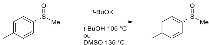
Figure III-106 : stabilité dans des conditions basiques
