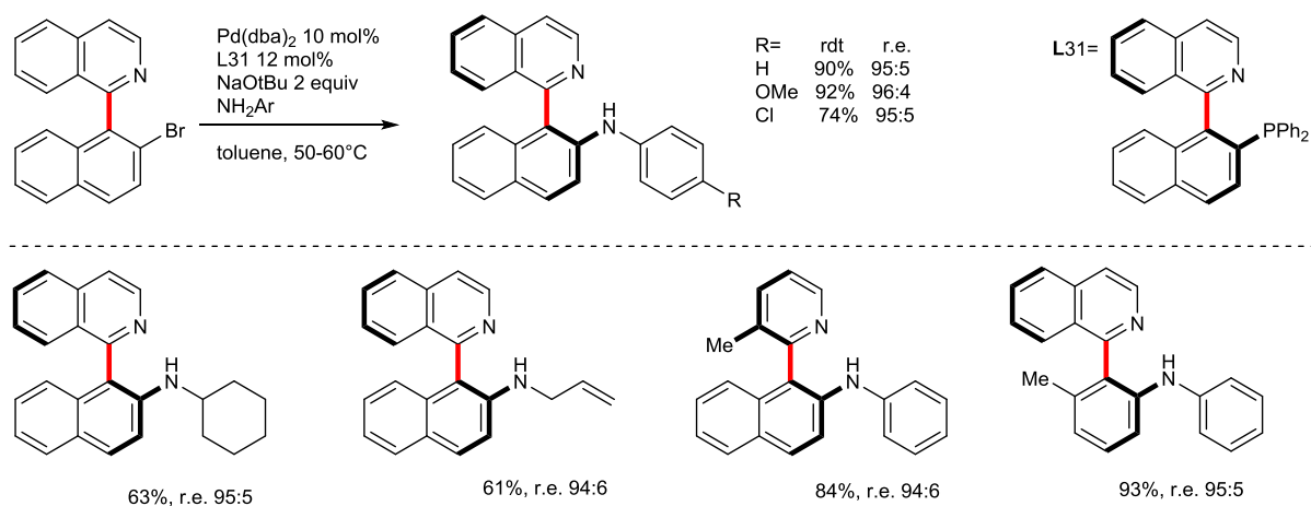
Figure III-60 : amination atropoénantiosélective
