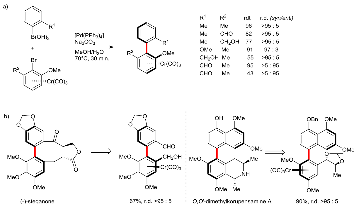
Figure III-34 : couplage atropodiasélectif
