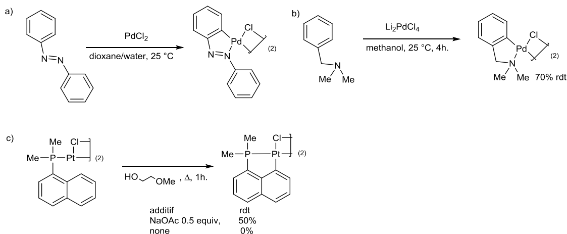
Figure III-6 : premières réactions de cyclométtallation du groupe d10
