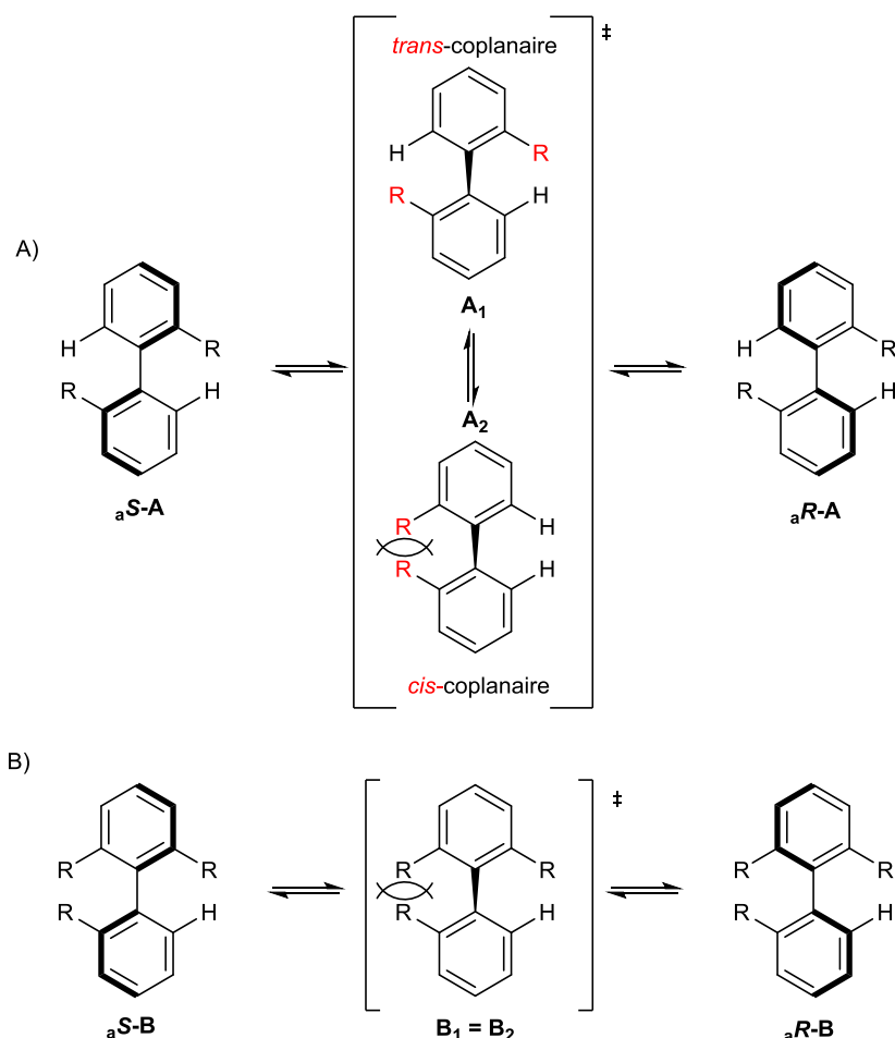
Figure III-18 : mécanisme d'atropisomérisation
