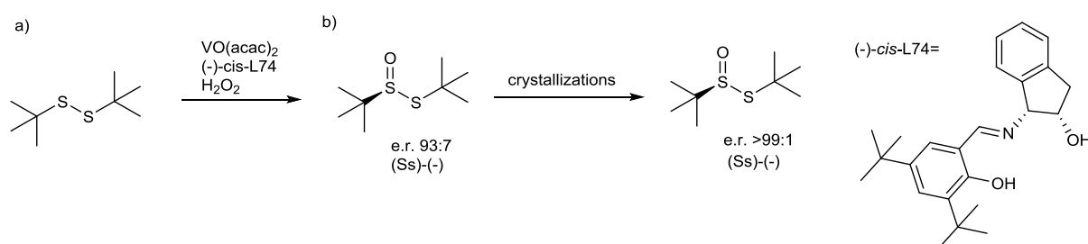
Figure III-101 : méthode d'Ellman
