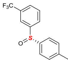
( S )-1-( p -tolylsulfinyl)-3-(trifluoromethyl)benzene Chemical Formula: C 14 H 11 F 3 OS Molecular Weight: 284,2962
