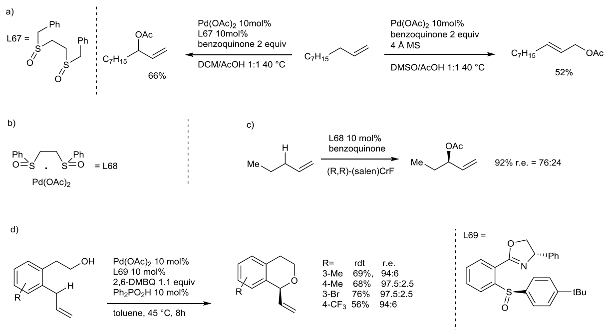
Figure III-88 : activation de liaisons C-H en présence de sulfoxydes
