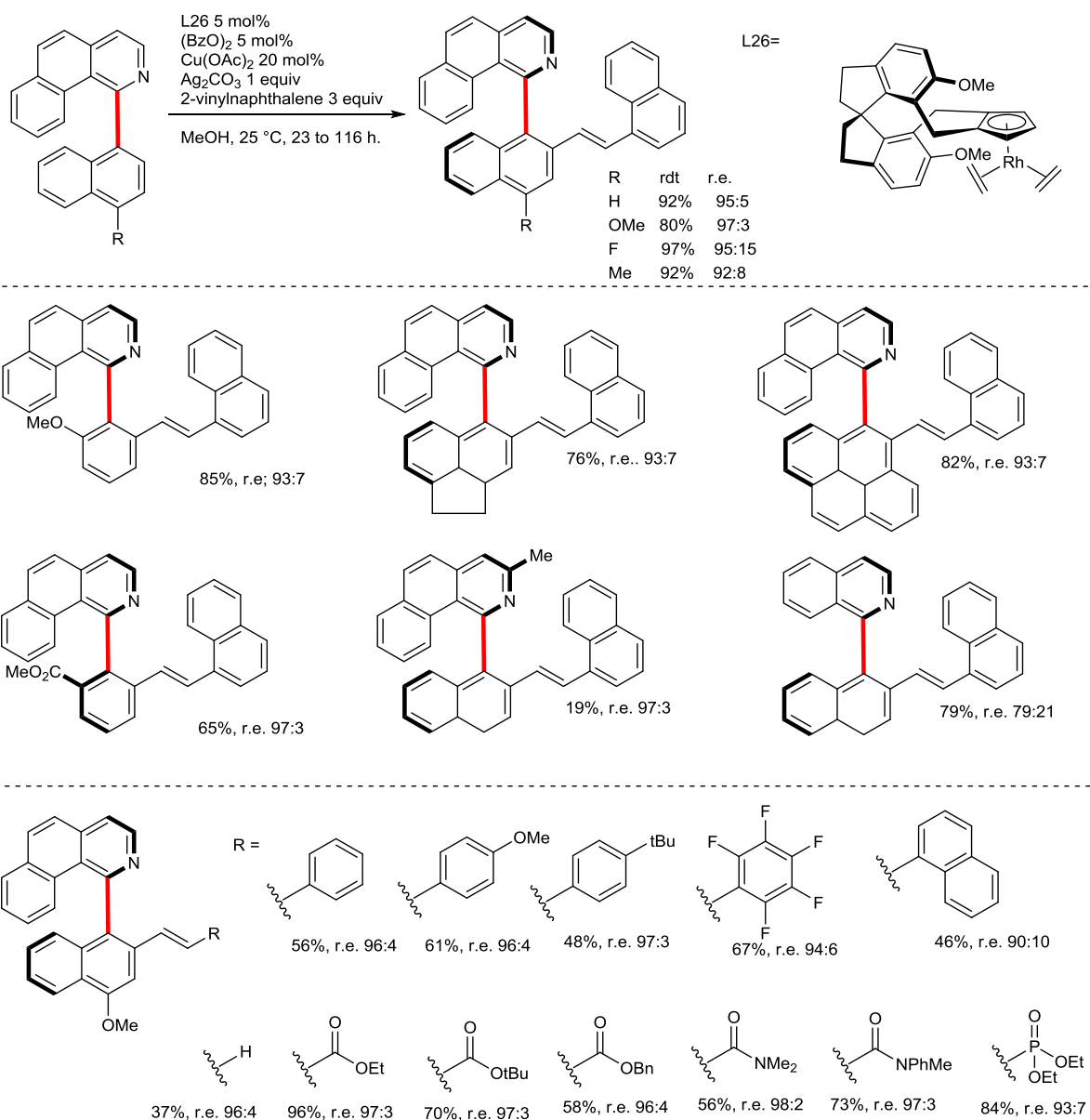
Figure III-52 : oléfination atropoénantiosélective
