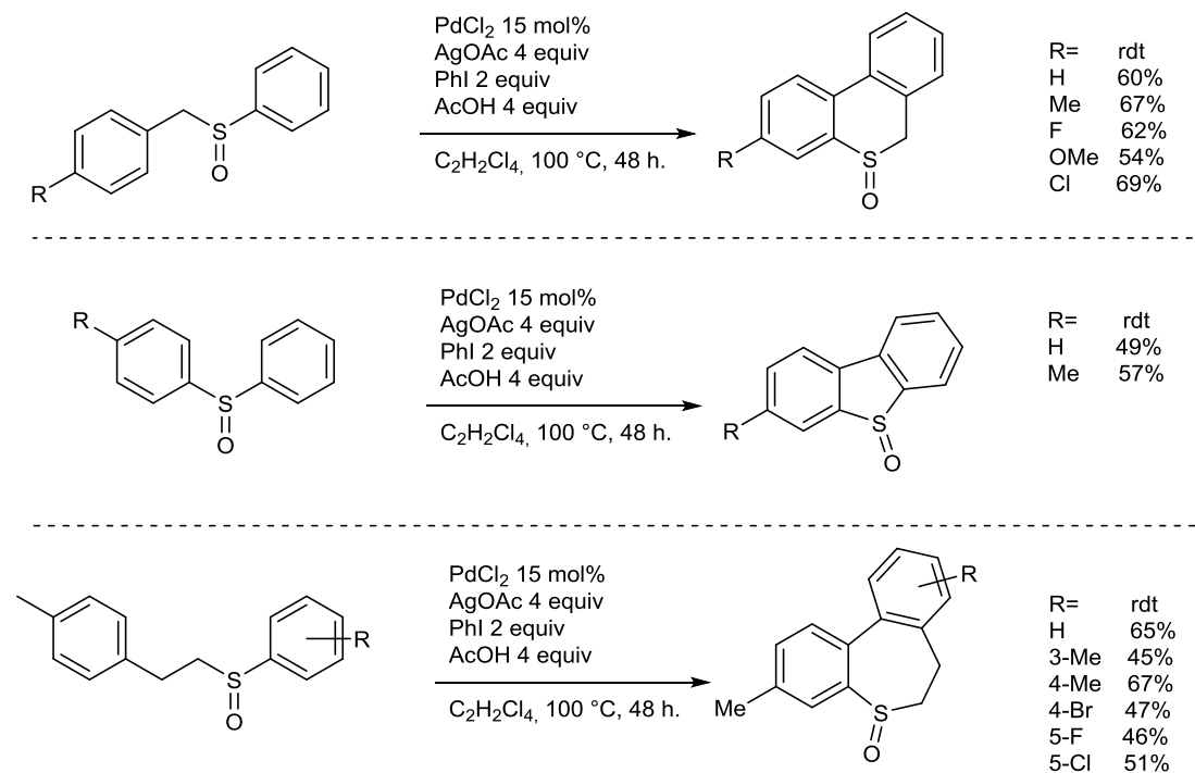
Figure III-92 : double activation de liaison C-H avec un sulfoxyde comme DG
