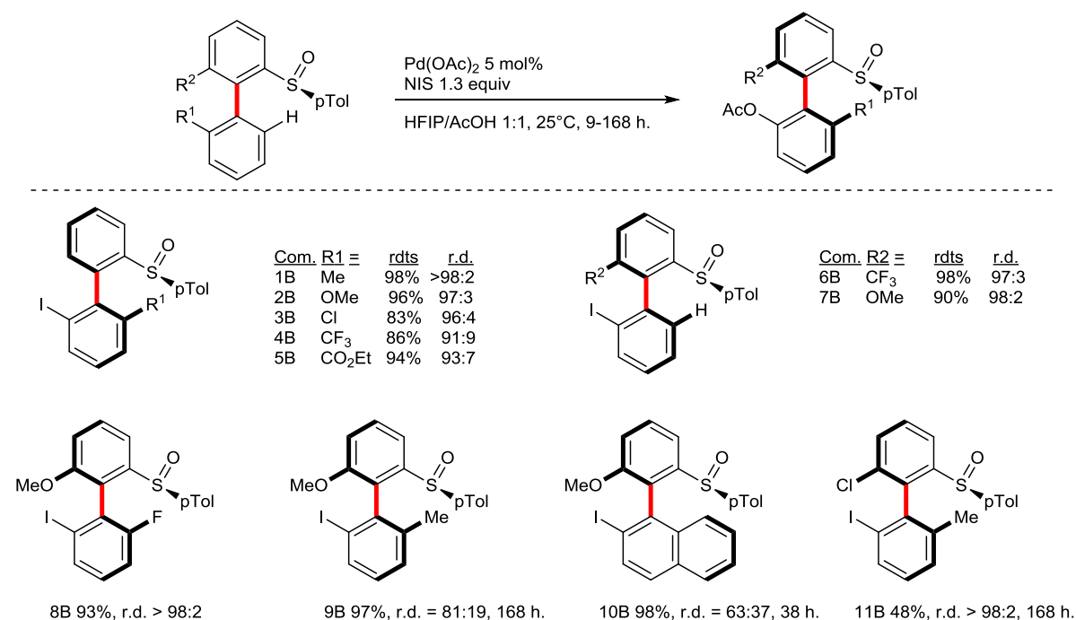
Figure IX-4 : portée de la réaction d'iodation
