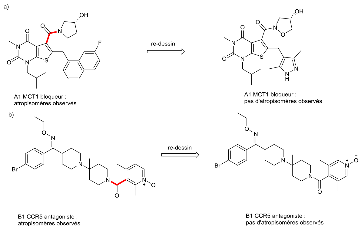
Figure III-68 : stratégie de contournement de l'atropisométrie
