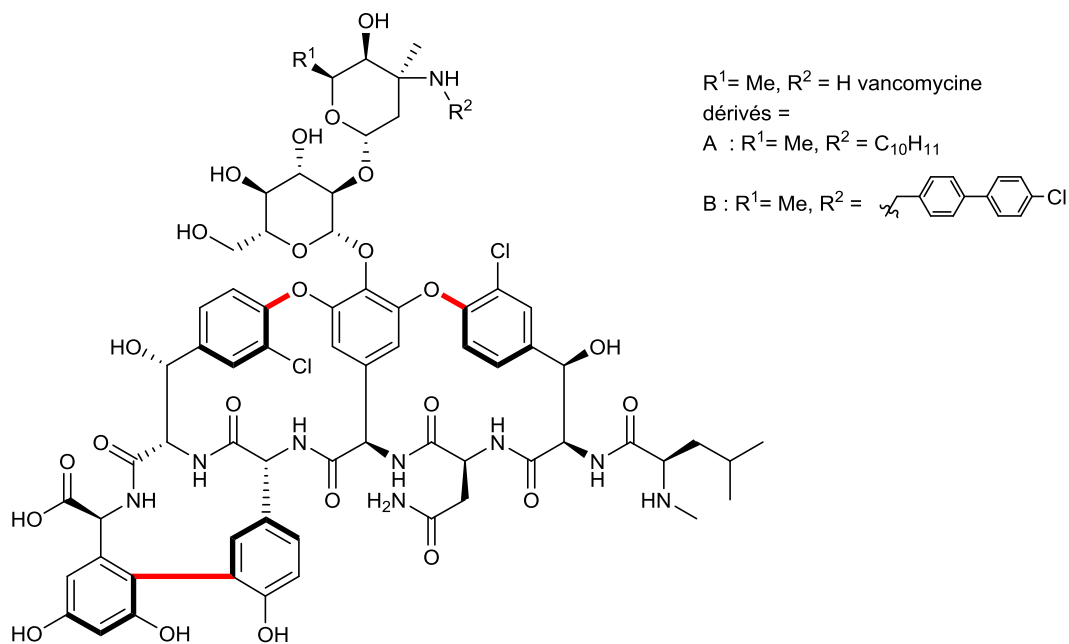
Figure III-70 : vancomycine et dérivés
