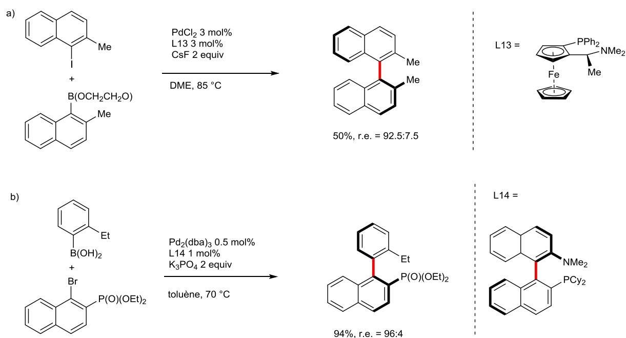
Figure III-35 : couplages atropéantiosélectifs avec des ligands N-P
