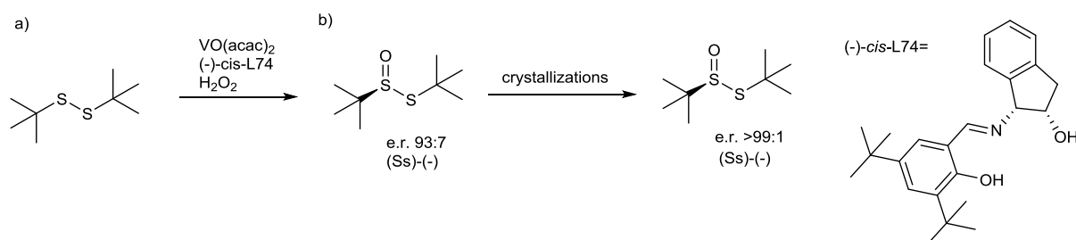
Figure III-101 : méthode d'Ellman
