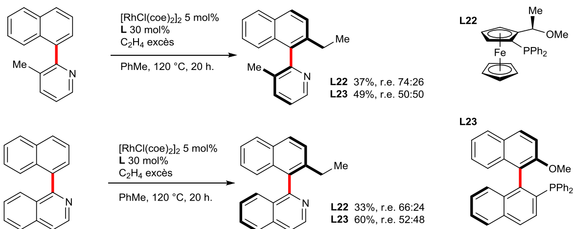
Figure III-48 : premier exemple de fonctionnalisation de liaison C-H atroposélective
