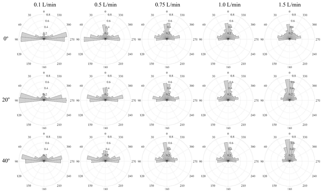
FIGURE 4.16 – Histogrammes (densité de probabilité pdf) en coordonnées polaires représentant l’orientation principale \theta des bulles remontant dans la suspension dense pour différents débits Q (colonnes) et angles d’inclinaison \alpha (lignes). La notation à l’extérieur des cercles indique l’orientation ( 0^\circ = bulles étirées verticalement), les chiffres à l’intérieur des cercles indiquent la valeur de la pdf, ici entre 0 et 0.8 pour l’ensemble des histogrammes.
