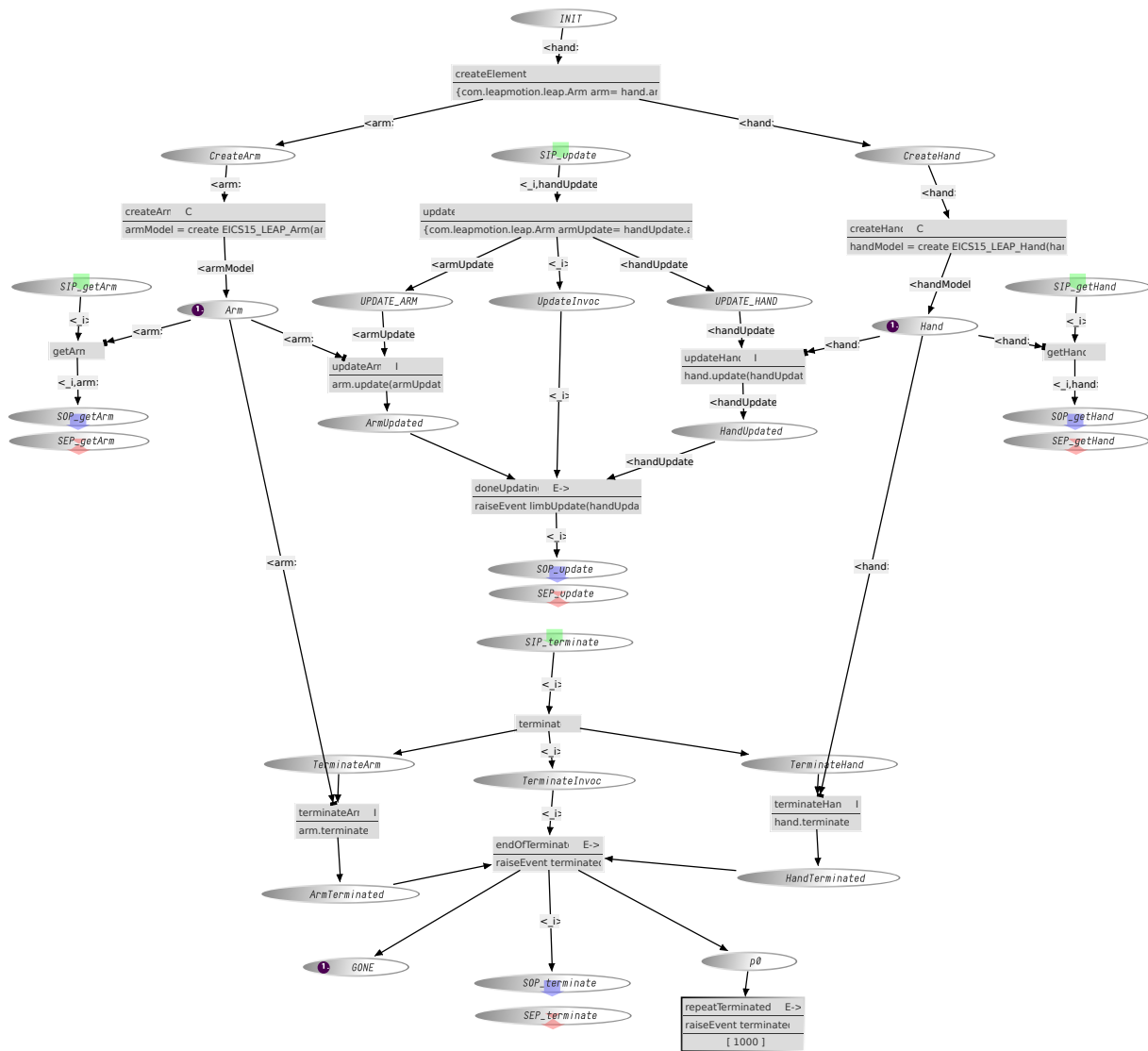
FIGURE 7.7 – Le modèle ICO du membre du Leap motion
