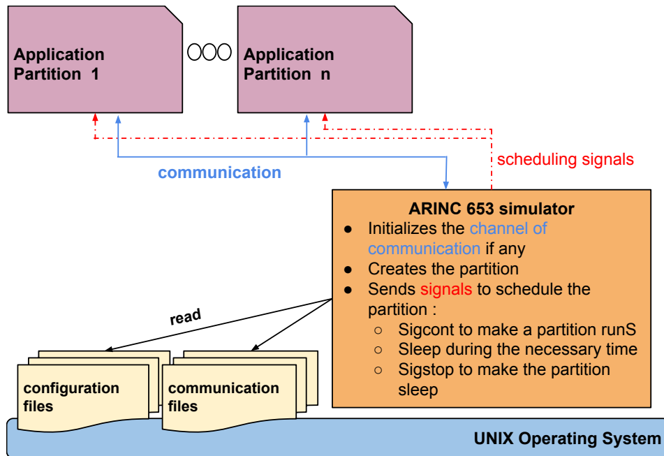
FIGURE 4.5 – Principe de fonctionnement du simulateur ARISSIM [Cronel, ]
