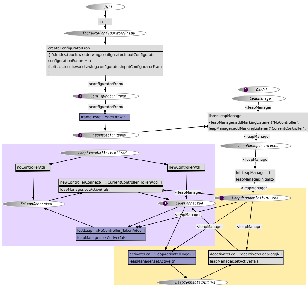
FIGURE 7.12 – Partie du modèle InputConfigurationManager liée à la gestion dynamique du Leap Motion
