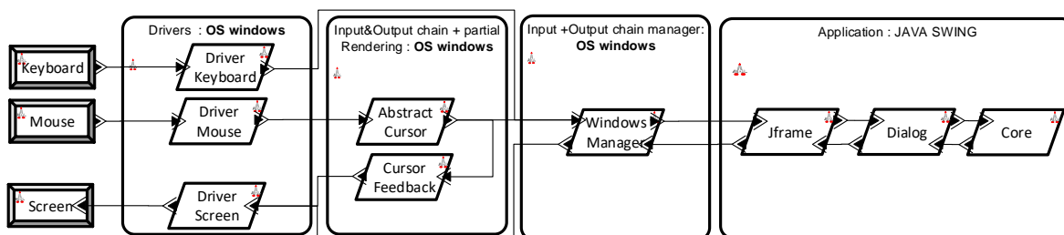
FIGURE 3.6 – Instance de MIODMIT adaptée à l'application des quatre saisons
