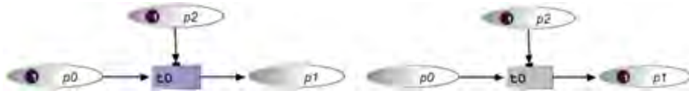
FIGURE 2.9 – État d'un réseau de Petri avant et après le franchissement de transition conditionnée par un arc de test
