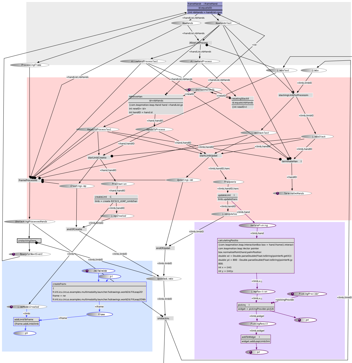
FIGURE 7.6 – Le modèle ICO du gestionnaire de Frame du Leap motion. En bleu les fonctions d'initialisation, en violet les appels aux fonctions de picking
