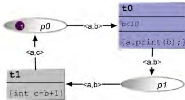
FIGURE 2.13 – Exemple de réseau de Petri à objets
