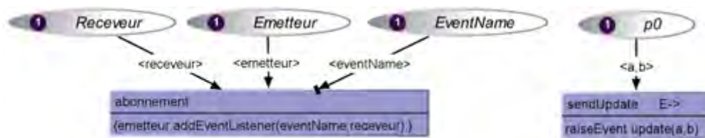
FIGURE 2.16 – Abonnement à un évènement (a) et envoi d'un évènement (b)
