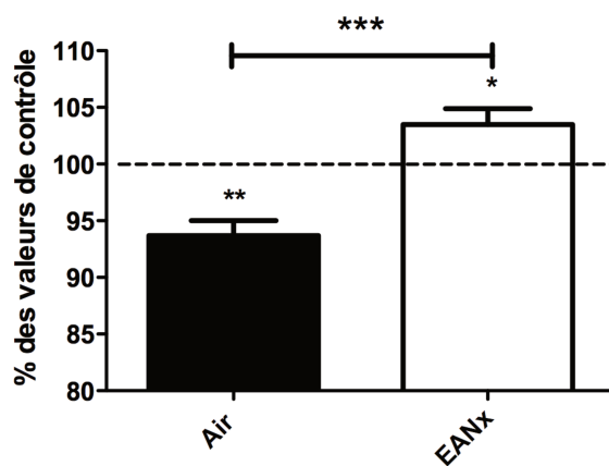
Figure 37. Variation du CFFF après plongée (20-22m/45 min). Les valeurs pré-plongées sont assimilées au 100 %. Chaque sujet est comparé à ses propres valeurs de référence. (**** p < 0,0001 ; *** p < 0,001 ; ** p < 0,01 ; * p < 0,05 ; ns non significatif) (Egypte, n = 219 ) (Les moyennes et déviations standards sont indiquées dans le graphique)
