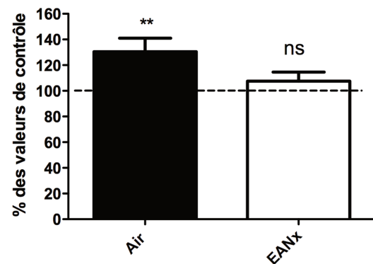
Figure 38. Variation de l'EVA après plongée (20-22m/45 min). Les valeurs pré-plongées sont assimilées au 100 %. Chaque sujet est comparé à ses propres valeurs de référence. (**** p < 0,0001 ; *** p < 0,001 ; ** p < 0,01 ; * p < 0,05 ; ns non significatif) (Egypte, n = 219 ) (Les moyennes et déviations standards sont indiquées dans le graphique)
