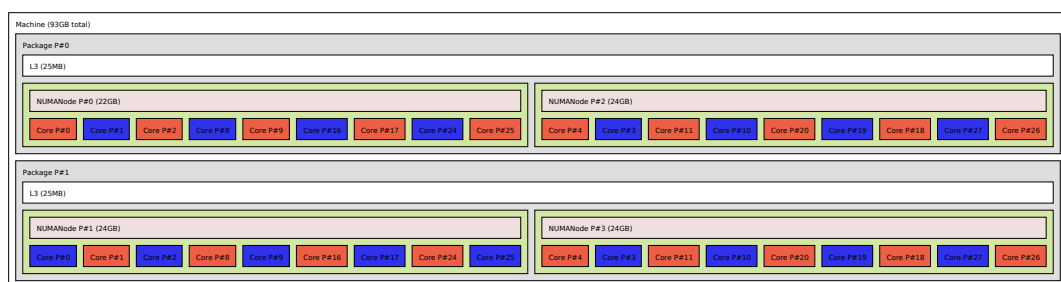
FIGURE 3.3 – Placement des threads qui parcourent des listes chaînées : longues avec chaînage aléatoire en bleu, et courtes avec chaînage contigu en rouge.
