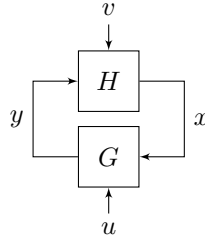
FIGURE C.2 – Interconnexion en boucle (C.80).
