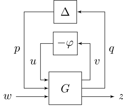
FIGURE C.3 – Représentation du système de Lur'e incertain défini dans (C.171).
