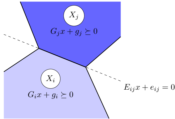
FIGURE C.1 – Partition polytopique de l'espace d'état
