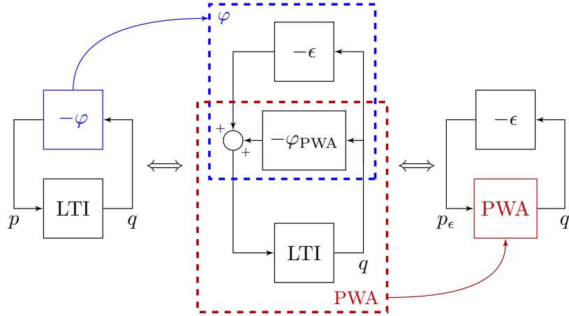
FIGURE C.4 – Diagramme illustrant l’approche proposée dans ce chapitre (les signaux de performance w et z , ainsi que l’incertitude \Delta , sont omis pour plus de clarté).
