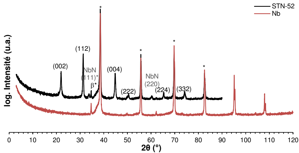
Figure IV-24 : Diagrammes de diffraction des rayons X \theta-2\theta du film STON-52 déposé sur Niobium (noir) et du substrat nu (rouge). Indexation selon SrTaO_2N . (*) pics appartenant au substrat
