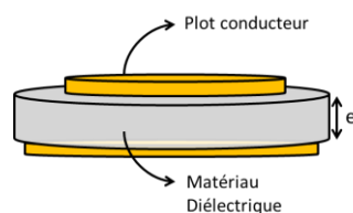
Figure II-17: Dispositif permettant de mesurer la capacité d'une pastille cylindrique
