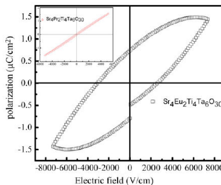
Figure III-44 : Cycles P-E mesurées sur céramiques Sr_4R_2Ti_4Ta_6O_{30} ( R = Pr, Eu ) 18
