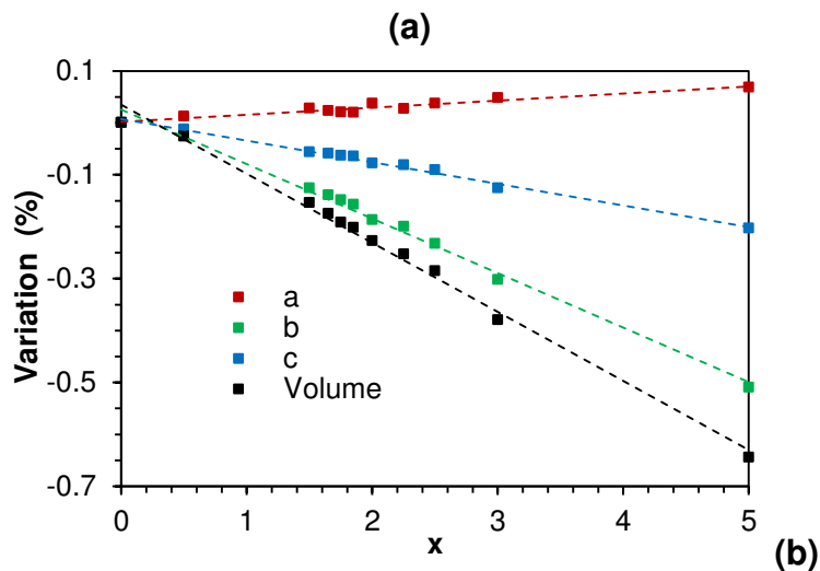
Figure II-3 : Evolution en fonction de la composition ( x ) des paramètres de maille a , b , c et du volume de maille ( V ) des poudres (\text{Sr}_2\text{Ta}_2\text{O}_7)_{100-x}(\text{La}_2\text{Ti}_2\text{O}_7)_x synthétisées par voie solide : (a) variations absolues et (b) variations relatives. L'incertitude sur les valeurs est inférieure à la hauteur du marqueur utilisé dans chaque graphe
