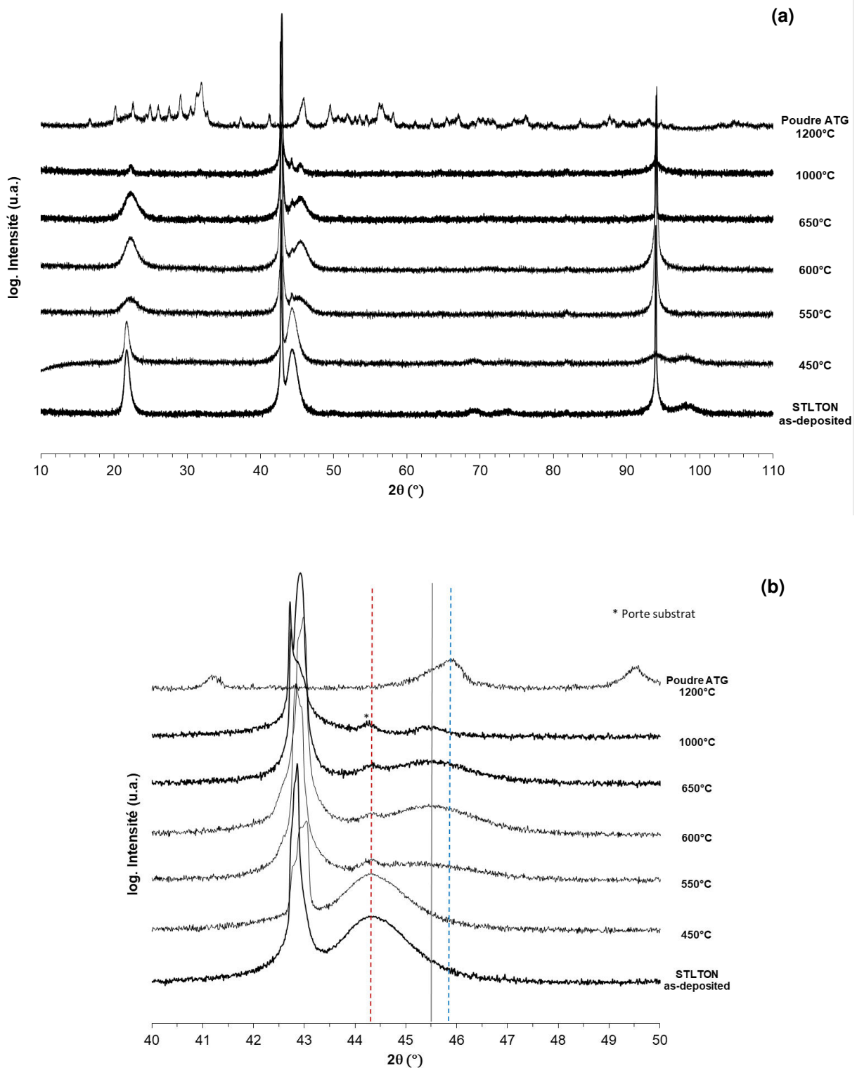
Figure IV-11: (a) Vue d'ensemble et (b) détail des diagrammes de diffraction des rayons X \theta-2\theta des couches STLTON recuites sous air à différentes températures. Nous avons également fait figurer le diagramme d'une couche oxyde STLTO as-deposited et d'une poudre SrTaO 2 N recuite en ATG à 1200°C sous air. Les droites verticales orange et bleues sont des repères visuels des positions angulaires des pics de diffraction des couches STLTON et STLTO as-deposited. La verticale en pointillés gris localise le pic de diffraction des échantillons recuits.
