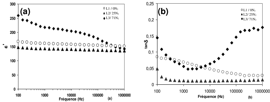
Figure I-21 : Evolution en fonction de la fréquence (a) de la permittivité \epsilon' et (b) des tangentes de pertes \tan\delta de couches \text{LaTiO}_x\text{Ny} déposées sur \text{Nb-SrTiO}_3 (001) à partir d'une cible \text{LaTiO}_2\text{N}^{140}
