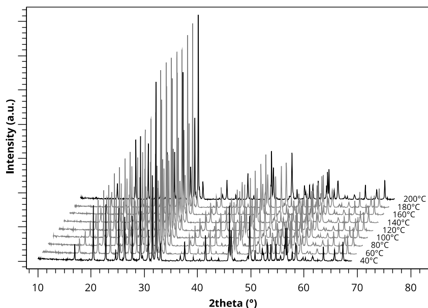
Figure II-45 : Diffractogrammes DRX \theta-2\theta de la poudre (\text{Sr}_2\text{Ta}_2\text{O}_7)_{100-x}(\text{La}_2\text{Ti}_2\text{O}_7)_x avec x = 3 en fonction de la température
