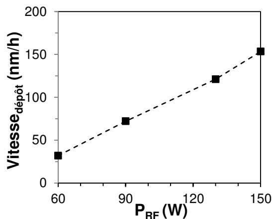
Figure III-6 : Evolution de la vitesse de dépôt en fonction de la puissance radiofréquence des films minces STLTO déposés par pulvérisation cathodique avec T S = 800°C ; %O 2 = 19 % et P T = 45 mTorr
