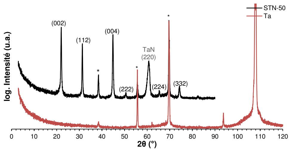
Figure IV-25 : Diagrammes de diffraction des rayons X \theta-2\theta du film STON-50 déposé sur Tantalum (noir) et du substrat nu (rouge). Indexation selon SrTaO_2N et selon TaN (JCPDS 49-1283). (*) pics appartenant au substrat
