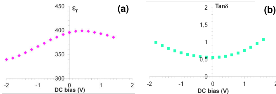
Figure I-22 : Evolution en fonction de la tension continue appliquée (a) de la permittivité \epsilon' et (b) des tangentes de pertes \tan\delta de la bicouche LTO-25 déposée sur \text{SrTiO}_3:\text{Nb} avec la cible \text{La}_2\text{Ti}_2\text{O}_7^{138}
