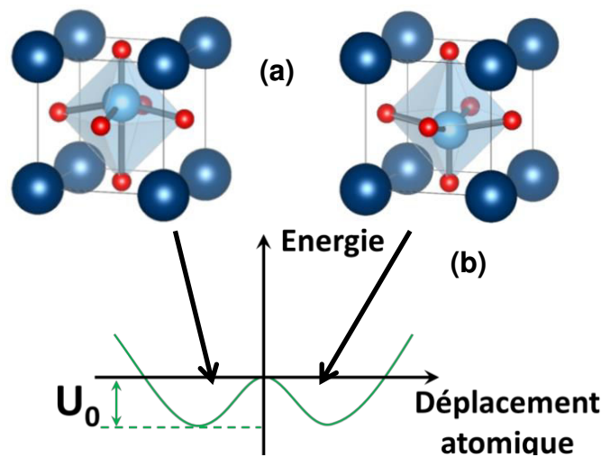
Figure I-6 : (a) Schéma d'une maille perovskite ferroélectrique dans deux états de polarisation, (b) barrière de potentiel entre les deux états. « Adaptée de la Ref 60 »
