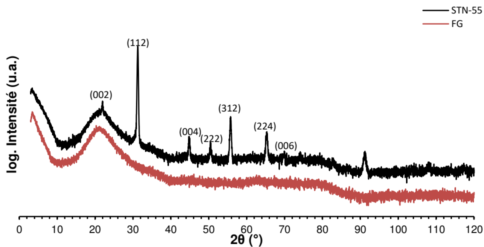
Figure IV-28 : Diagrammes de diffraction des rayons X \theta-2\theta du film STON-55 déposé sur Fused Glass (noir) et du substrat nu (rouge). Indexation selon SrTaO 2 N
