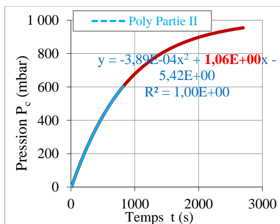
Figure 2.14. Remontée de la pression P_c(t) (sur une éprouvette de notre étude)
