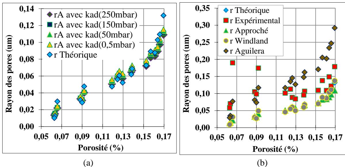
Figure A.7. Rayons calculés pour différentes k_{ad} (a) et rayons de différents modèles (b)
