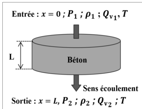
Figure 2.6. Conditions aux limites pour écoulement d'un gaz à travers un échantillon en béton. Le type de pression (dépression et surpression) et le type de régimes de débit (permanent ou non-permanent) sont définis dans le Tableau 2.3 pour les différentes techniques de mesure utilisées dans ce travail.
