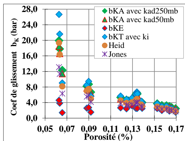
Figure A.8. Coefficient de glissement b_K théorique, expérimentaux et estimés
