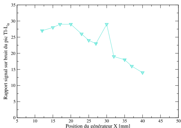
FIGURE 4.44 – Rapport signal sur bruit du pic TI- L_{\alpha} avec un détecteur positionné à 3 mm en fonction de la position du générateur X.
