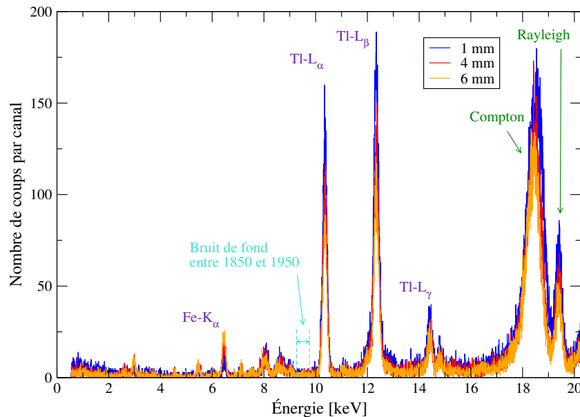
FIGURE 4.18 – Spectre X d'une solution de thallium à 5 g/L acquis durant 300 secondes, pour différentes distances entre l'échantillon et le détecteur X.
