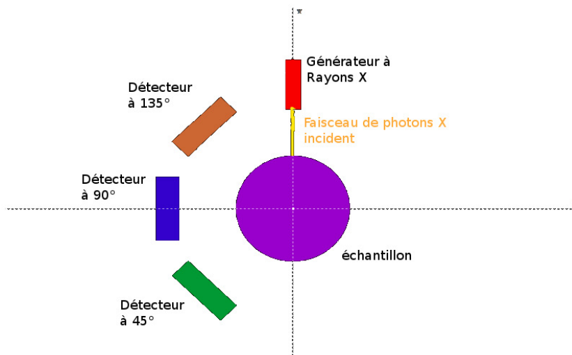
FIGURE 3.10 – Mesure du rayonnement de fluorescence X et de diffusion aux angles de 45°, 90° et 135°.
