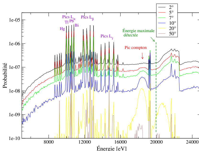
FIGURE 3.34 – Spectres XRF d'une solution de mercure à 10 g/L, de thallium à 10 g/L, de plomb à 10 g/L et de bismuth à 10 g/L dans une matrice HNO 3 à 10% en fonction de l'orientation angulaire de la cible secondaire.
