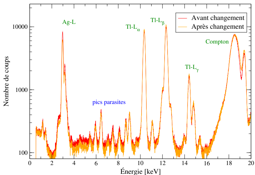
FIGURE 4.48 – Présence maintenue des pics parasites après le changement du générateur X.
