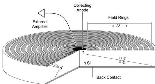
FIGURE 1.20 – Détecteur SDD ( silicon drift detector ) [31].
