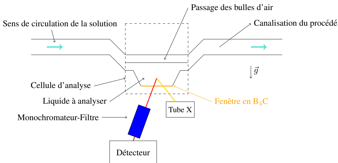
FIGURE 1.36 – Schéma d'une cellule d'analyse en ligne réalisée par le CEA Saclay [70, 71].
