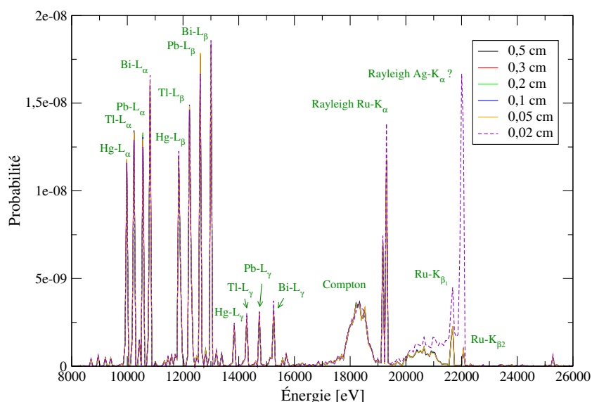
FIGURE 3.37 – Spectres XRF en fonction de l'épaisseur de la cible en ruthénium orientée à 20^\circ et pour un récipient cylindrique en Téflon de 0,1 mm d'épaisseur.
