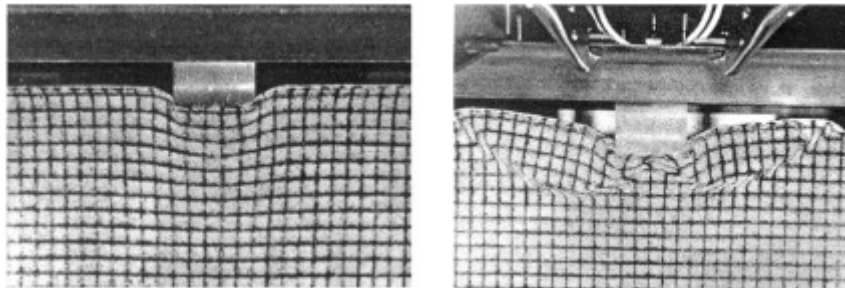
Figure 2.10 : Mécanisme de rupture pour un chargement dynamique (à gauche) et statique (à droite) (d'après Selig et McKee (1961) )
