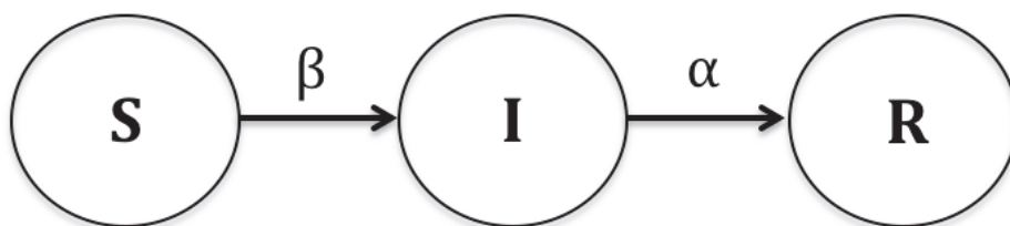
Figure 2. Modèle SIR de Kermack et McKendrick (55). S : susceptible, I : infectieux, R : recovered, \beta : probabilité d'infection par contact, \alpha : taux de guérison
