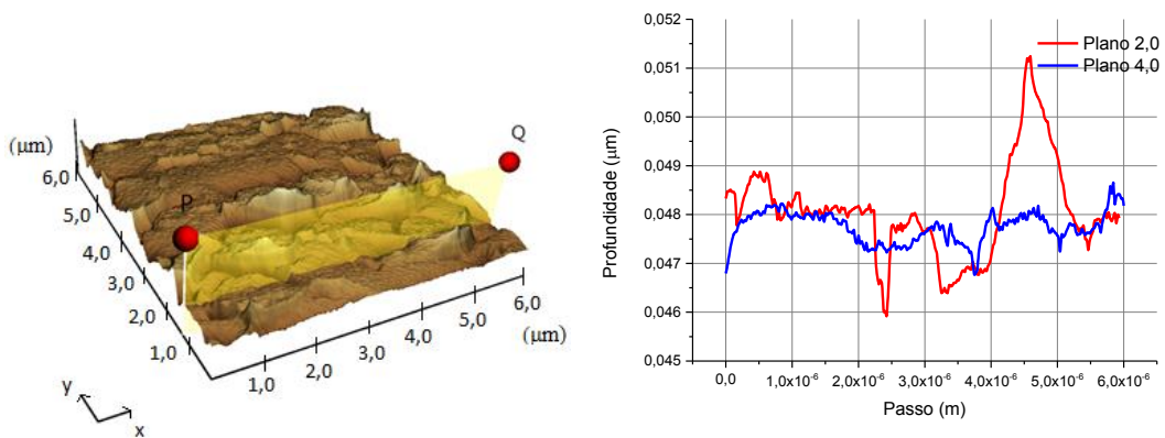
Figura 5.11: Imagem AFM da superfície da amostra Al_002 em perfil. Ao lado, são mostrados os perfis ao longo da direção y.
