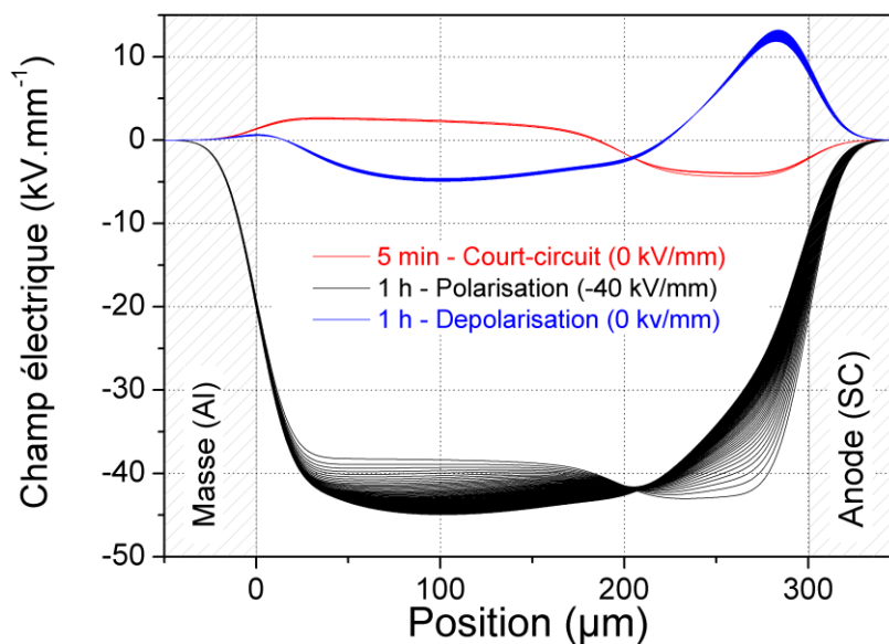
Figure 4.25 : Champ électrique associé aux densités de charges d'espace simulées en Figure 4.24b, pour un PEbd vierge polarisé pendant une heure sous un champ électrique continu de - 40 \text{kV}/\text{mm} , suivi d'une heure de dépolarisation. Paramètre du Tableau 4.5.
