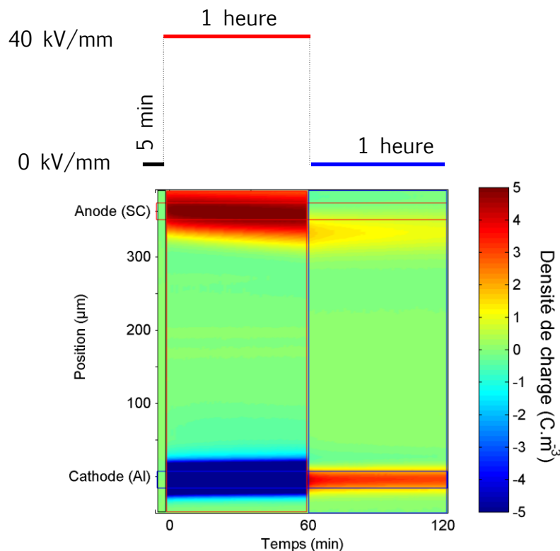
Figure 2.11 : Protocole et type de résultats obtenus à partir de mesures PEA ex-situ sous polarisation DC. Cas d'un film de PEbd vierge (non-irradié) de 350 \mu\text{m} d'épaisseur.
