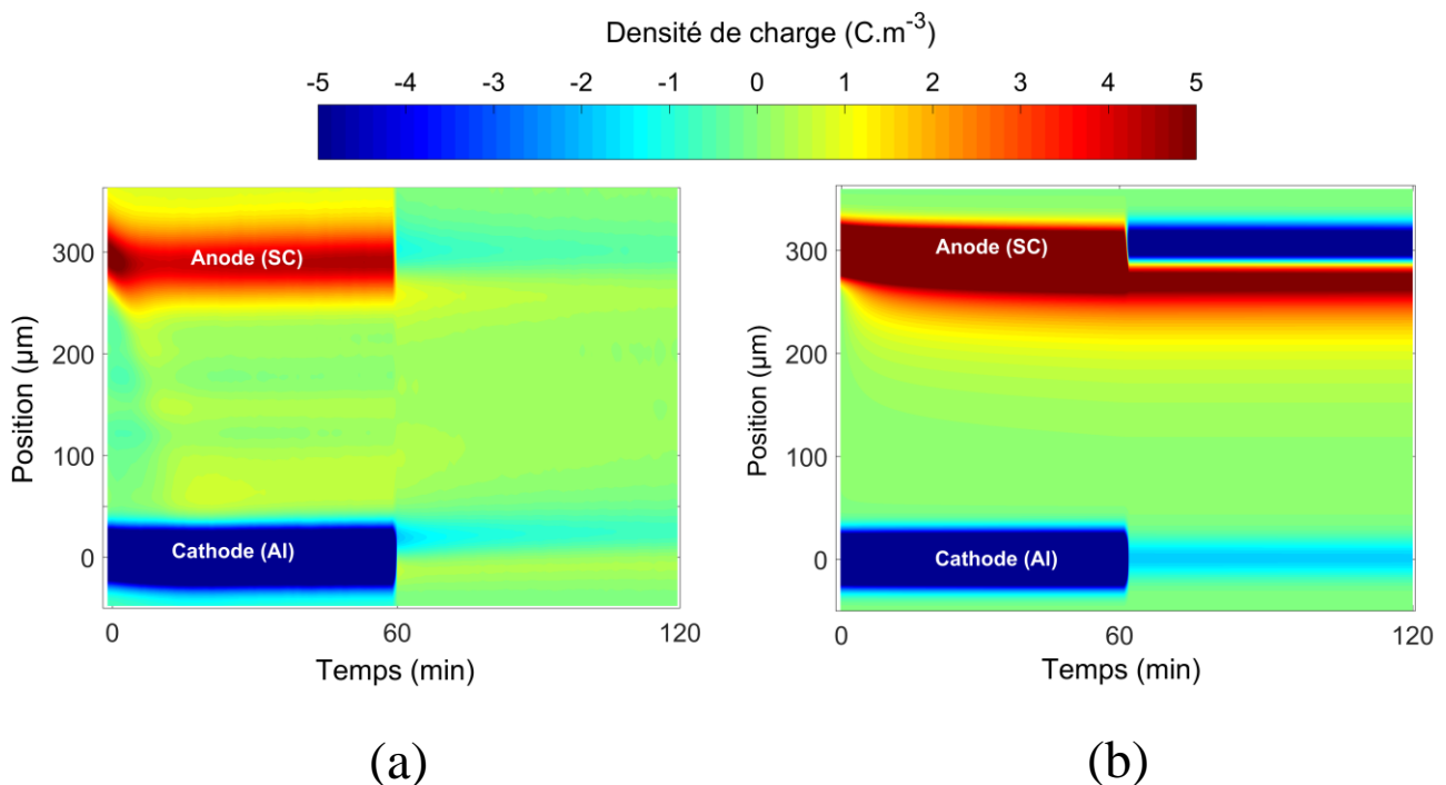
Figure 4.21 : Densités de charges (a) mesurées et (b) simulées, en fonction de la position au sein d'un film de PEbd de 300\ \mu\text{m} d'épaisseur. Polarisation pendant une heure sous un champ électrique continu de -40 kV/mm suivi d'une heure de dépolarisation. Paramètre du Tableau 4.5.
