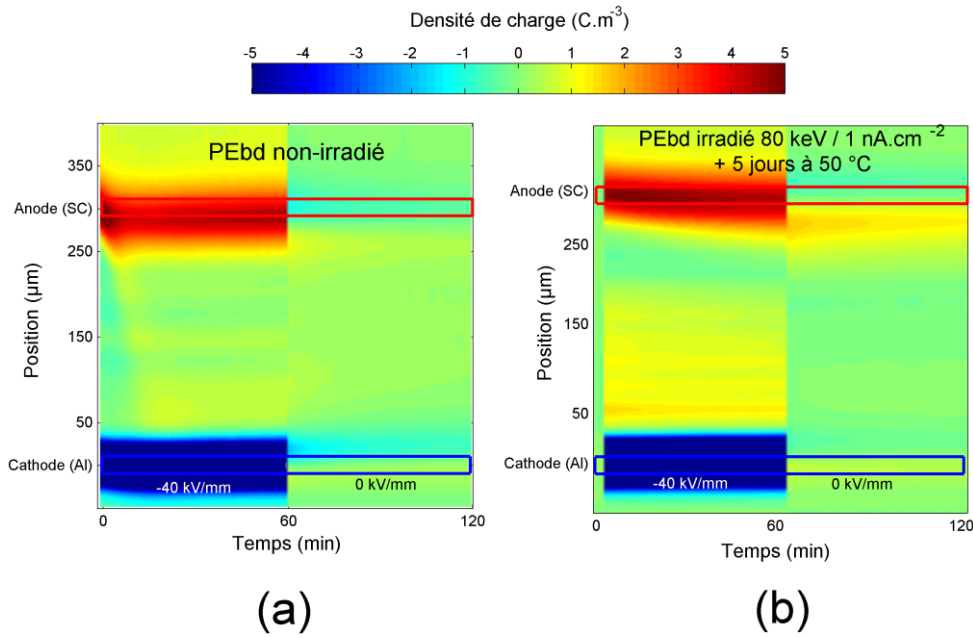
Figure 3.21 : Cartographies de charge d'espace PEA sur un PEbd de 300 μm d'épaisseur. (a) PEbd non-irradié (référence) ; (b) PEbd irradié à 80 keV et 1 nA/cm 2 pendant 10 minutes et polarisé une première fois sous un champ électrique de -40 kV/mm puis maintenu sous étuve à 50 °C pendant 5 jours avant nouvelle mesure PEA sous polarisation -40 kV/mm.
