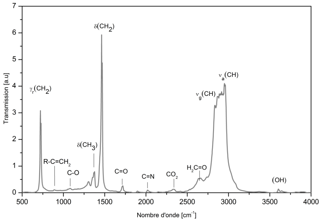
Figure 2.17 : Spectre Infra-Rouge (FTIR) mesuré sur un film PEbd vierge (non-irradié) de 200 µm d'épaisseur. Mesure réalisée en transmission.
