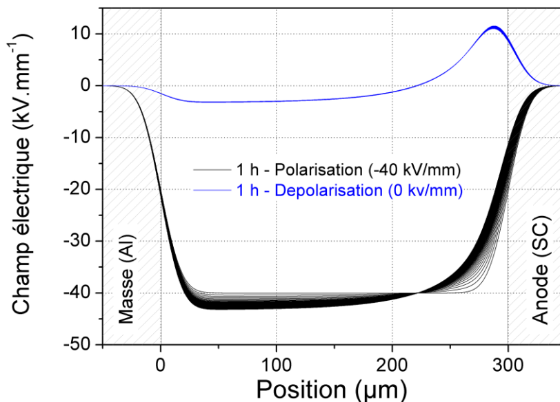
Figure 4.22 : Champ électrique associé aux densités de charges d'espace simulées en Figure 4.21b. Pour un PEbd vierge polarisé pendant une heure sous un champ électrique continu de - 40 kV/mm suivi d'une heure de dépolarisation. Paramètres du Tableau 4.5.
