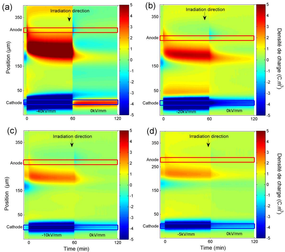
Figure 3.12 : Cartographie de densités de charges pour différentes épaisseurs de PEbd irradié puis soumis à différentes amplitudes de champ électrique : (a) -40 kV/mm, (b) -20 kV/mm, (c) -10 kV/mm, (d) -5 kV/mm. Mêmes conditions de mesures qu'en Figure 3.8.
