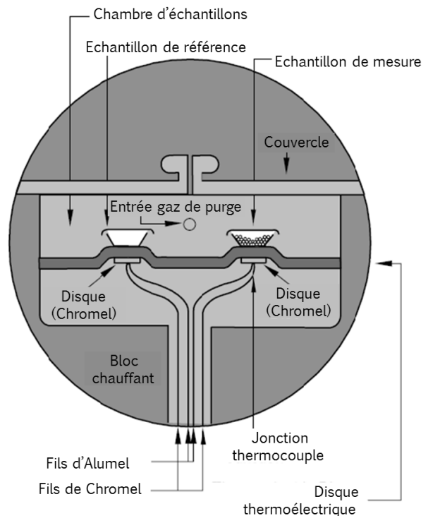
Figure 2.18 : Schéma du dispositif de mesure DSC.
