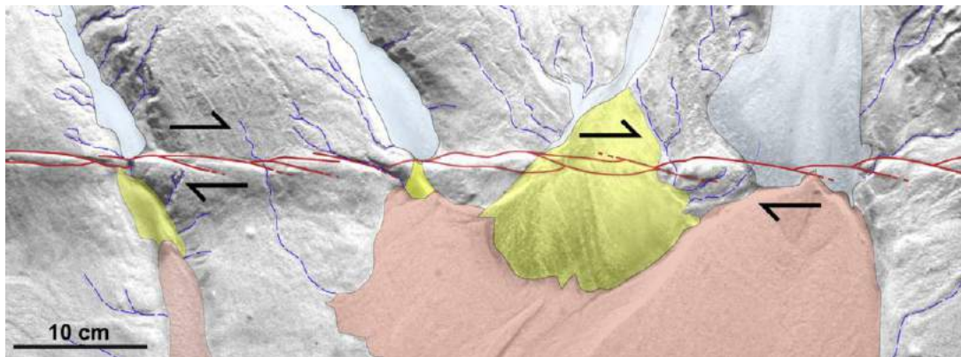
FIGURE II.25 – Vue de la dynamique de la topographie liée à une tectonique décrochante. Modélisation réalisée avec le dispositif de Montpellier (Graveleau et al. , 2015).
