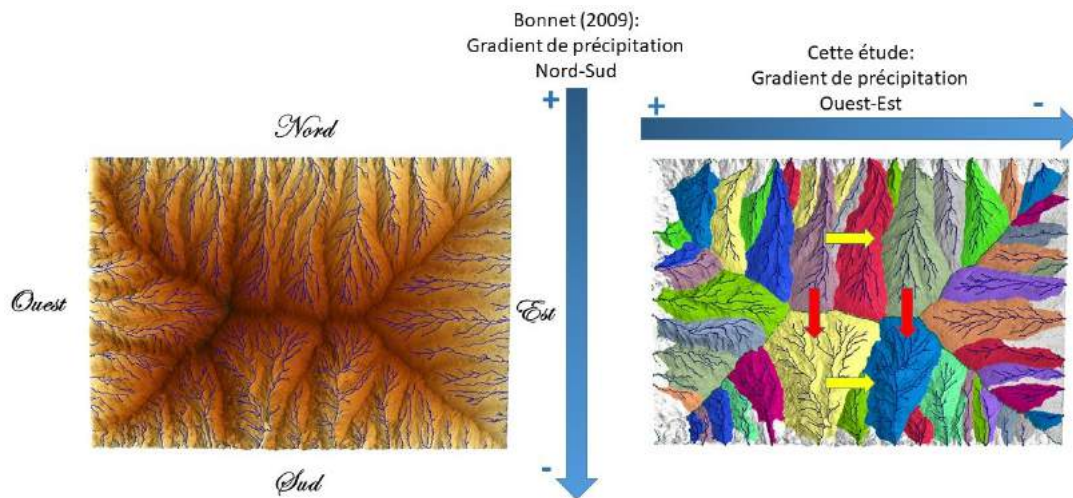
FIGURE VI.3 – Gradient de précipitation Nord-Sud étudié par Bonnet (2009), perpendiculaire à la principale ligne de partage des eaux, ce qui induit son déplacement (flèches rouges). Dans ce chapitre nous présentons les résultats d'expériences réalisées selon un gradient Ouest-Est dans le but de documenter d'éventuels déplacements des lignes de crête et des réseaux de rivières (flèches jaunes).
