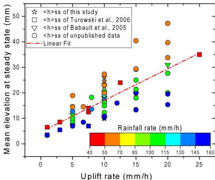
FIGURE IV.15 – Synthèse des données de hauteurs moyennes d'équilibre en fonction des taux d'Uplift. Les données représentées en étoiles sont issues de notre étude sur la réponse érosive des reliefs (voir chapitre V).
