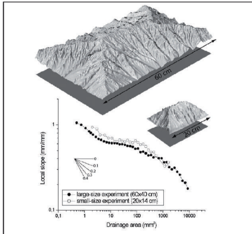
FIGURE II.15 – Étude comparative entre deux topographies expérimentales issues de dispositifs de modélisations de tailles différentes (Bonnet et Crave, 2006).
