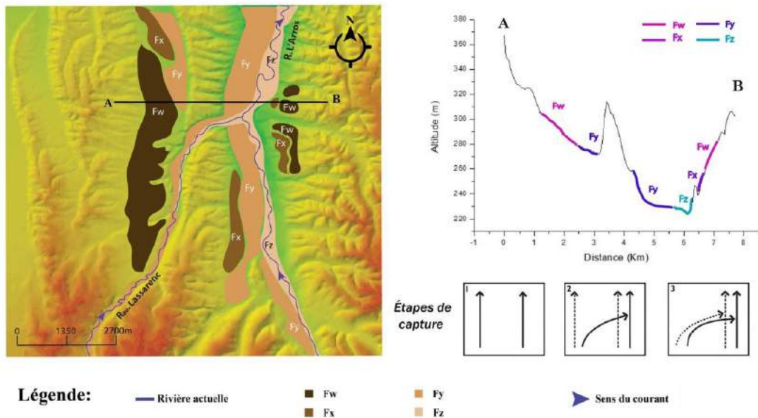
FIGURE VI.12 – Exemple de capture observable dans la zone d'étude (capture du Lers par L'Arros). La cartographie des terrasses est issue de la carte au 1/50 000 de Tarbes. figure de Al Reda, 2015, Evolution et réorganisation des réseaux hydrographiques du piedmont Nord-Pyrénéen. Mémoire de Master 2, Univ Paul Sabatier).
