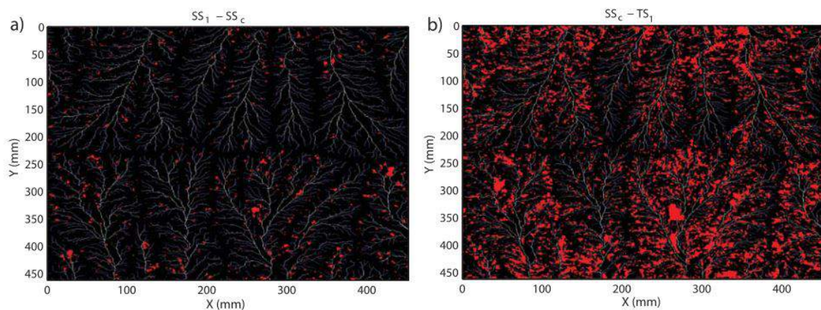
FIGURE II.7 – Distribution spatiale de l'érosion a la surface de la topographie (a) Différence entre deux topographie a l'équilibre et (b) Différence entre topographie transitoire et topographie d'équilibre (Singh et al. , 2015).
