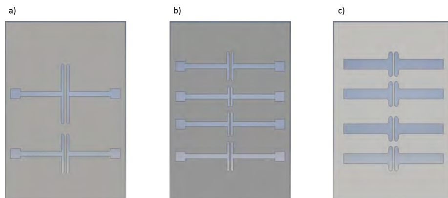
FIGURE 3.17 – Masques en inox de 300 \text{ }\mu\text{m} d'épaisseur pour réaliser les électrodes source et drain du transistor avec une a) longueur de canal de 500 et 600 \text{ }\mu\text{m} , b) longueur variant de 100 à 400 \text{ }\mu\text{m} , c) longueur de canal fixe.
