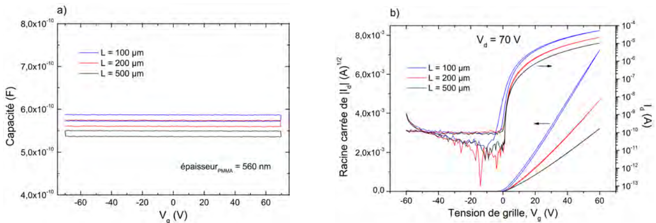
FIGURE 4.4 – a) Capacité en fonction de la tension de grille d'une couche de PMMA de 560\ \text{nm} pour une longueur de canal de 500 , 200 et 100\ \mu\text{m} . b) Caractéristiques de transfert des OFETs avec des longueurs de canal de 500 , 200 et 100\ \mu\text{m} .
