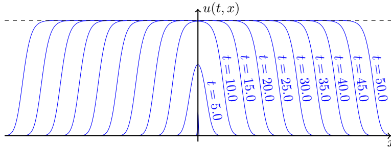
FIGURE 1.2 – Solutions de l'équation de Fisher-KPP partant d'une condition initiale concentrée en x = 0
