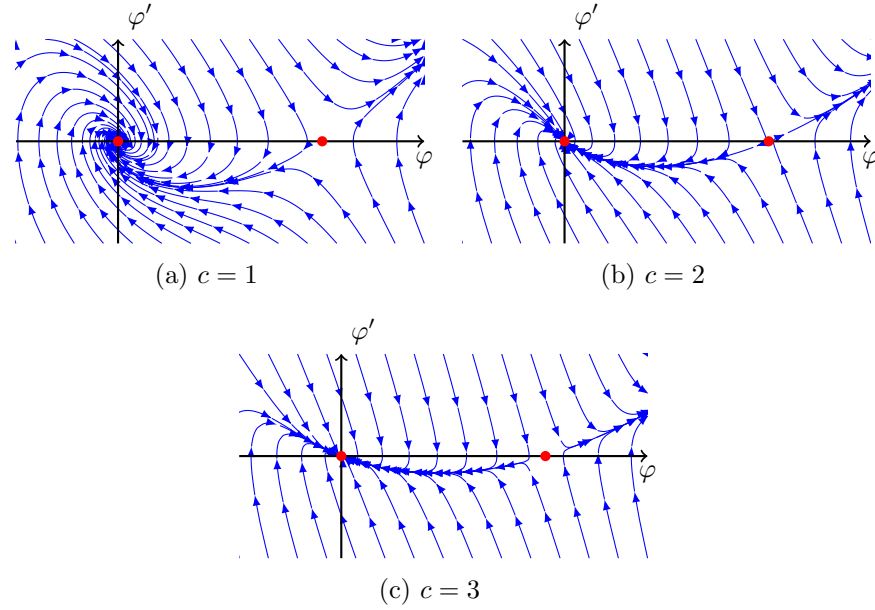
FIGURE 1.3 – Plan de phase de l’EDO des fronts progressifs pour Fisher-KPP. Les points rouges représentent les équilibres.
