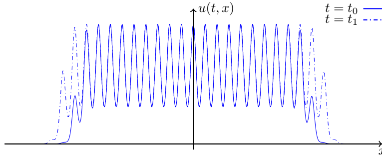
FIGURE 1.5 – Exemple de solution du problème de Cauchy (1.8) à deux temps proches t_0 < t_1 , pour la nonlinéarité f(x, u) = (\frac{1}{2} + \cos(x))u - u^2 et L = \partial_{xx} .
