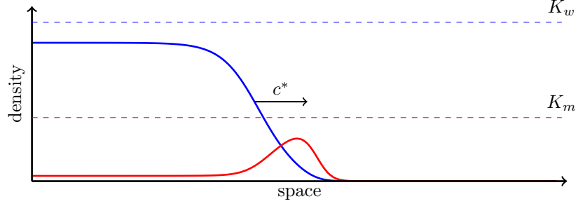
FIGURE 1.6 – Forme typique des fronts du système (1.19) (en bleu : I_w ; en rouge : I_m ).
