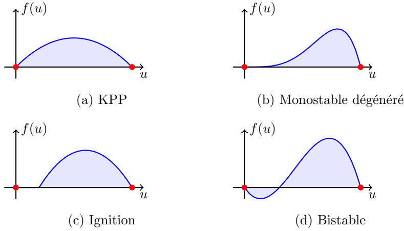
FIGURE 1.4 – Différents types de nonlinéarités
