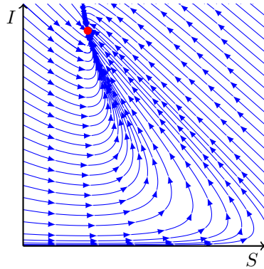
FIGURE 1.1 – Plan de phase associé au système (1.2)
