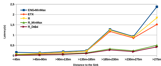
(c) Topologie arbitraire avec RX=100%
