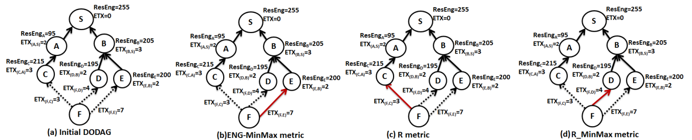
FIGURE 6.1 – Construction du DODAG RPL avec plusieurs métriques à partir du nœud F : (a) exemple de réseau avec le DODAG construit avant l’ajout de F, (b) choix du parent préféré avec la métrique ENG_MinMax, (c) choix du parent préféré avec la métrique R , (d) choix du parent préféré avec la métrique R\_MinMax proposée.
