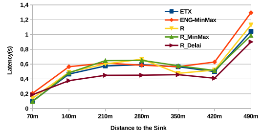
(d) topologie grille hétérogène 1 avec RX=60%
