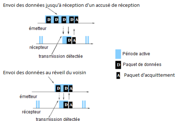
FIGURE 3.6 – Phase de transmission dans ContikiMAC [Dunkels 2011]
