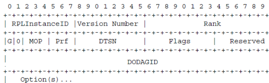
FIGURE 5.3 – Format des messages de type DIO [Vasseur et al. March 2012]
