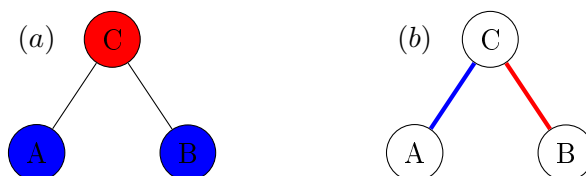
FIGURE 4.3 – Coloration de sommets et coloration d'arêtes.
