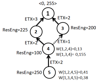
FIGURE 6.7 – Construction du DODAG RPL avec la métrique composite R\_Delai en prenant en compte la paire \langle ETX, ENG\_MinMax \rangle lors du choix du parent préféré.
