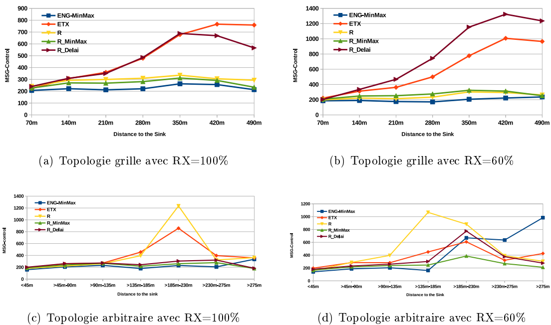
FIGURE 6.12 – Messages de contrôle.
