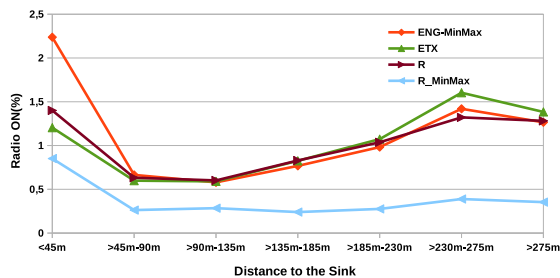
(c) Topologie arbitraire avec RX=100%
