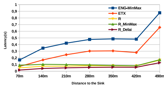
(a) Topologie grille avec RX=100%
