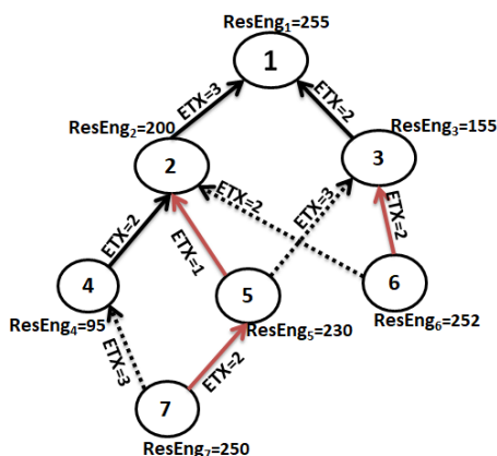
FIGURE 5.8 – Construction du DODAG avec la métrique ELT.
