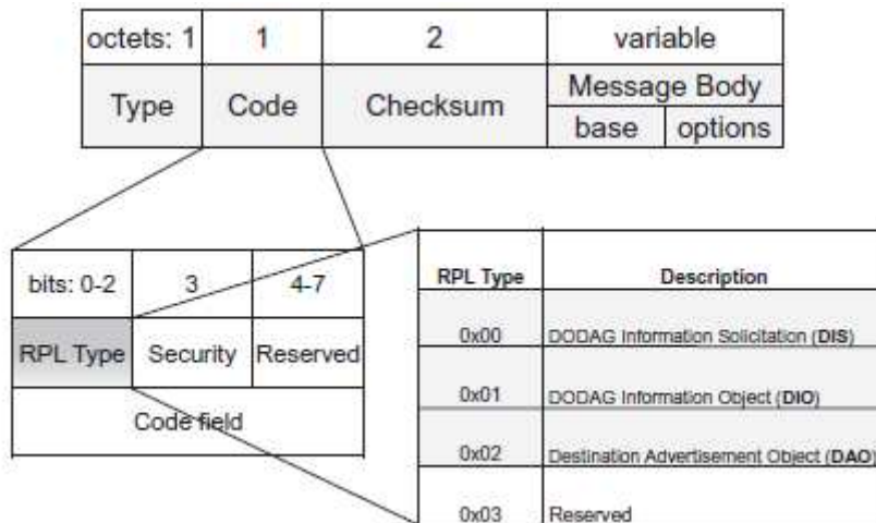
FIGURE 5.2 – Format des messages de contrôle RPL [Gaddour and Koubaa 2012]
