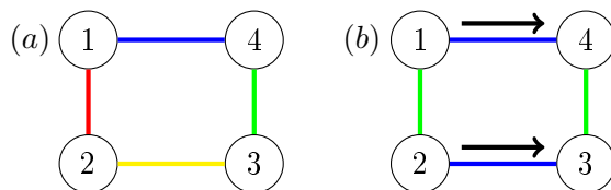
FIGURE 4.5 – Coloration non-orientée et orientée d'arêtes.
