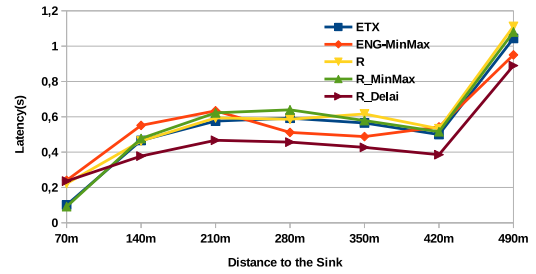
(f) topologie grille hétérogène 2 avec RX=60%
