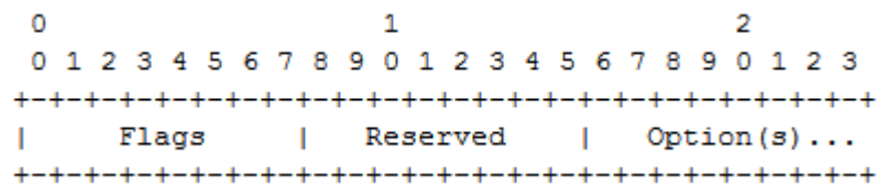
FIGURE 5.4 – Format des messages de type DIS [Vasseur et al. March 2012]
