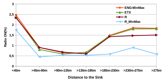
(d) Topologie arbitraire avec RX=60%
