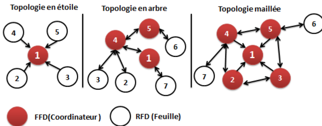
FIGURE 2.7 – Les topologies des réseaux de capteurs sans fil
