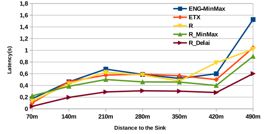
(b) topologie grille homogène avec RX=60%
