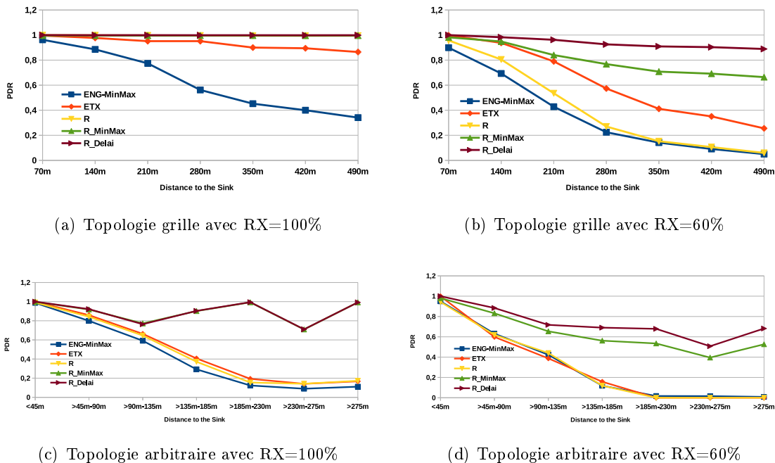
FIGURE 5.11 – Taux de livraison des paquets.
