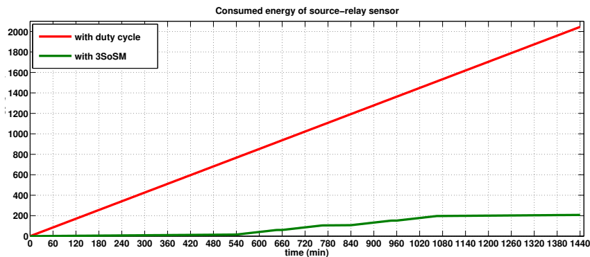
(d) Consumed energy of a source-relay device (24h).
