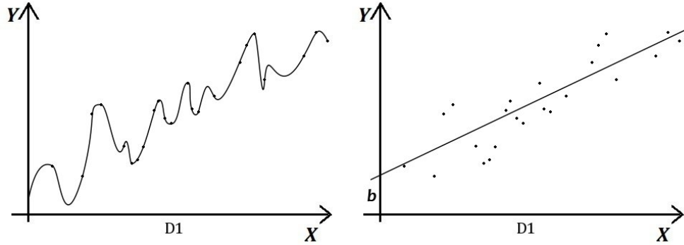
FIGURE 7.2 : Deux manières d'ajuster une courbe à un échantillon D_1 de n données représentées sous forme d'un nuage de points dans un repère : avec un polynôme de degré n - 1 : y = a_{n-1}x^{n-1} + \dots + a_1x + a_0 (à gauche) ; ou avec un polynôme de degré 1 : y = ax + b (à droite).
