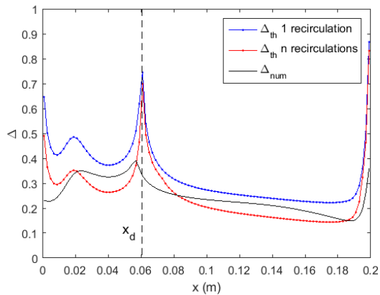
C2 : Profil de \Delta , Re_L = 10^5
