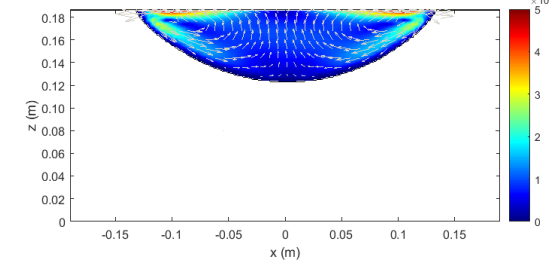
D2 - \|\vec{u}\| ( \text{m}\cdot\text{s}^{-1} ), t = 4.5 h.
