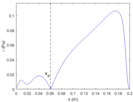
C1 : Profil de \tau , Re_L = 10^5
