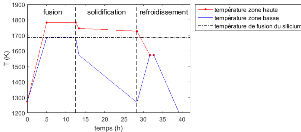
FIGURE 4.2 – Exemple de cycle thermique d'un procédé de solidification dirigée pour un lingot G2.
