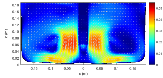
A2 - \|\vec{u}\| ( \text{m}\cdot\text{s}^{-1} ), t = 1 h.
