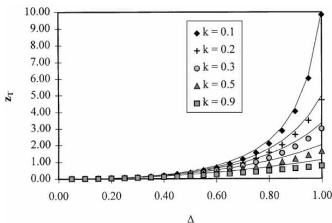
FIGURE 1.4 – Variation de la longueur du transitoire initial normalisée ( Z_T = z_T V_I/D_L ) en fonction de \Delta . Comparaison des solutions exacte (1.24) et approchée (1.25). Figure extraite de Garandet et al. [39].
