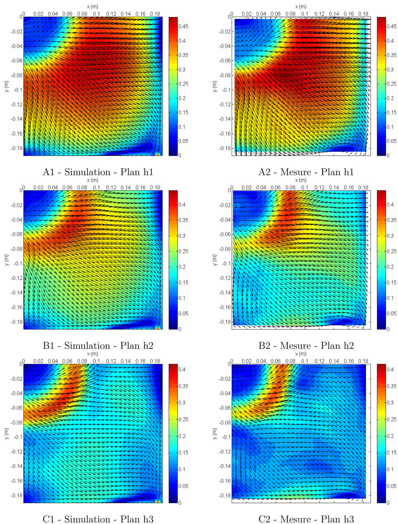
FIGURE B.2 – Comparaison des champs de vitesse normalisés numériques et expérimentaux pour la configuration 3 ( H = 15 cm et Re = 3.0 \times 10^5 ) dans les plans horizontaux. Les vecteurs représentent les deux composantes coplanaires de la vitesse ( V_x et V_y ) et les contours de couleurs représentent l'amplitude de ces vecteurs normalisés ( à suivre ).
