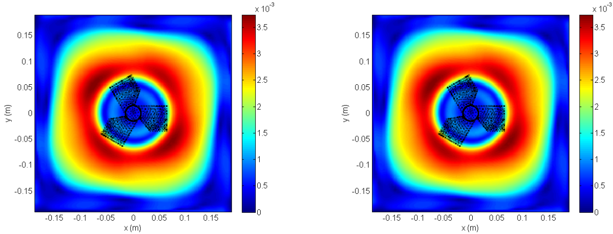
A - brassage Si 50 rpm
