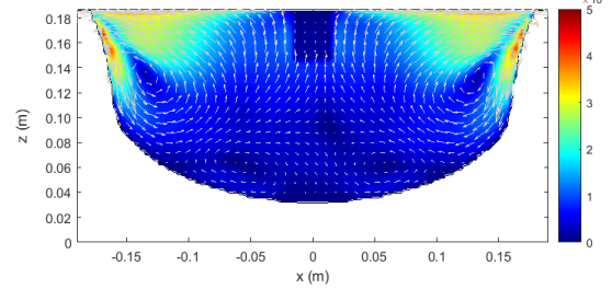
C2 - \|\vec{u}\| ( \text{m}\cdot\text{s}^{-1} ), t = 2.58 h.
