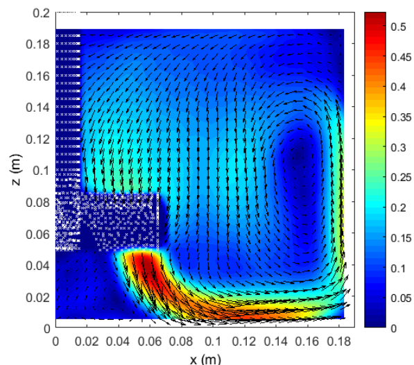
A2 - Mesure H = 20 cm ; N = 70 rpm
