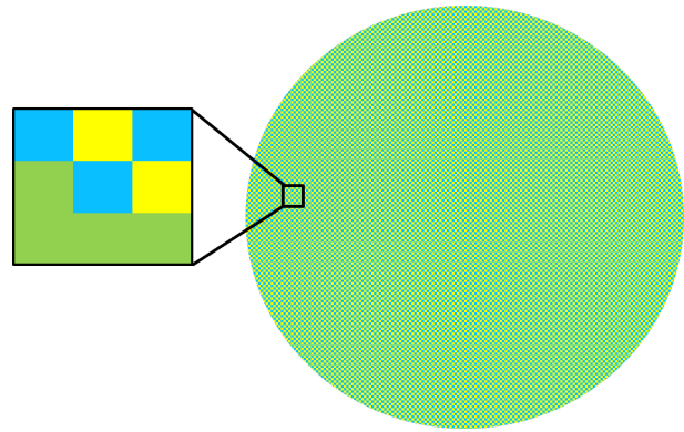
Figure 1.7 – Représentation conceptuelle de l’écart géophysique.
