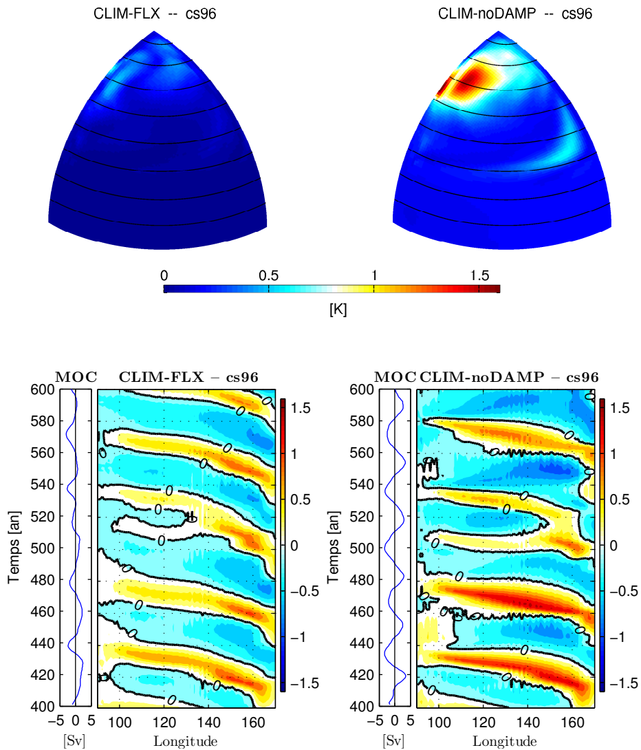
FIGURE 4.10 – Identique à la figure 4.9 pour la configuration cs96. Les anomalies de température sont moyennées entre 65\text{-}75^\circ\text{N} à 540 m de profondeur.
