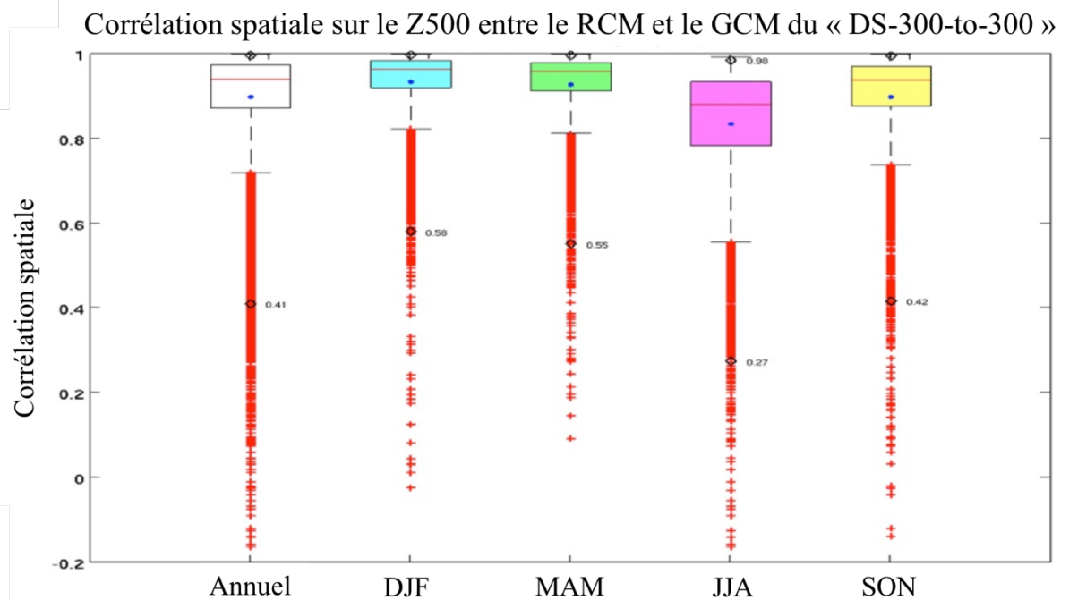
Figure 3. 7 : Comme Figure 3.6, mais pour le géopotentiel à 500 hPa.
