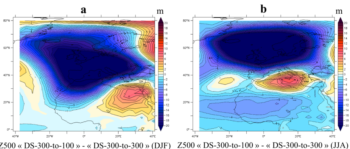
Figure 4.5 : Différence du géopotential à 500 ha en hiver (a) et en été (b), à l'issue de la soustraction des résultats « DS-300-to-100 » par « DS-300-to-300 ». Seul l'effet de la résolution est retenu, puisque celui de la relaxation a été éliminé par la soustraction.
