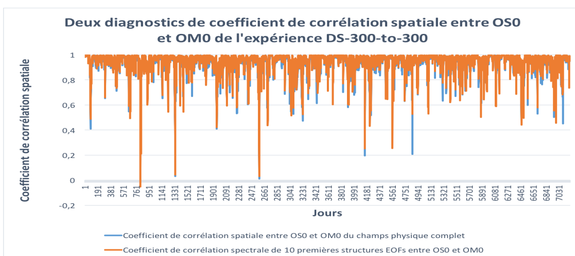
Figure 3. 13 : Coefficients de corrélation (variabilité synoptique seule) en fonction du temps, calculée sur Z500 entre OS0 (OWN) du RCM et OM0 (GCM) de l'expérience « DS-300-to-300 », par deux méthodes différentes en espace physique et espace spectrale des 10 premières composantes principales.
