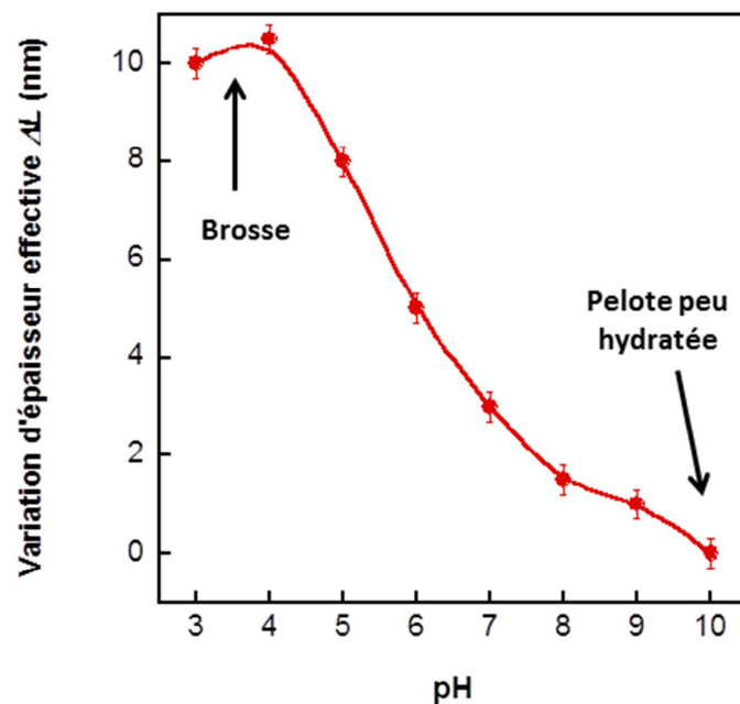
Figure 4.15 : Evolution de la variation d'épaisseur effective \Delta L (nm) d'un film de PDMAEMA en fonction de l'augmentation du pH ([KCl]=2mM).
