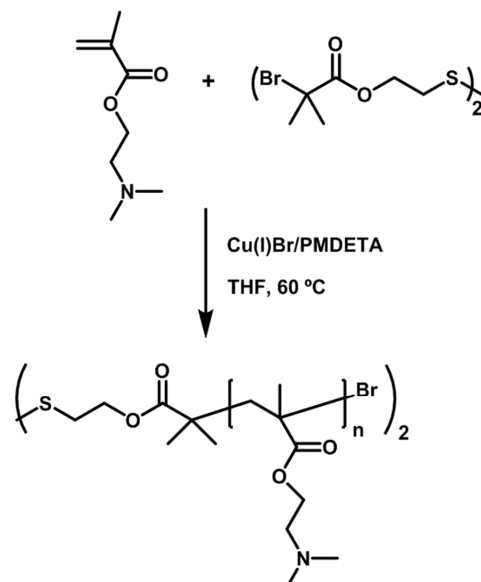
Figure 2.4 : Schéma réactionnel de l'ATRP pour l'obtention du (PDMAEMA n ) 2 S 2
