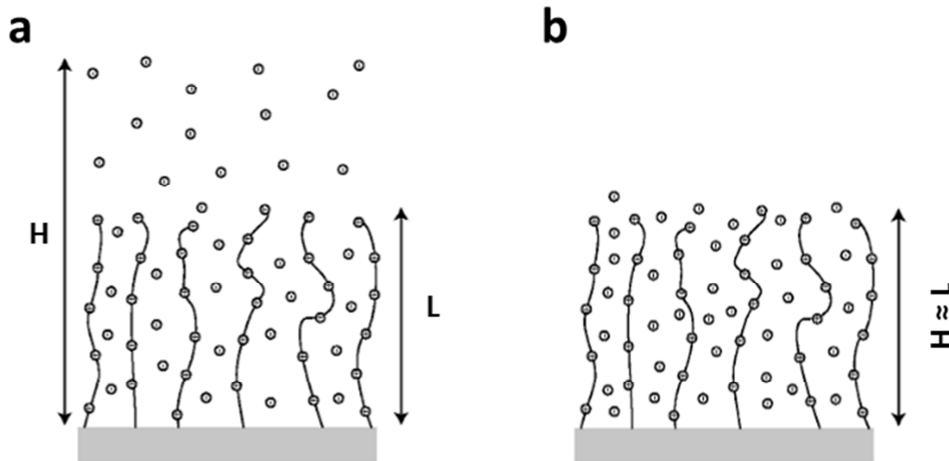
Figure 1.24 : Schéma de la structure des chaînes de polyélectrolytes avec (a) H > L et (b) H \approx L [123, 127]
