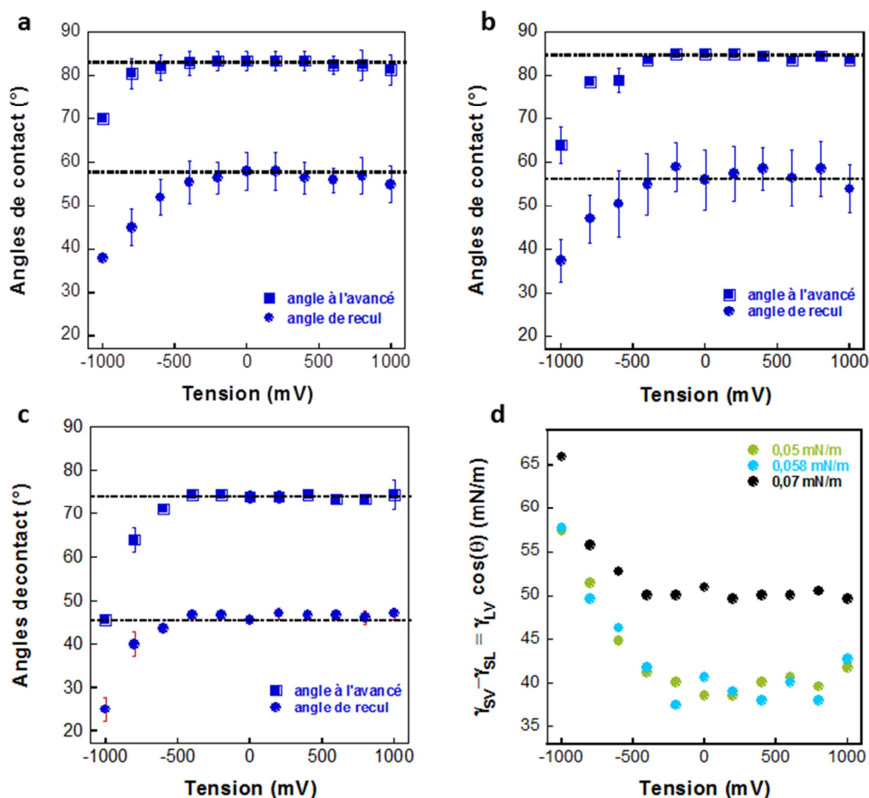
Figure 5.10 : Evolution des angles de contact de films de PS 36 PAA 125 lors de l'application d'un champ électrique pour des densités égales à 0.05 chaînes/nm 2 (a), 0.058 chaînes/nm 2 (b), 0.07 chaînes/nm 2 (c) et (d) évolution de \gamma_{SV} - \gamma_{SL} = \gamma_{LV}\cos(\theta) pour l'angle de contact de recul en fonction de la tension appliquée pour les différentes densités de greffage des chaînes de PAA
