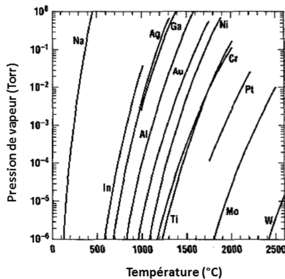
Figure 2.7 : Pressions de vapeur de différents métaux en fonction de la température [9]
