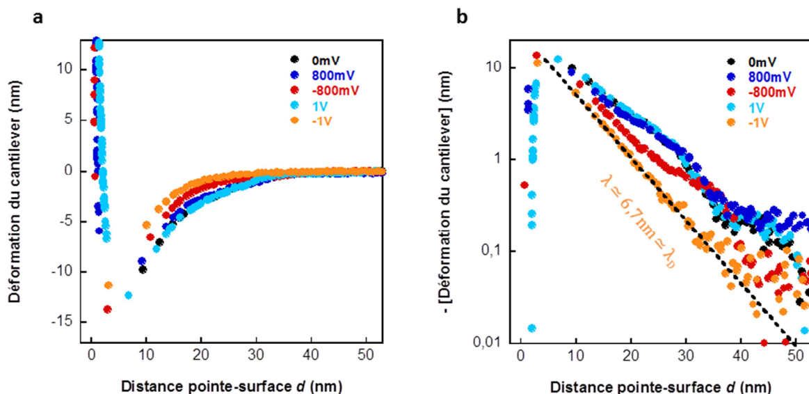
Figure 5.21 : (a) Courbes moyennes d'interactions entre la pointe de silice et un film de PS 72 P2VP 119 (0,04 chaîne/nm 2 ) et (b) représentation en échelle semi-log des valeurs de la déformation du cantilever (pH=3 ; [KCl]=1mM)
