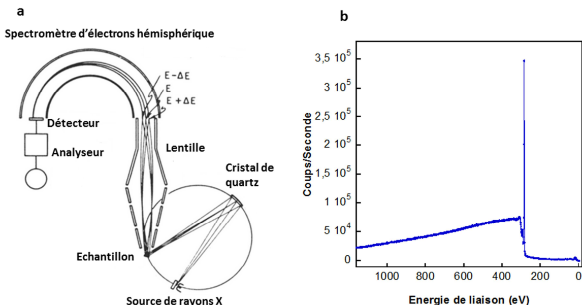
Figure 2.17 : (a) Schéma du fonctionnement de l'XPS [24] et (b) spectre XPS d'un film de PS de 50nm
