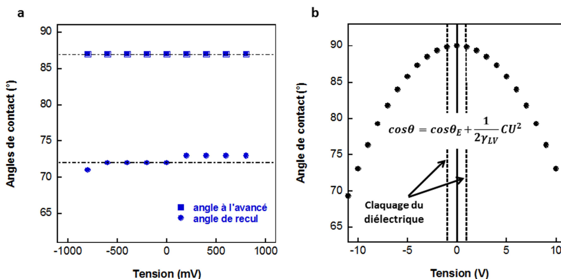
Figure 5.6 : (a) Mesure expérimentale des angles de contact d'un film de PS de 50nm mouillé par une goutte d'eau (pH 4 ; [KCl] = 2mM) lors de l'application d'une tension électrique et (b) variation d'angle de contact calculée pour un film de PS de 50nm à partir de l'équation de Young-Lippmann (énoncée sur la Figure)
