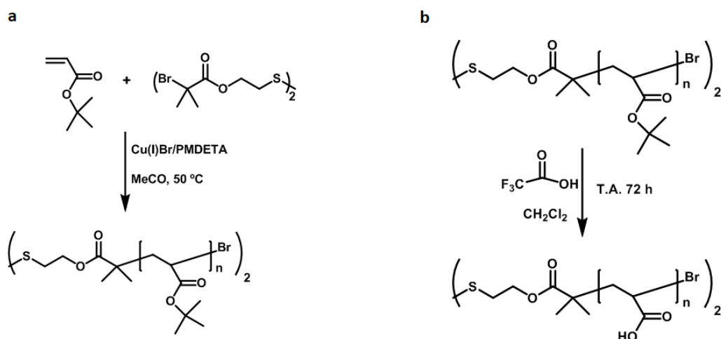
Figure 2.3 : Schémas réactionnels de l'ATRP pour l'obtention du (tBA 47 ) 2 S 2 (a) et de l'hydrolyse du (tBA 47 ) 2 S 2 (b)
