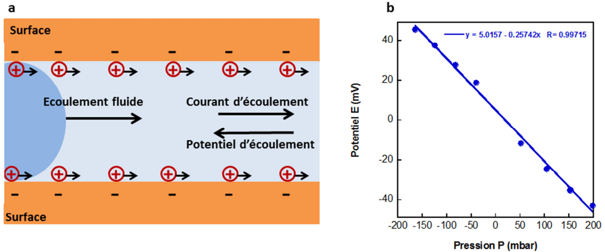
Figure 2.22 : (a) Schéma de la technique de potentiel d'écoulement et (b) linéarité de l'évolution de E avec P pour des wafers de silicium dans une solution aqueuse à pH=9 et [KCl]=5.10^{-4}M ( \zeta=-30mV )
