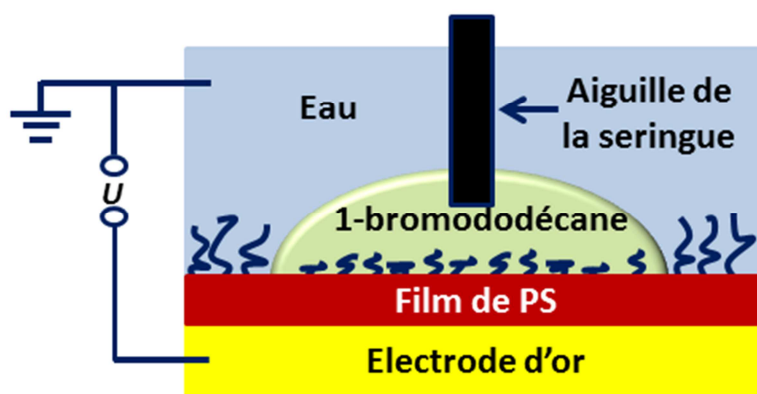
Figure 2.36 : Schéma du montage de l'électro-mouillage en milieu liquide
