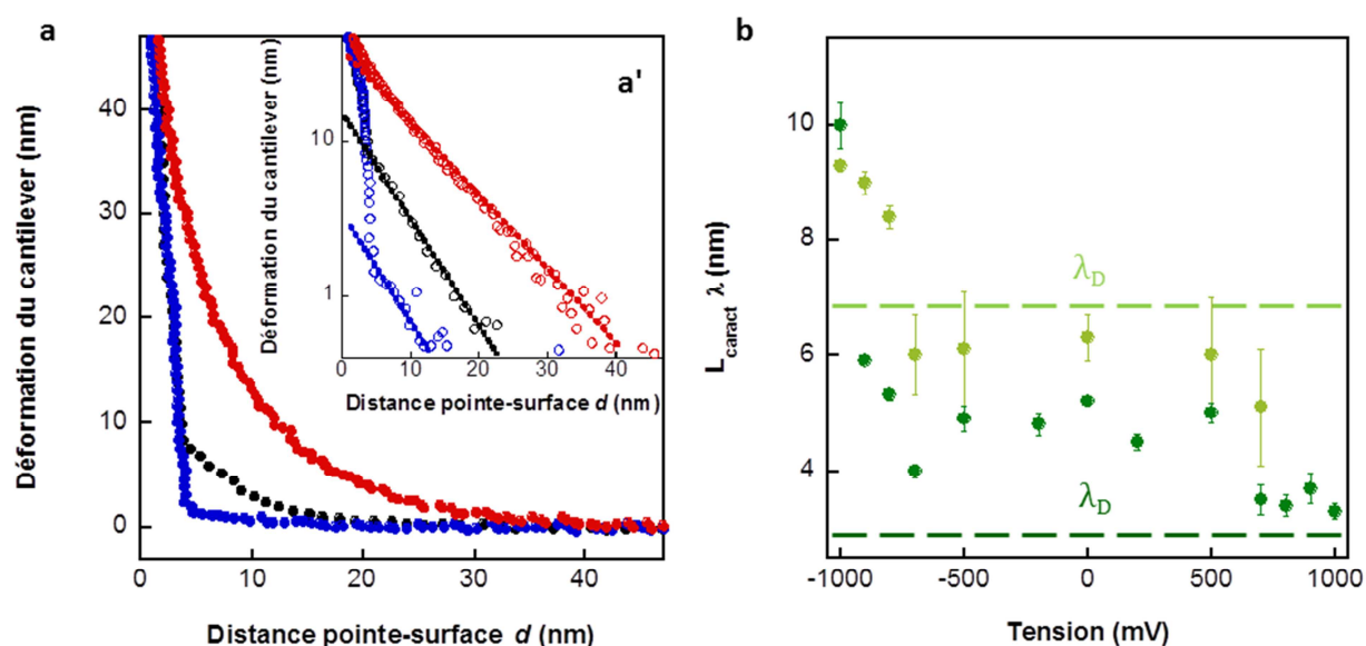
Figure 5.15 : Courbes d'interactions entre la pointe de silice et un film de PS 36 PAA 125 pour des tensions de 0mV (noir), 800mV (bleu) et -800mV (rouge) représentées en échelle linéaire (a) et semi-log (a'). (b) Longueurs caractéristiques \lambda de la répulsion mesurées pour différentes tensions à des concentrations en KCl de 2mM (vert clair) et 8mM (vert foncé) (pH=4.5)
