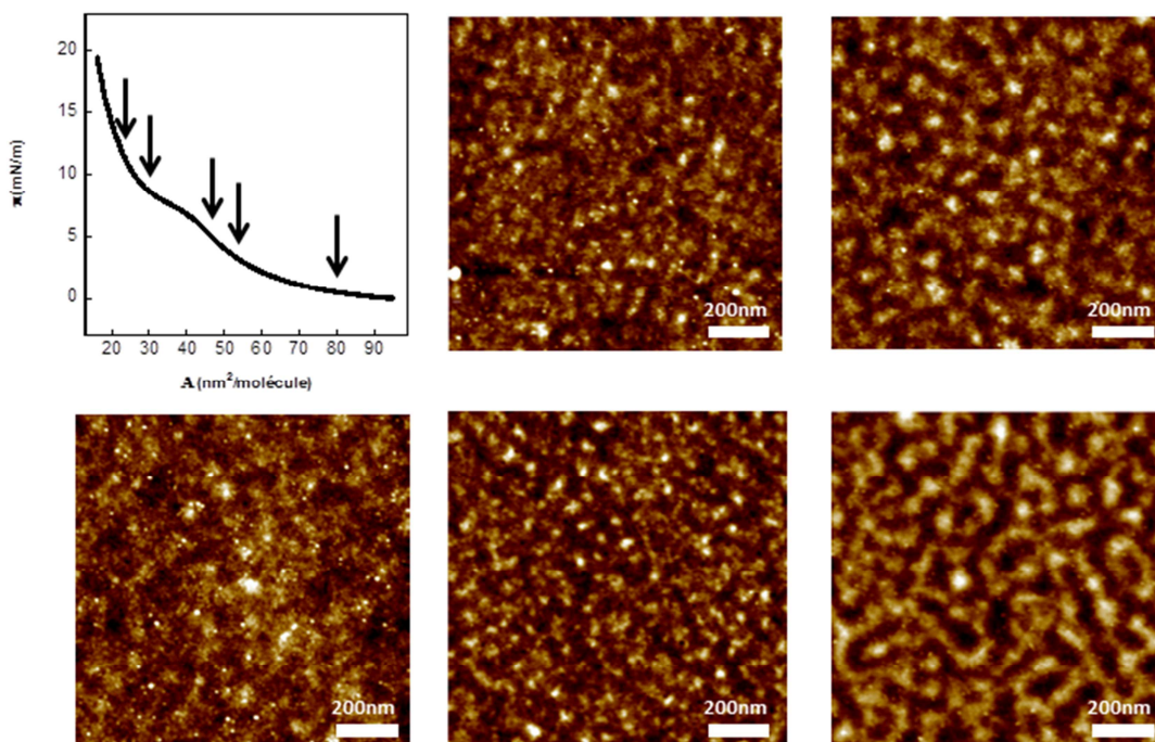
Figure 3.7 : (a) Isotherme de compression de films de PS 72 P2VP 119 à l'interface entre l'eau (pH = 4 ; 0.1M NaCl) et l'air. Les flèches indiquent les pressions de surface et les aires par molécule pour les transferts dont sont obtenues les images AFM. (b) à (f) : images AFM de hauteur en mode tapping pour des molécules transférées à (b) 0.5mN/m, (c) 4mN/m, (d) 6mN/m, (e) 10mN/m et (f) 12mN/m
