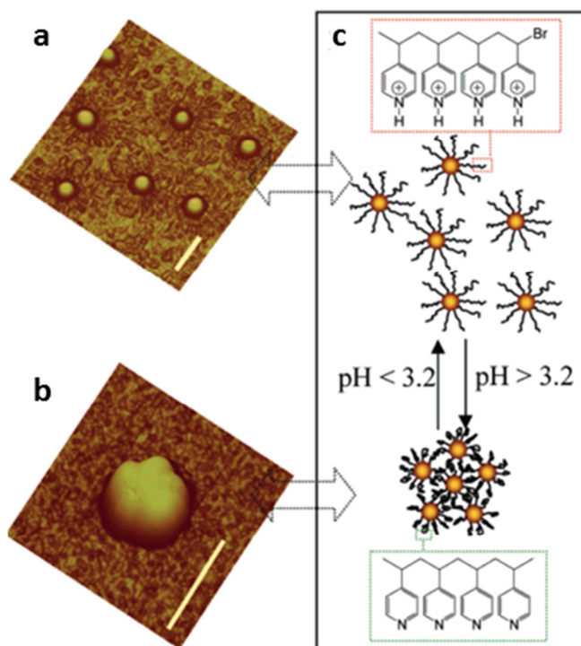
Figure 1.8 : Particules d'or décorées avec des brosses de P4VP à pH inférieur à 3,2 (a) et supérieur à 3.2 (b) et (c) schéma expliquant la réversibilité de l'agrégation des particules [38]
