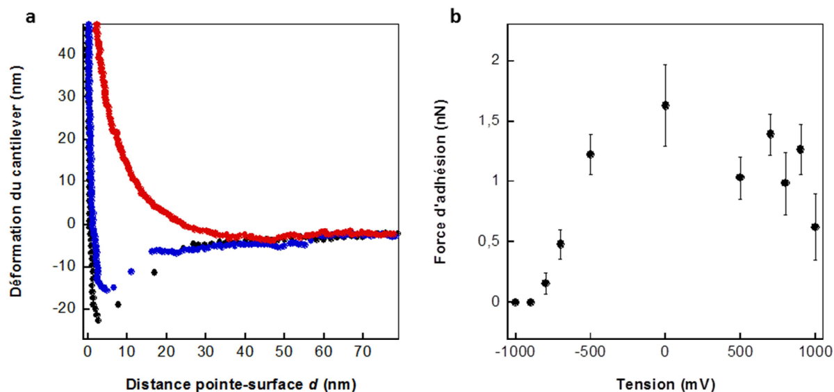
Figure 5.17 : (a) Courbes de retrait entre la pointe de silice et un film de \text{PS}_{36}\text{PAA}_{125} ( \sigma = 0.05 chaînes/ \text{nm}^2 ) pour des tensions de 0mV (noir), 800mV (bleu) et -800mV (rouge) et (b) forces d'adhésions moyennes obtenues en fonction de la tension appliquée (pH=4.5, [KCl]=2mM).
