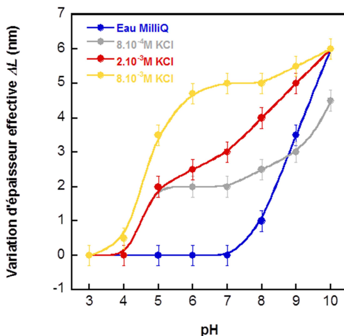
Figure 4.8 : Evolution de la variation d'épaisseur \Delta L (en nm) d'un film de (PAA_{47})_2S_2 mesurée à l'aide de la QCM-D, en fonction du pH, pour différentes concentrations en KCl dans la solution
