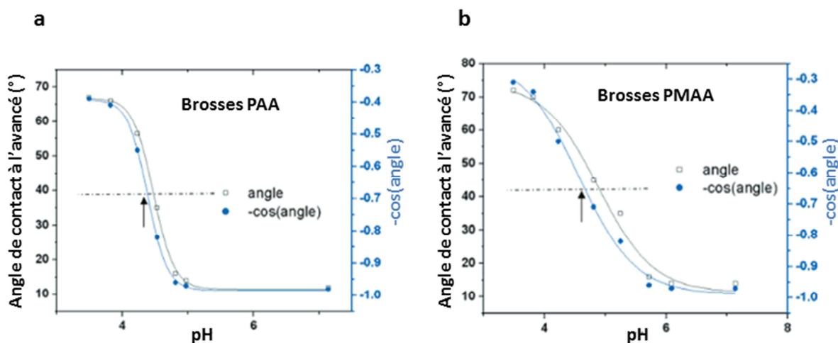
Figure 1.7 : Evolution de l'angle de contact à l'avancé et de son cosinus pour des brosses de PAA (a) et de PMAA (b) en fonction du pH [31]
