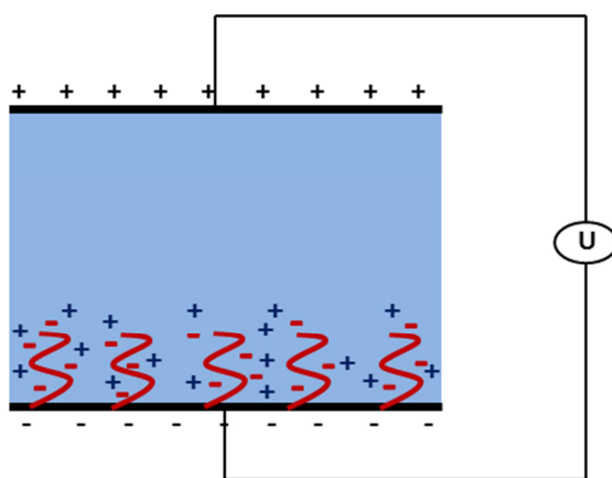
Figure 1.28 : Surface chargée de même signe que les charges sur les chaînes des polyélectrolytes. Rouge : charges sur les chaînes ; bleu : contre-ions.
