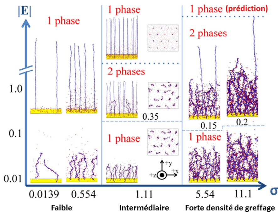
Figure 1.29 : Comportement de polyélectrolytes forts en fonction de la tension appliquée et de la densité de greffage [141]
