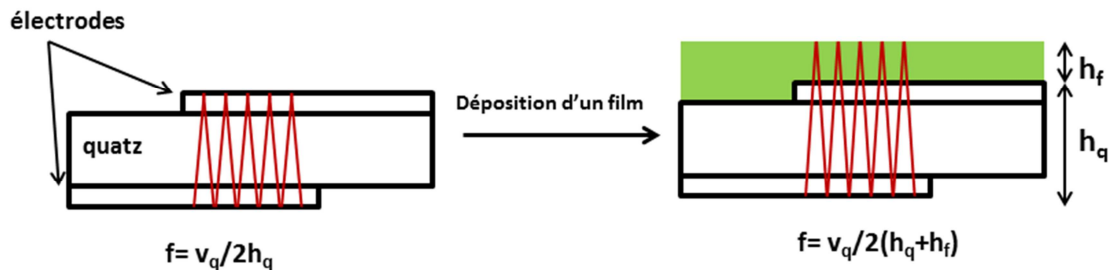
Figure 2.25 : Variation de la fréquence de l'onde acoustique après le dépôt d'un film sur le quartz ( v_q vitesse du son dans le quartz, h_q épaisseur du quartz et des électrodes et h_f épaisseur du film déposé)
