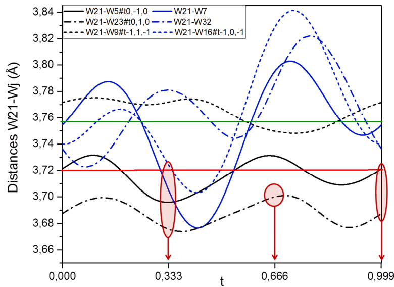
Figure 26 : Evolution des distances W_{21}-W_j , en Å, en fonction de t . Même légende que figure 24.
