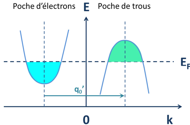
Figure 6 : Représentation schématique des poches d'électrons et de trous résiduelles après un nesting imparfait de la Surface de Fermi.
