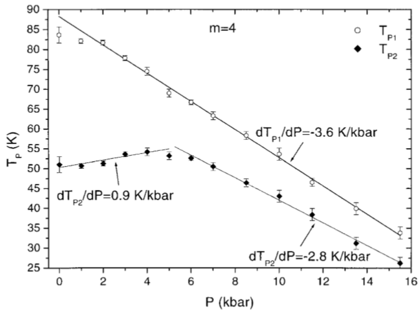
Figure 32 : Evolution des températures de transition ODC en fonction de la pression pour un cristal de m=4 [Beille2001].
