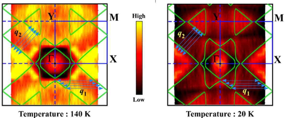
Figure 13 : Intensité spectrale ARPES à l'énergie de Fermi du composé P_4W_{12}O_{44} à 140K et 20K, c'est-à-dire au-dessus et en dessous des températures de transition T_{c1} et T_{c2} correspondant respectivement aux vecteurs de nesting \mathbf{q}_1 et \mathbf{q}_2 déterminés par diffraction des rayons X (tableau 1). L'emboîtement partiel de portions plates de la Surface de Fermi par \mathbf{q}_1 et \mathbf{q}_2 est mis en évidence. [Paul2014][Paul2016]
