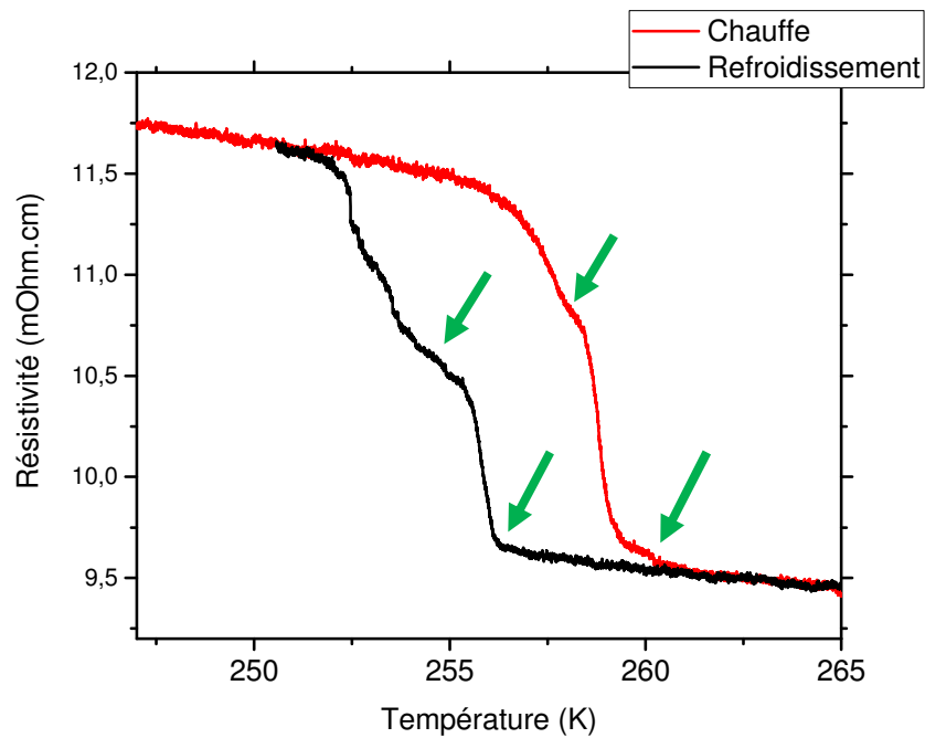
Figure 41 : Détail de la figure 40 (noté I) révélant l'existence deux transitions très proche en température. Les flèches visualisent les débuts de transition.
