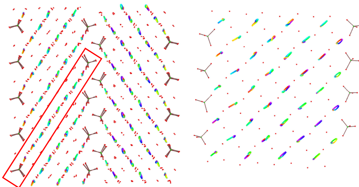
Figure 30 : Structure modulée du m=8 à 200K. Les déplacements des atomes W, P, O (respectivement en violet, vert et rouge) ont été multipliés par un facteur 3. Les courbes de Lissajous représentant les déplacements des atomes dans le cristal modulé sont dessinées pour les tungstènes. A gauche, projection selon a , à droite vue à 90^\circ d'un ruban identifié par un cadre rouge sur la projection selon a . Dessins réalisés à l'aide de Molecoolqt [Hübschle2011].
