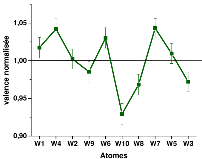
Figure 20 : Représentation de la valeur de la valence normalisée pour chaque atome de tungstène de la chaîne d'octaèdres constituant le matériau.
