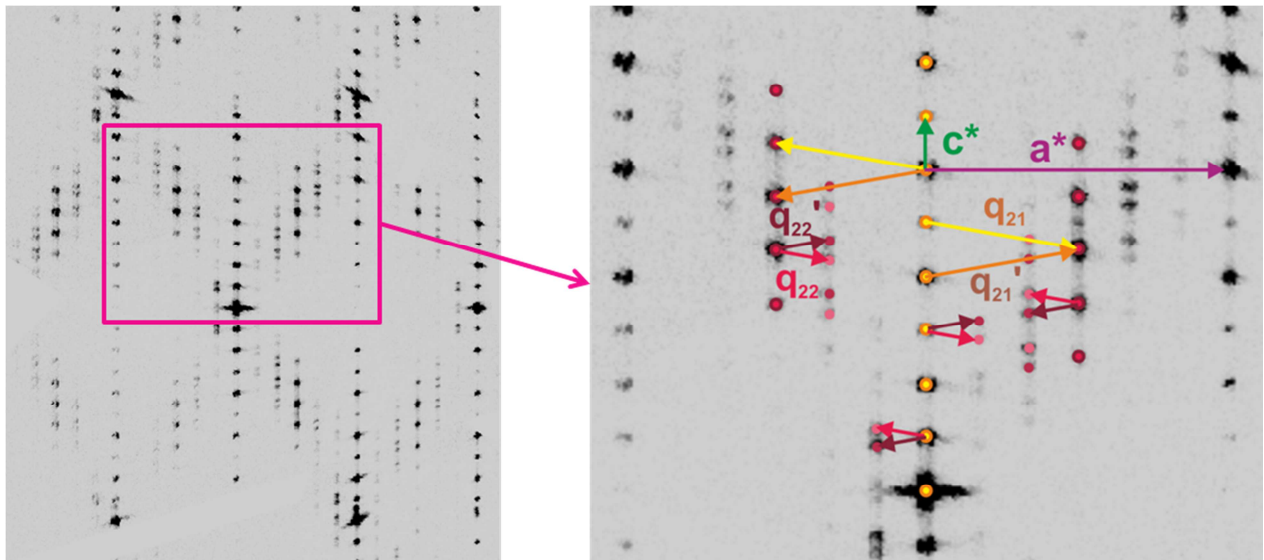
Figure 13 : Indexation des réflexions satellites caractéristiques de l'état ② du m=8 . Les vecteurs de modulation jaune ( q_{21} ) et rose ( q_{22} ) correspondent au premier individu de la macle et les vecteurs orange ( q_{21}' ) et rouge foncé ( q_{22}' ) au deuxième élément.
