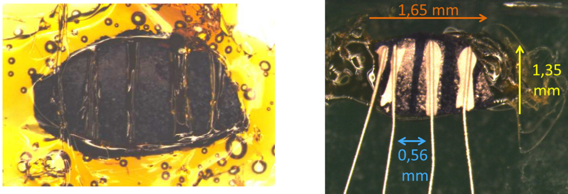
Figure 49 : Images d'un cristal de m=8 sans réflexion satellite à 220K après application d'un masque au vernis « General Electric » et après dépôt de platine et pose de 4 contacts.
