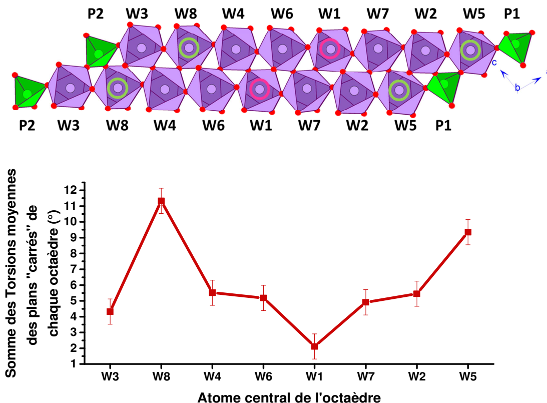
Figure 31 : Représentation de la chaîne d'octaèdres étudiée ainsi que des sommes de torsions moyennes associées à chacun de ces octaèdres. Les atomes centraux des polyèdres les moins déformés sont indiqués par un anneau rose et ceux des plus déformés par un anneau vert.
