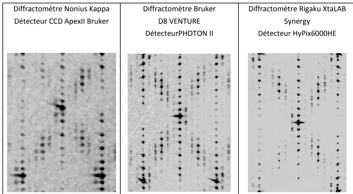
Figure 9 : Reconstitution d'une partie du plan (h0l)^* du deuxième état ② du m=8 à partir d'images obtenues à l'aide de différents diffractomètres.
