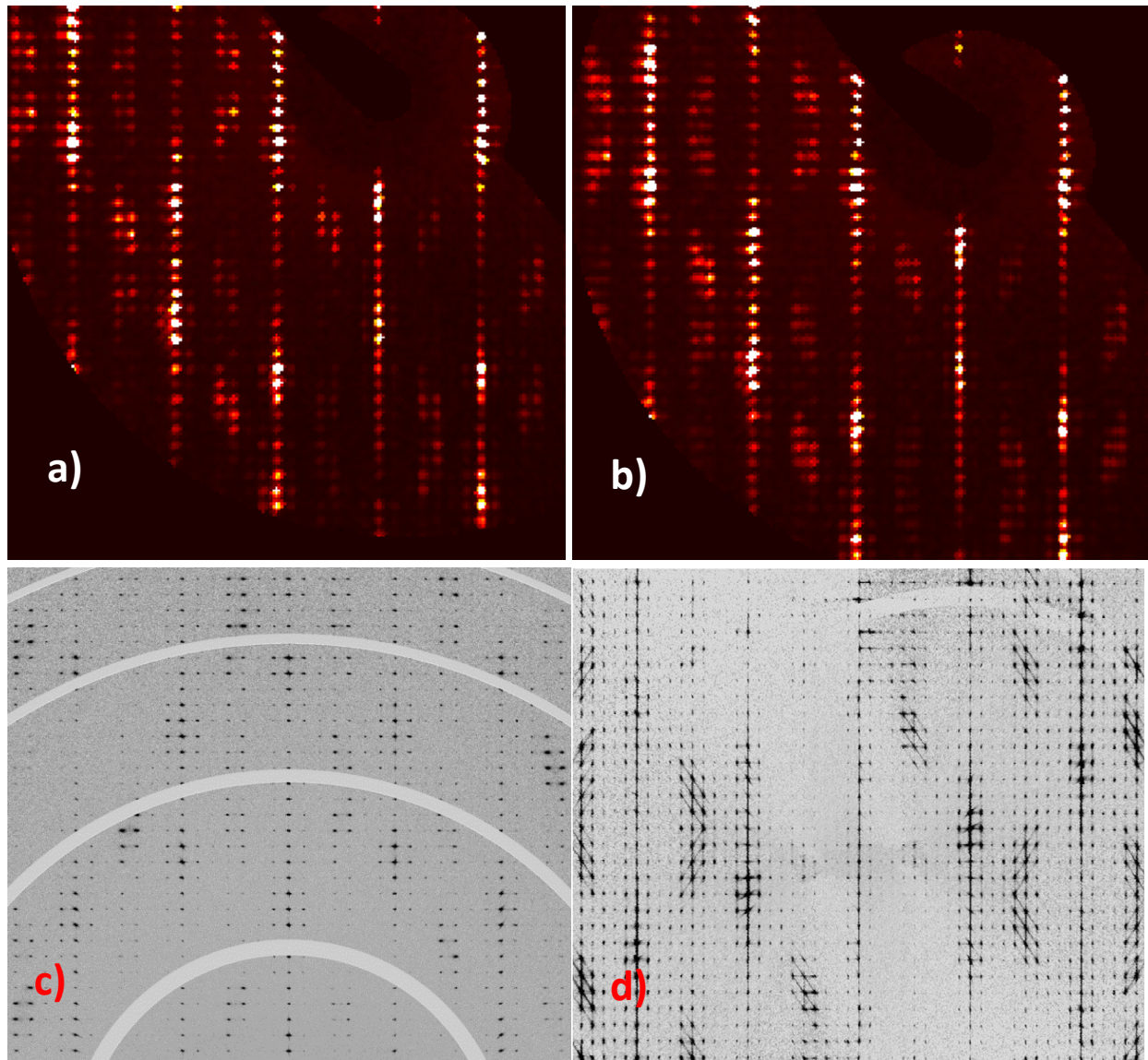
Figure 11 : Plans de diffraction (h0\ell)^* reconstitués à partir d'images expérimentales mesurées au laboratoire CRISMAT avec un diffractomètre équipé d'un détecteur CCD APEXII (a) à température ambiante et (b) à 100K), à l'ESRF sur la ligne BM01a avec détecteur Pilatus 2M (c) à température ambiante) et toujours à l'ESRF sur la ligne ID23 avec un détecteur Pilatus 6M (d) à 100K.
