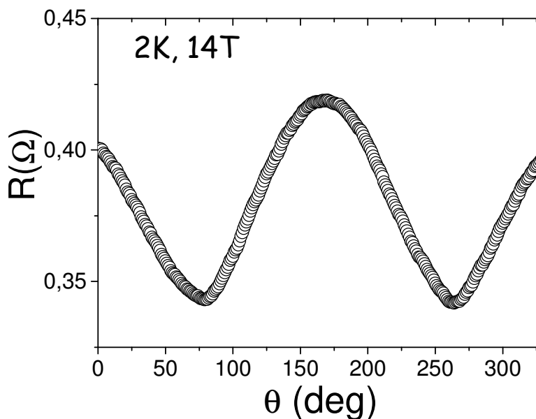
Figure 57 : Evolution de la valeur de la résistance en fonction de l'orientation du champ magnétique par rapport au cristal, avec \theta l'angle entre le champ magnétique appliqué et l'axe c du cristal.
