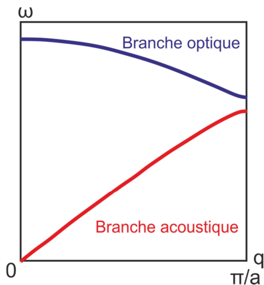
Figure 19 : Spectre de dispersion théorique des phonons. Deux branches de phonon sont identifiables : une branche optique et une branche acoustique.
