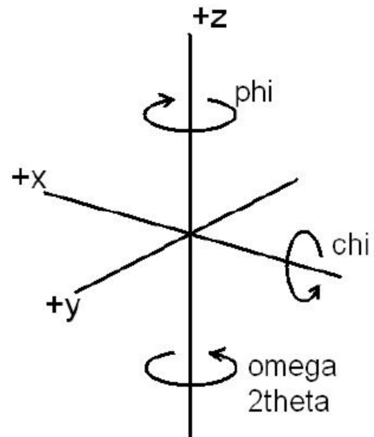
Figure 37 : Définitions des angles de rotation du goniomètre Kappa
