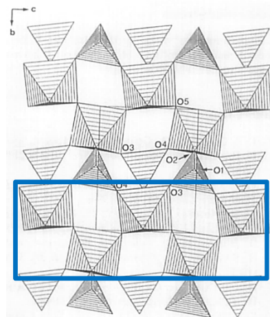
Figure 22 : Représentation de la structure du MPTBp m=2 vue suivant l'axe a [Wang1989]. Cette figure met en évidence la présence de chaînes unidimensionnelles courant suivant c , comme montré par l'encadré bleu.
