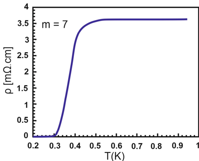
Figure 11 : Mesure de la résistivité du MPTBp m=7 , P_4W_{14}O_{50} , à très basses températures [Hess1997c].
