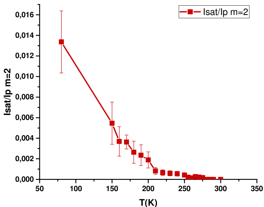
Figure 45 : Evolution de l'intensité des réflexions satellites du second ordre par rapport à l'intensité des réflexions principales en fonction de la température.
