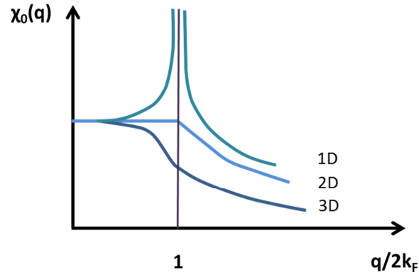
Figure 3 : Variation de la susceptibilité électronique en fonction de la valeur de q pour différentes dimensionnalités électroniques [Dugdale2016].
