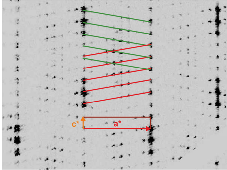
Figure 12: Reconstruction du plan (h2\ell)^* du MPTBp m=8 avec mise en évidence de la localisation des réflexions satellites des deux éléments de la macle apparaissant à l'état ①. Sur les lignes vertes sont placées les réflexions appartenant au premier élément, indexées par le vecteur de modulation \mathbf{q}_{11} . Celles du deuxième individu, indexées à l'aide de \mathbf{q}_{11}' , sont situées sur les lignes rouges.
