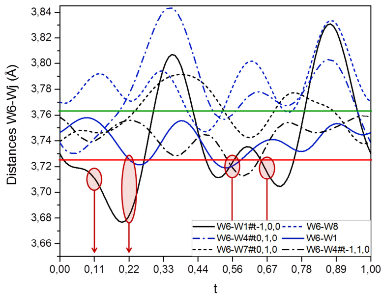
Figure 36 : Evolution des distances W6-W_j , en Å, en fonction de t . Même légende que figure 35.
