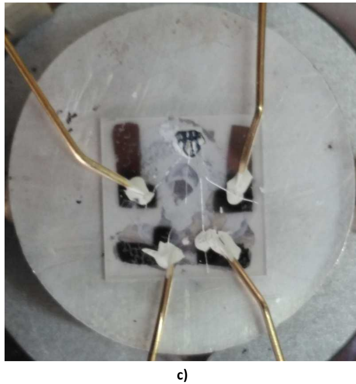
Figure 2 : Photographies du montage expérimental, en a) est représentée la platine chauffante/refroidissante Linkam© utilisée lors des mesures de résistivité pour le terme m=10 . L'intérieur de la platine est montré en b). Quatre pointes en or permettent d'injecter le courant dans le cristal par les plots latéraux déposés sur le cristal et de mesurer la tension au niveau des deux plots centraux du cristal. Un agrandissement de la lame de saphir sur laquelle est fixé le cristal vous est présenté en c). Nous pouvons y voir les quatre plots déposés sur la lame en vue de faire des contacts déportés. Les fils d'argent contactés sur le cristal sont alors fixés sur chaque plot à l'aide de laque d'argent époxy et les pointes d'or ont alors été plongées dans la goutte de laque avant de subir un recuit.
