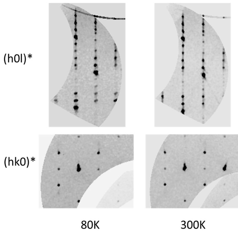
Figure 53 : Suivi d'une portion des plans (h0\ell)^* et (hk0)^* en température du deuxième cristal.
