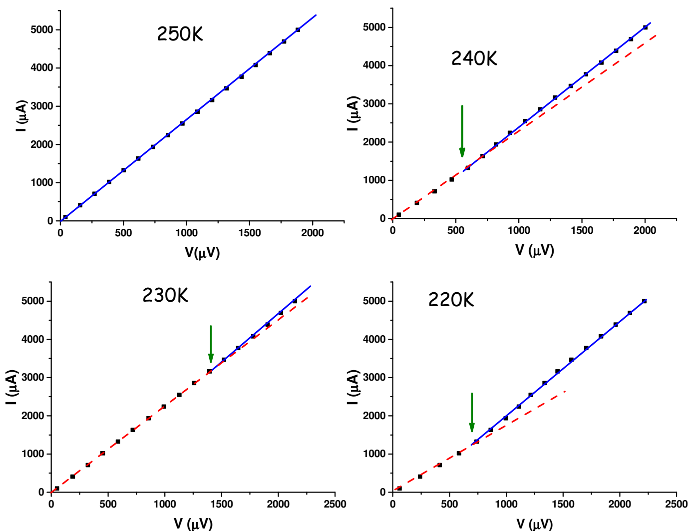
Figure 41 : Courbes I(V) obtenues pour le m=2 à différentes températures. Les droites bleues et rouges permettent d'ajuster les comportements aux régimes hautes valeurs de courant et basses valeurs de courant respectivement. Le point d'inflexion signalé par une flèche verte révèle la non linéarité et pointe le courant à partir duquel l'onde est dépiégée. Dans ce cas, la droite bleue représenterait le régime de glissement de l'ODC et la droite rouge le régime où l'ODC est ancrée au matériau.
