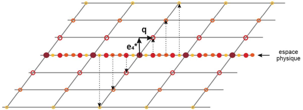
Figure 14 : Schéma de la reconstruction d'un réseau réciproque périodique à partir de la théorie superspace donnée par De Wolff. La ligne représentant l'espace physique est en fait le diagramme de diffraction réel.
