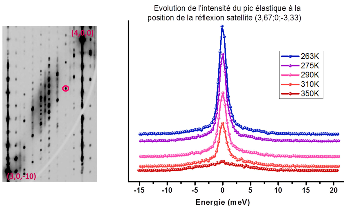
Figure 70 : Intensité de la diffusion élastique à la position (3,67 ; 0 ; -3,33) en fonction de la température.
