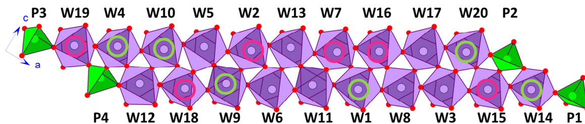
Figure 21: Représentation de la somme des torsions moyennes de chaque plan « carré », constitué de quatre atomes d'oxygène, de chaque octaèdre. La position des octaèdres les moins distordus est marquée par un anneau rose et celle des octaèdres les plus distordus d'un anneau vert.
