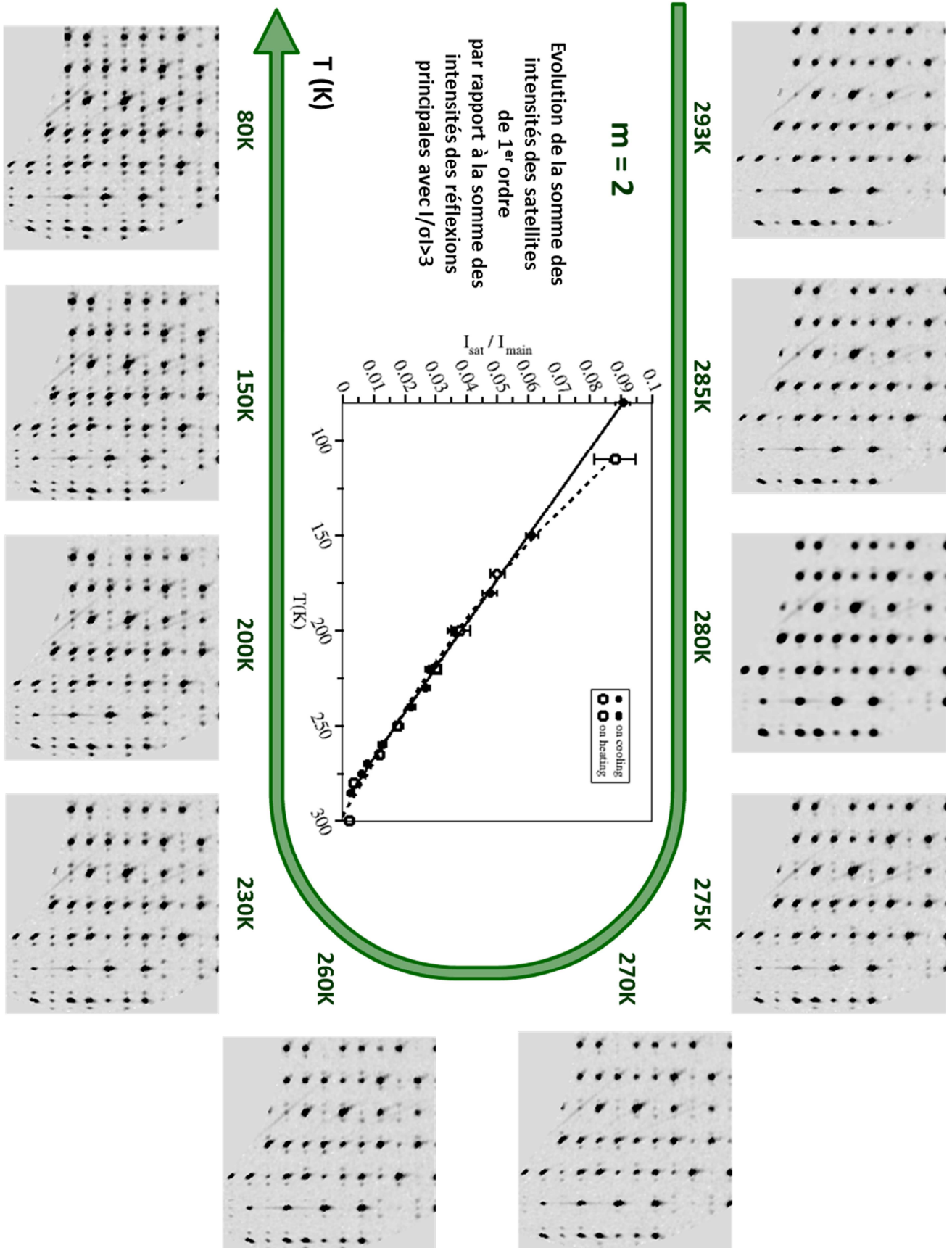
Figure 24 : Suivi en température du plan (0k\ell)^* et de l'intensité des réflexions satellites du premier ordre d'un cristal de m=2 .
