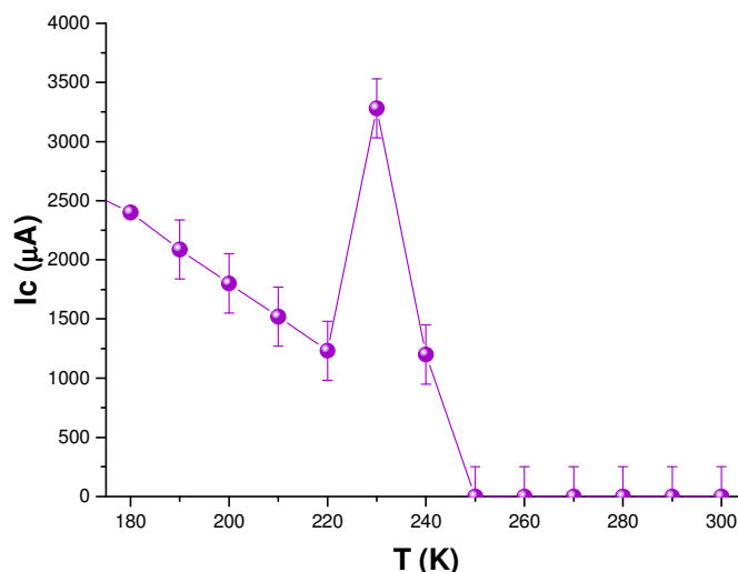
Figure 44 : Evolution de la valeur de courant à injecter dans le matériau pour atteindre le régime de glissement de l'ODC.
