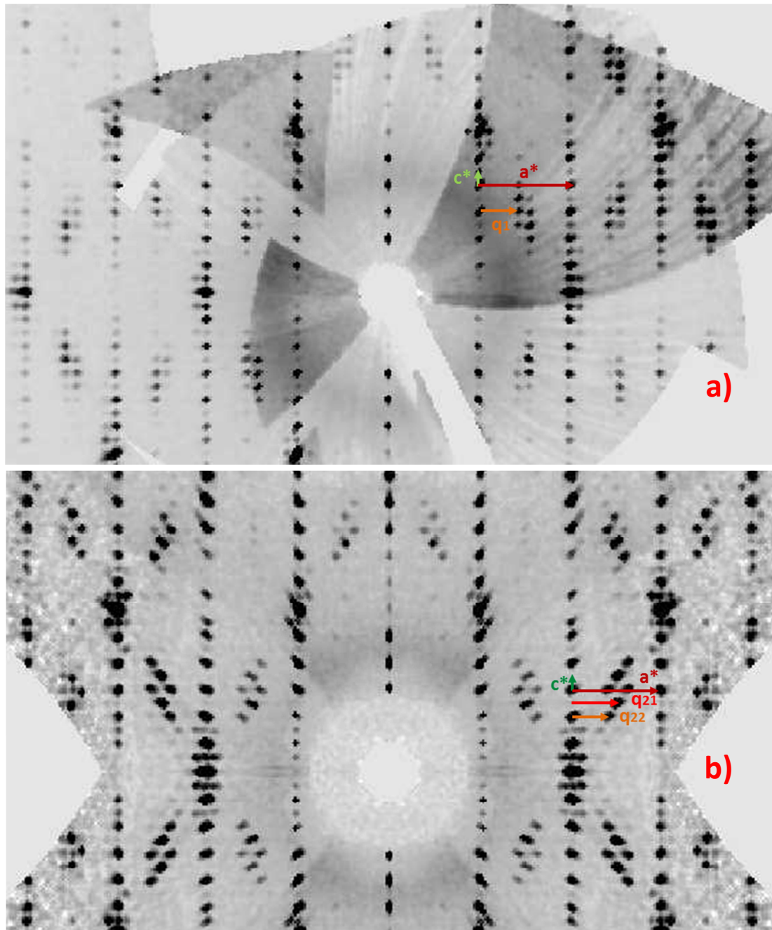
Figure 4 : Reconstruction du plan (h0l)^* pour le m=10 à température ambiante. a) état ① présentant le vecteur de modulation q_1=3/7a^* observé par Roussel et al. b) état ② présentant deux vecteurs de modulation: q_{21}=1/2a^* et q_{22}=2/5a^* .
