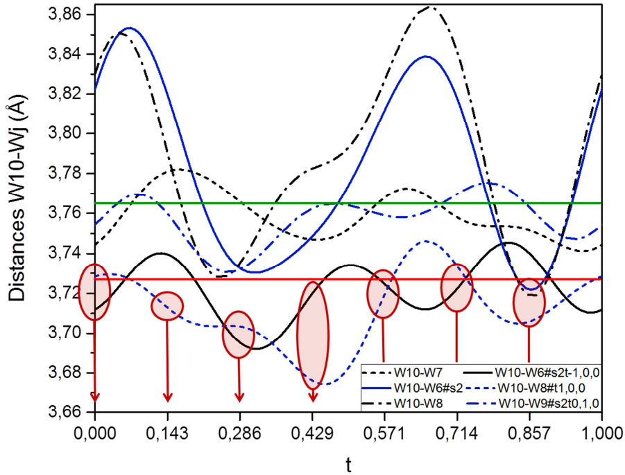
Figure 19 : Variations des distances W10-W_j , en Å, en fonction de t . Même légende que la figure 17.
