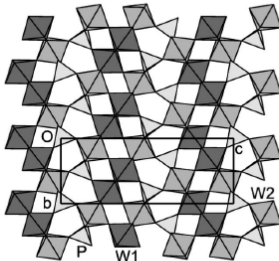
Figure 6 : structure du terme m=4 déterminée à 20K par Lüdecke et al [Lüdecke2001]. Les octaèdres les plus foncés correspondent aux tungstènes d'où serait originaire l'onde de densité de charges.
