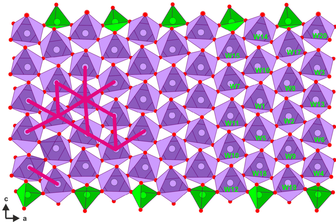
Figure 24 : Représentation de la couche constituant la structure de l'état \odot du MPTBp m=10 vue suivant b . Les distances W_i-W_j impliquées dans les regroupements de tungstènes mis en évidence sur les figures 25, 26, 27, 28 et 29 sont représentées par un bâtonnet rose permettant la visualisation de la position au sein de la couche des amas de tungstènes observés pour certaines sections t . Un amas d'atomes de tungstène, massif, est mis en évidence au centre de la couche de WO_3 ainsi que l'existence d'un dimère en bord de couche, formé de W19 et W18.
