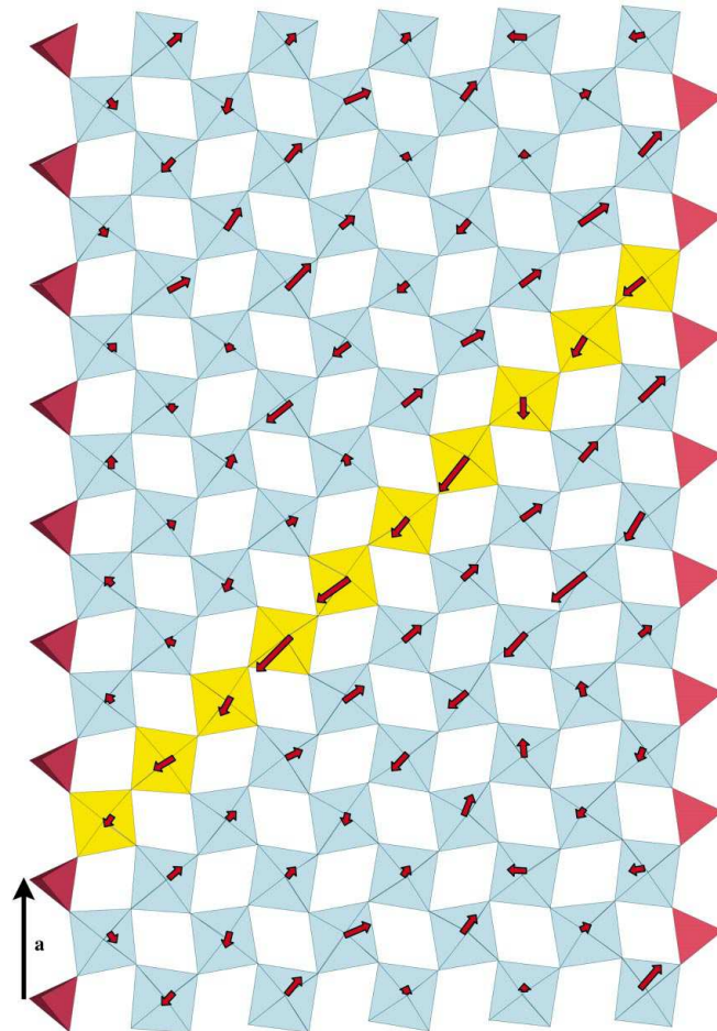
Figure 7 : Représentation structurale du terme m=10 à 293K [Roussel2000a]. Les déplacements des atomes de tungstène sont symbolisés par des flèches. Ceux-ci ont été multipliés par 10 pour mettre en évidence leur comportement type anti-ferro-électrique.
