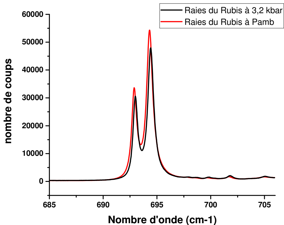
Figure 38 : Mesure de spectroscopie de fluorescence obtenue pour la première pression étudiée. Le déplacement des raies du rubis par rapport à celles mesurées à pression ambiante est clairement visible. Ce déplacement nous permet d'avoir accès à la valeur de la pression appliquée au sein de la cellule à enclumes de diamant via la formule ci-dessus.
