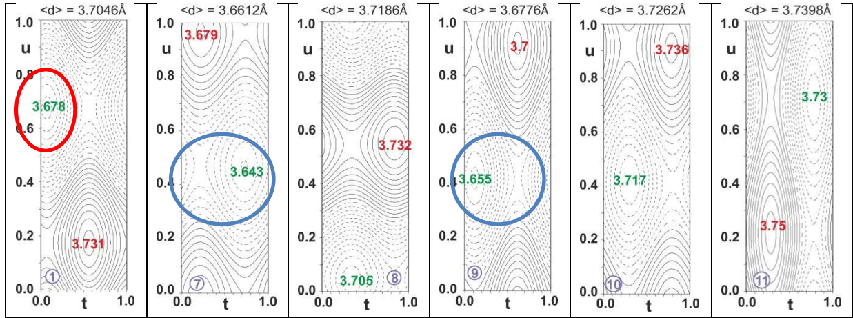
Figure 17: Carte 2d représentant l'évolution de l'écart par rapport à la distance moyenne (contours en pointillés : écart négatif ; contour plein : écart positif) pour la distance W1_2 - W_i en fonction des deux dimensions internes t et u . Les extrema sont donnés en vert et en rouge en Å.
