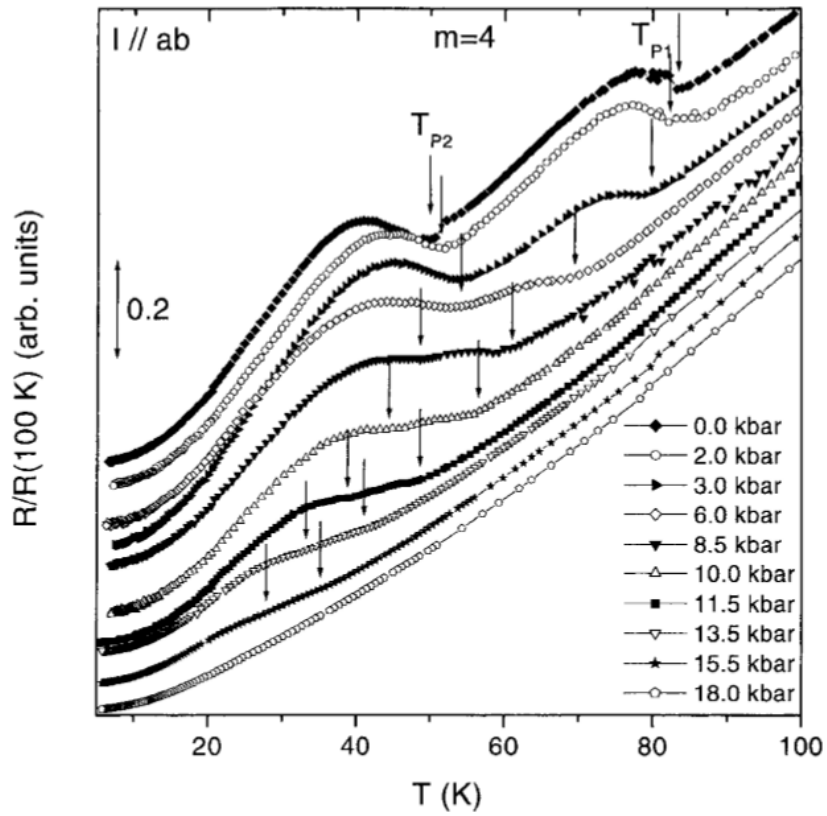
Figure 31 : Dépendance en température de la résistivité mesurée dans le plan ( ab ) d'un cristal de m=4 , normalisée à 100K, pour différentes valeurs de pression appliquée au cristal [Beille2001].
