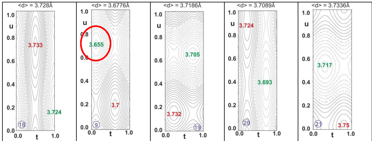
Figure 18: Carte 2d représentant l'évolution de l'écart par rapport à la distance moyenne (contours en pointillés : écart négatif ; contour plein : écart positif) pour la distance W2_1 - W_i en fonction des deux dimensions internes t et u . Les extrema sont donnés en vert et en rouge en Å.
