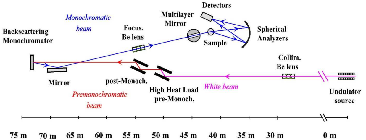
figure 18 : Schéma de la ligne ID28 de diffusion inélastique de l'ESRF [ESRF].
