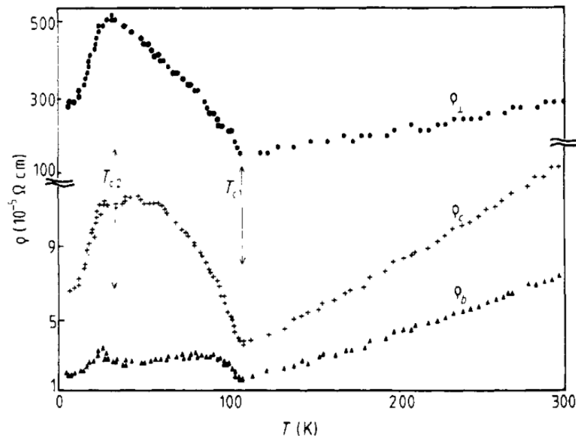
Figure 44 : Résistivité électrique du \eta - Mo_4O_{11} en fonction de la température pour les 3 orientations cristallographiques b , c et a au plan de la plaquette ( bc ) [Guyot1983].
