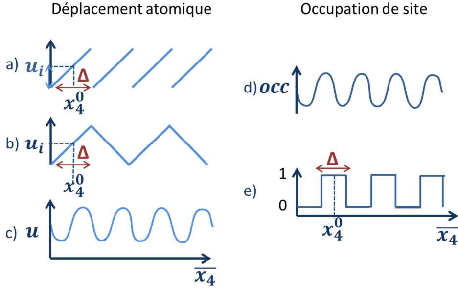
Figure 16 : Fonctions utilisées pour modéliser les déplacements atomiques (a, b et c) et les modulations d'occupation des super-atomes (d et e).
