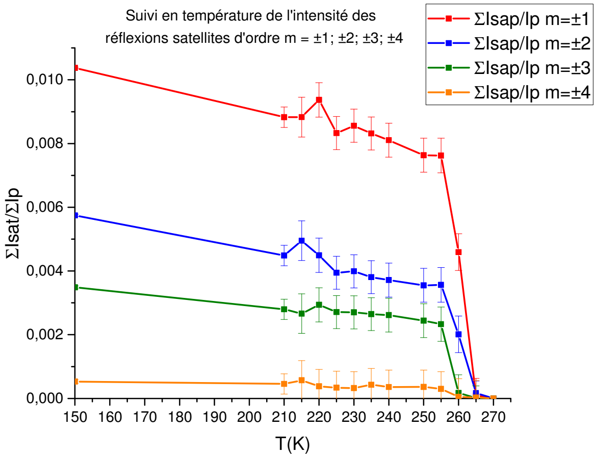
Figure 6 : Graphique représentant l'évolution du ratio de la somme des intensités des réflexions satellites sur la somme de l'intensité des réflexions principales, jusqu'au quatrième ordre, en fonction de la température du système. Les valeurs de \Sigma Isat/\Sigma Ip ont été calculées en moyennant \Sigma Isat(+m)/\Sigma Ip et \Sigma Isat(-m)/\Sigma Ip . Une extinction de l'intensité des réflexions satellites peut être mise en évidence aux alentours de la température de transition T=265K .
