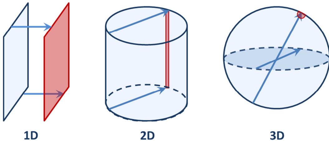
Figure 5 : Emboîtement de la Surface de Fermi pour des matériaux 1D, 2D et 3D idéaux. Les zones en rouges sont les zones susceptibles de subir un nesting.
