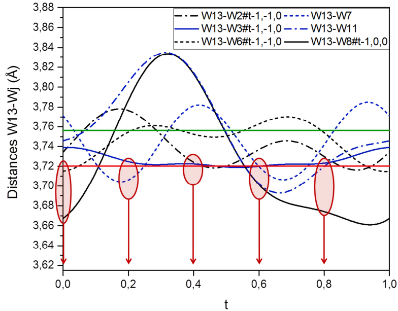
Figure 27 : Variations relatives des distances W13-W_j en fonction de t . Légende identique à la figure 26.
