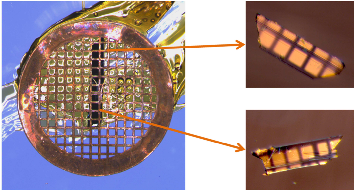
Figure 25 : Dépôt obtenu sur deux cristaux test en utilisant une grille de microscopie TEM de maillage 100 \times 100 \mu\text{m}^2 comme masque. La photo de la grille a été prise avec un grossissement \times 40 et les photos des cristaux avec un grossissement de \times 120 .
