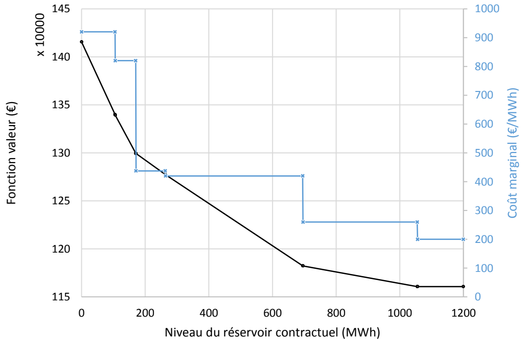
Figure 6. Courbe de coût marginal et fonction valeur des effacements type load-shedding
