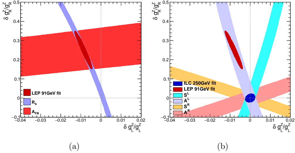
Figure C.15: Les régions de \pm 1\sigma sur les couplages Z^0 b \bar{b} définies par l'asymétrie avant-arrière et les mesures des sections efficaces totales au LEP (a) et à l'ILC via l'ajustement de la section transversale différentielle (b). Les lignes directrices détaillées montrent la valeur modèle standard. Quant à l'ILC les bandes d'erreurs se chevauchent aux valeurs des couplages attendues par le Modèle standard.
