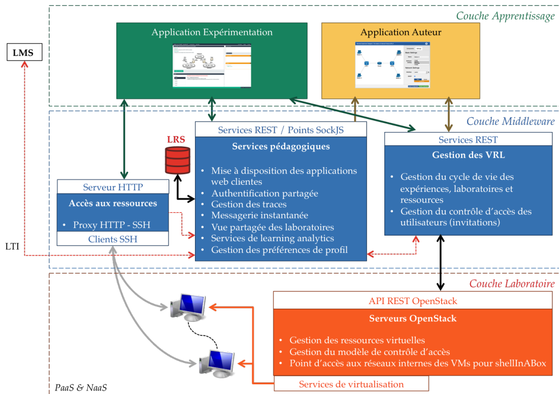
Figure 4.3 – Architecture conceptuelle de Lab4CE
