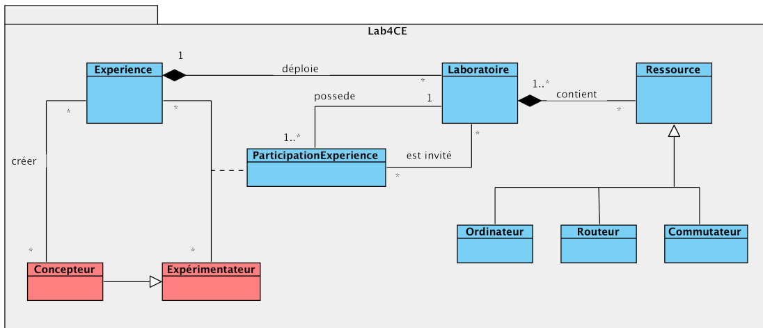
Figure 4.2 – Diagramme de classes général de Lab4CE
