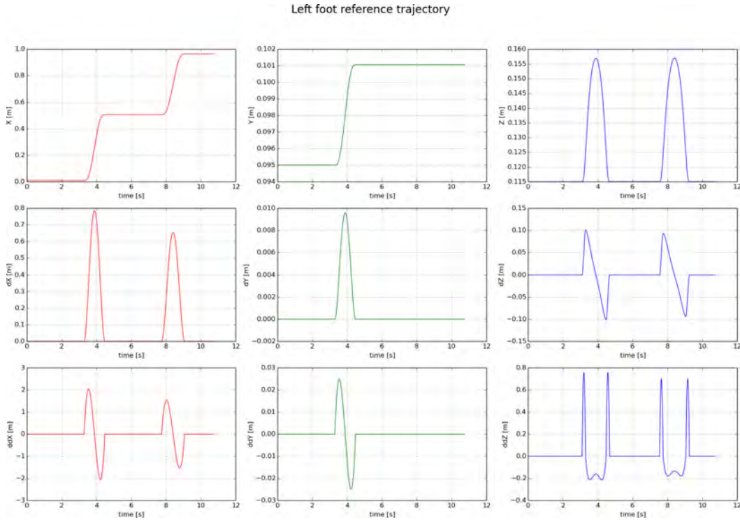
FIGURE 6.7 – Exemples de trajectoires par défaut, pour deux pas sur sol plat. Les lignes sont (de haut en bas) la position, la vitesse et l'accélération de l'organe terminale et les colonnes sont (de gauche à droite) les axes x, y, z .
