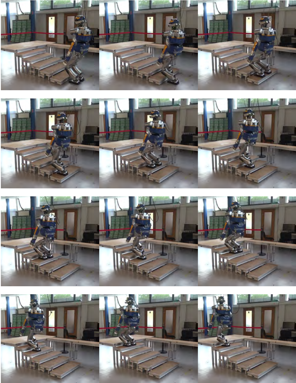
FIGURE 7.11 – Captures du mouvement corps complet réalisé par le robot HRP-2 pour le scénario de la montée des marches.
