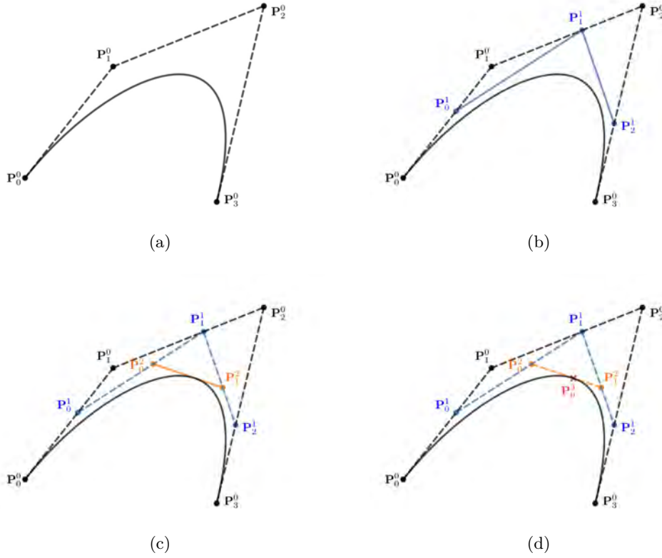
FIGURE A.1 – Itérations successives de l'algorithme de De Casteljau pour une courbe de Bézier de degré n = 3 définie par les points de contrôle \mathbf{P}_i^0 , évaluée à u_0 = 0.6 .
