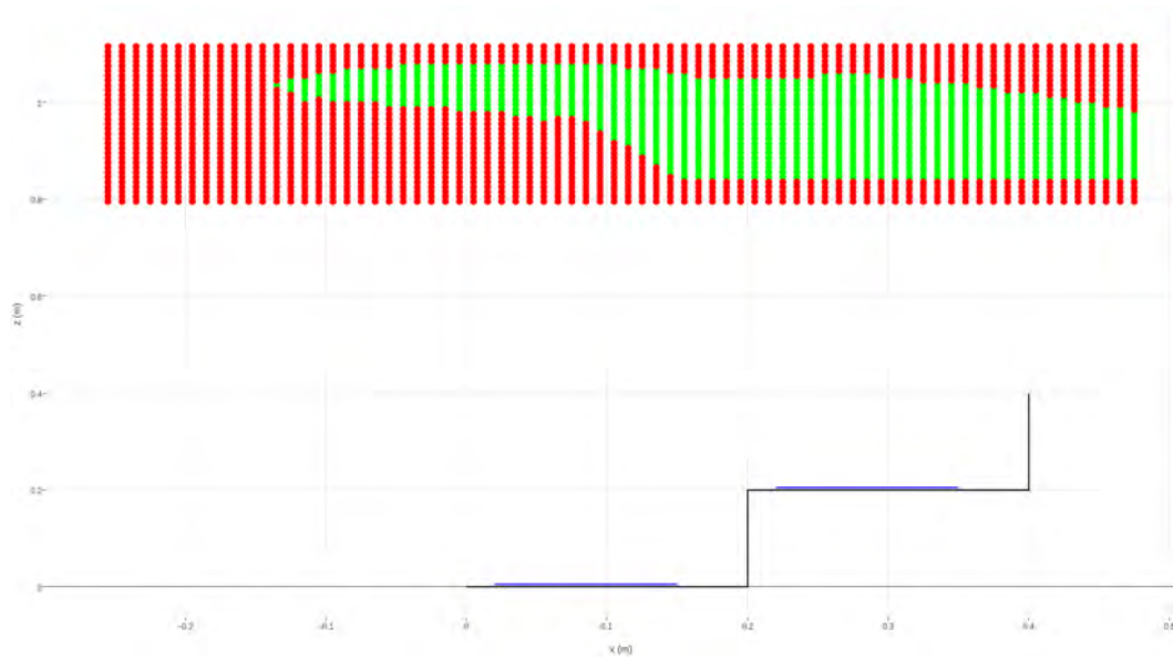
(a) Existence d'une configuration cinématiquement valide
