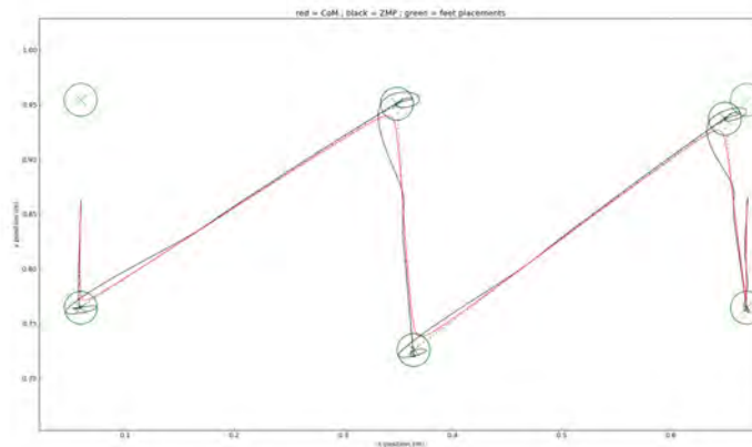
FIGURE 7.10 – Trajectoire centroïdale (en rouge) et trajectoire du ZMP (en noir) générée pour la montée de deux marches de 10cm de hauteur et de 30cm de profondeur. En vert les positions des contacts.
