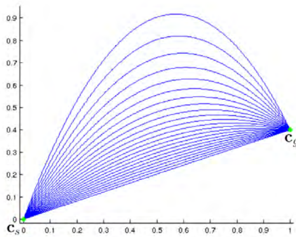
FIGURE 1.4 – Figure extraite de [Campana 2016b]. Faisceau de paraboles connectant \mathbf{c}_s et \mathbf{c}_g (points verts), pour différentes valeurs de \alpha_s , dans le plan \pi_\theta .
