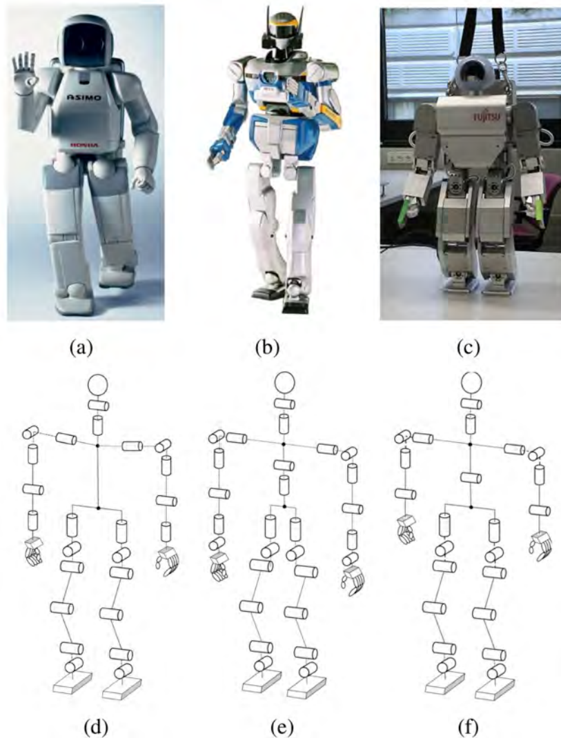
FIGURE 8 – Figure extraite de [Ali 2010]. Exemple de trois robots et des chaînes cinématiques les composant. (a) le robot ASIMO et sa chaîne cinématique (d). (b) le robot HRP-2 et sa chaîne cinématique (e). (c) le robot HOAP-2 et sa chaîne cinématique (f).
