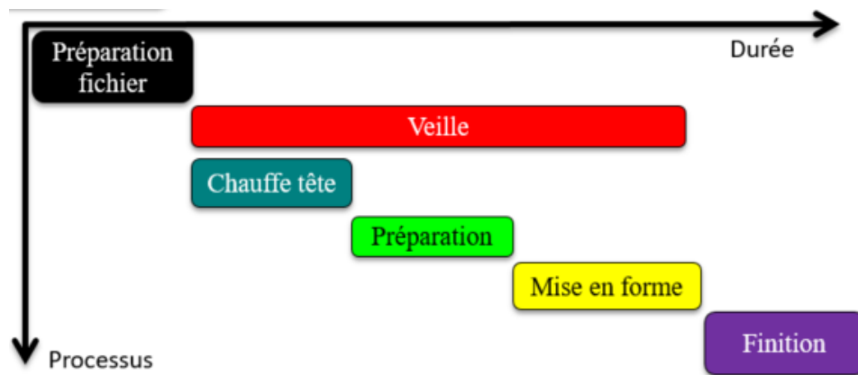
Figure B.2 - Agencement des différentes phases de fabrication pour l'objet260 connex
