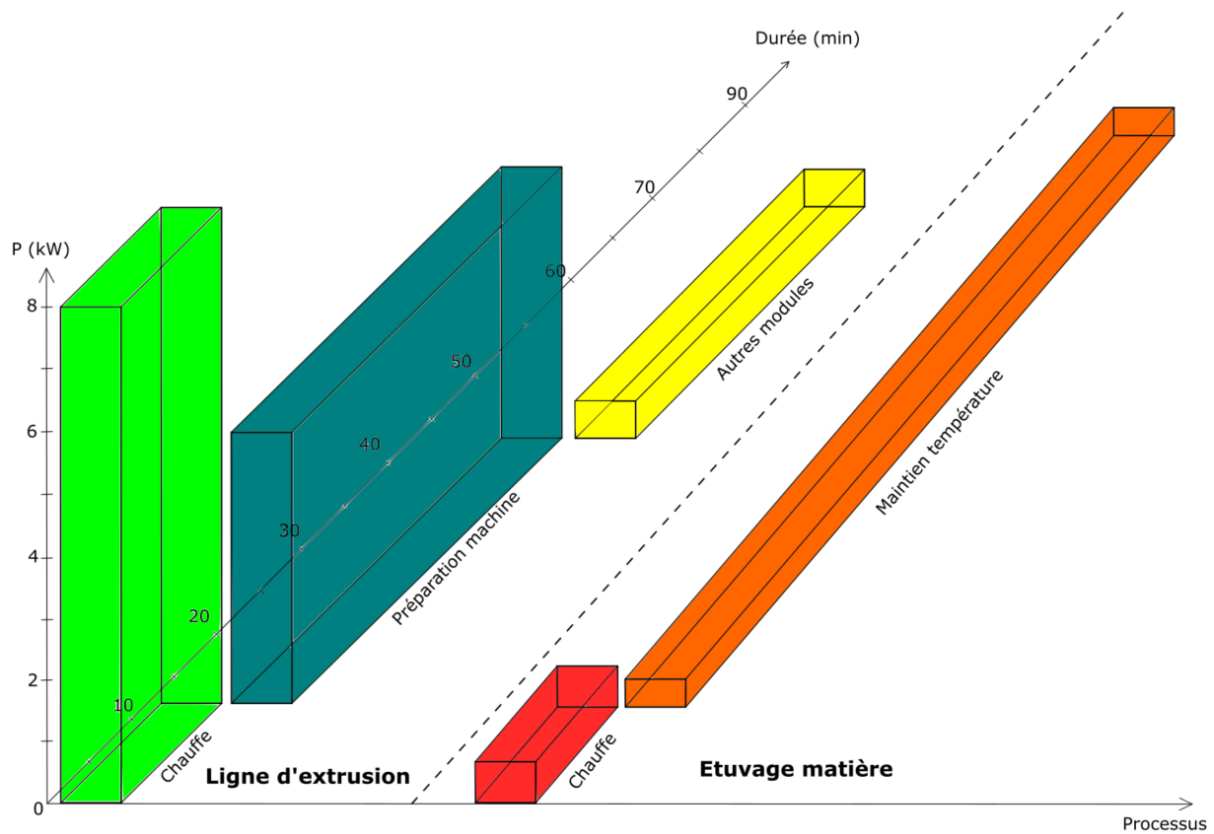
Figure 4.8 - Puissance moyenne et durée des phases de fabrication de la ligne d'extrusion pour la mise en fil d'1 kg d'ABS
