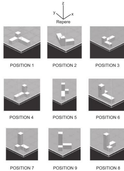
Figure 2.5 - Les différentes orientations de la pièce étudiée (Mognol2006)
