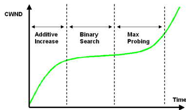
(a) Fonction d'accroissement de la fenêtre de congestion chez BIC-TCP . (Source : [NCSUNRL]).
