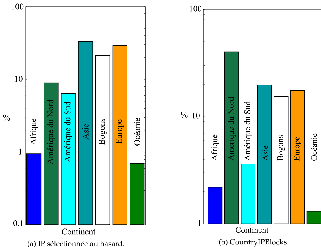
FIGURE 2.2 – Distribution géographique des adresses IPv4 publiques.
