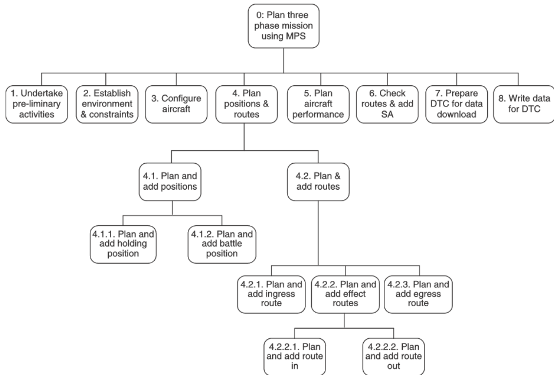
FIGURE 2.7 – Exemple d'un modèle HTA
