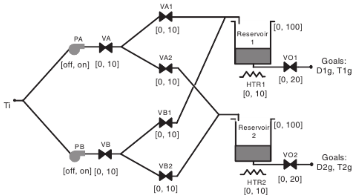
FIGURE 2.1 – Représentation schématique du système DURESS II [113]
