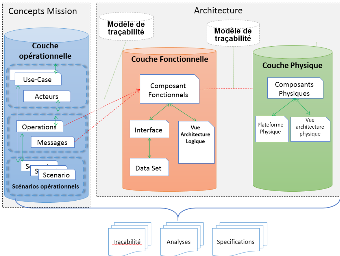
FIGURE 1.1 – Modèle MBSE générique utilisé pour NECTAR
