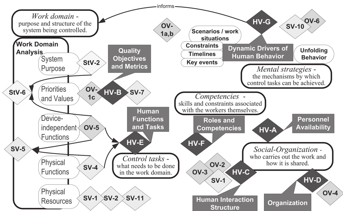
FIGURE 3.5 – Relations entre les Human Views , le CWA et les vues du Mo-DAF [21]
