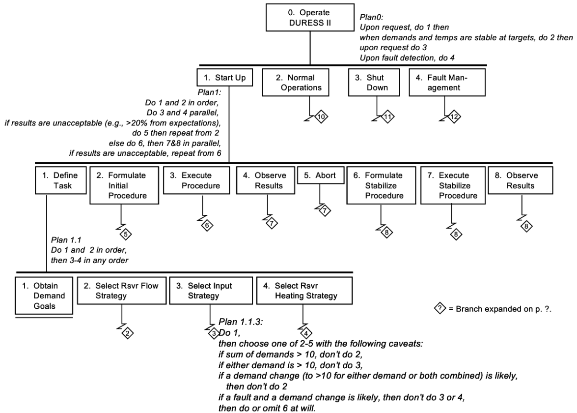
FIGURE 2.7 – Modèle HTA de DURESS II [40]
