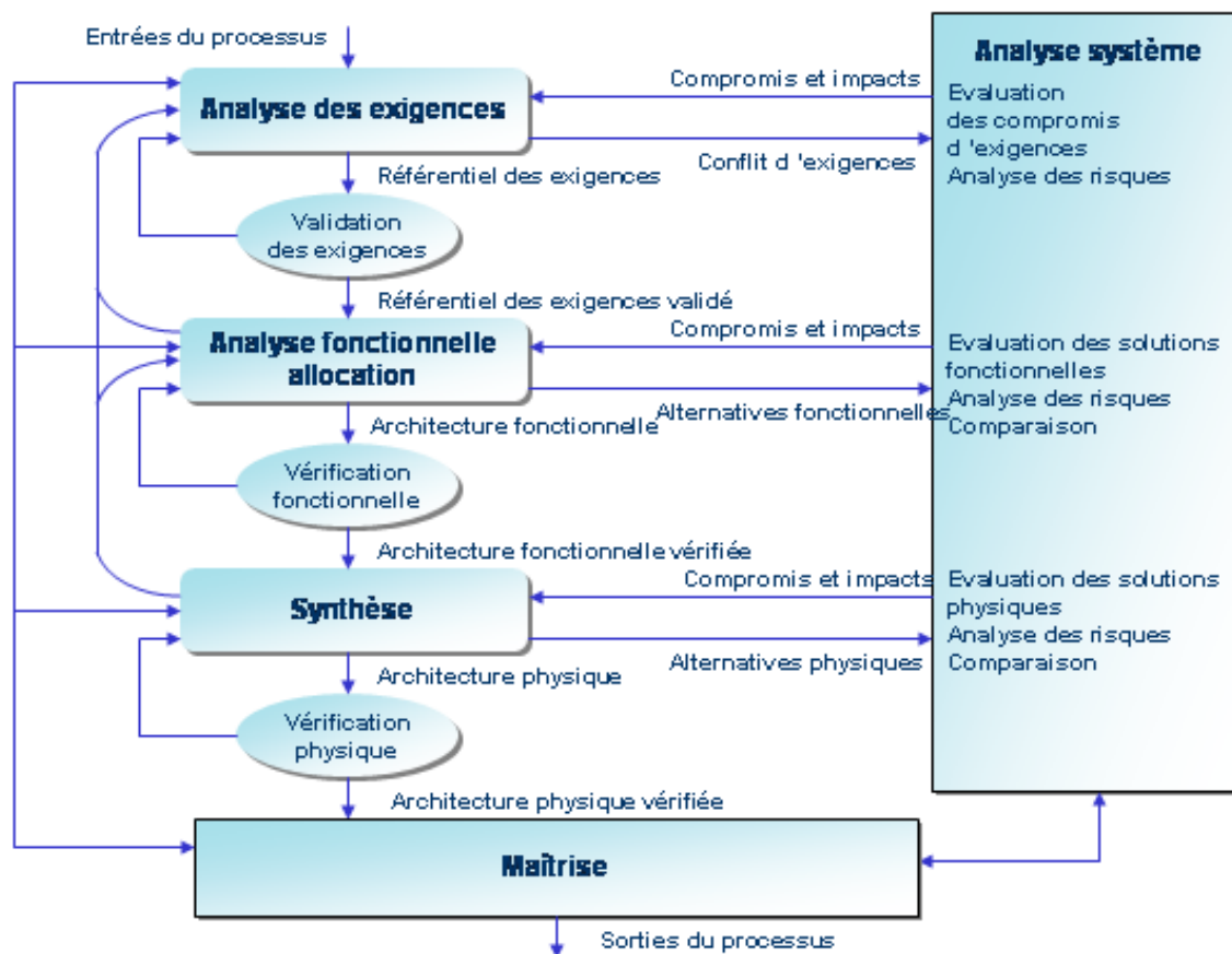
FIGURE 1.7 – Processus de la norme IEEE 1220 [5]
