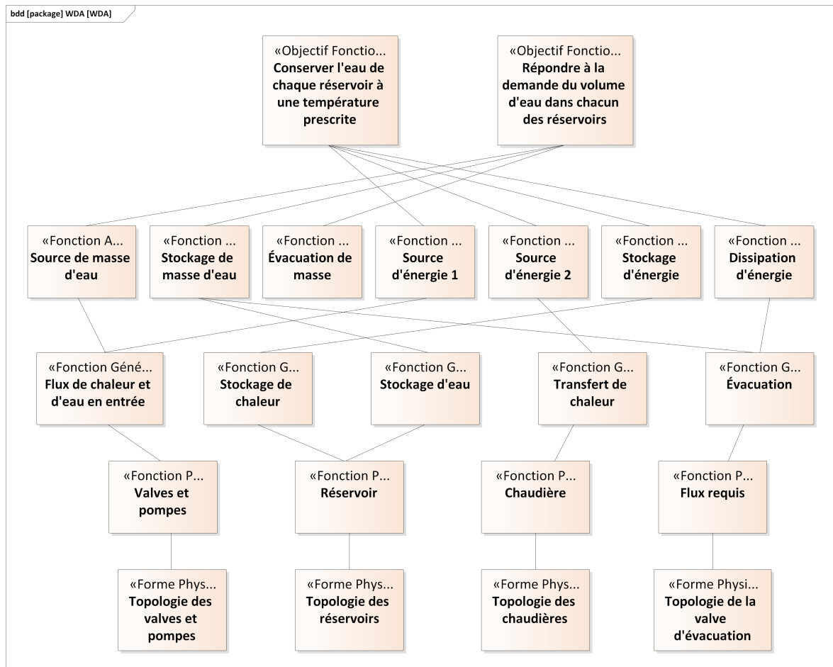
FIGURE 2.4 – Hiérarchie d'abstraction modélisée en SysML
