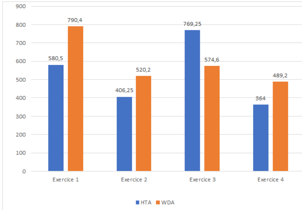
FIGURE 1.3 – Moyenne de temps de réalisation des exercices (en secondes)
