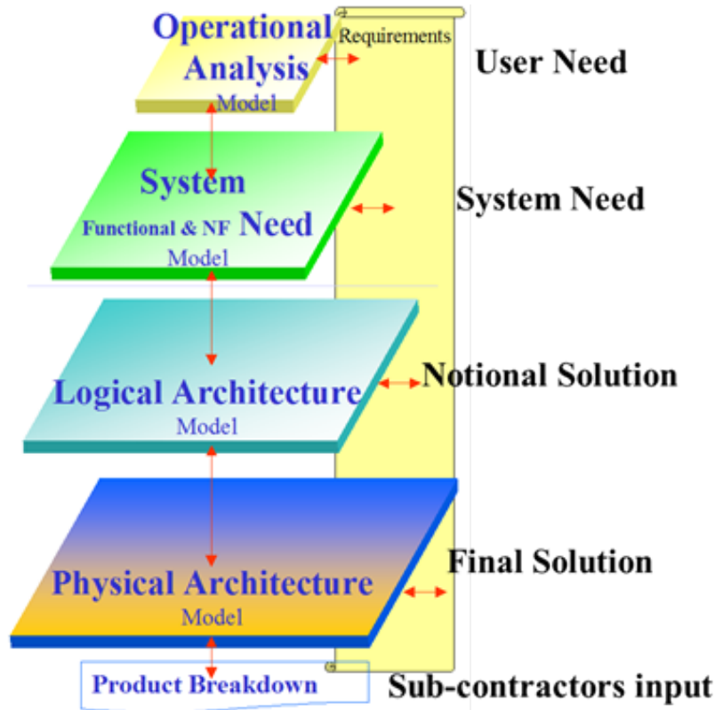
FIGURE 1.11 – Démarche de la méthodologie ARCADIA [98]
