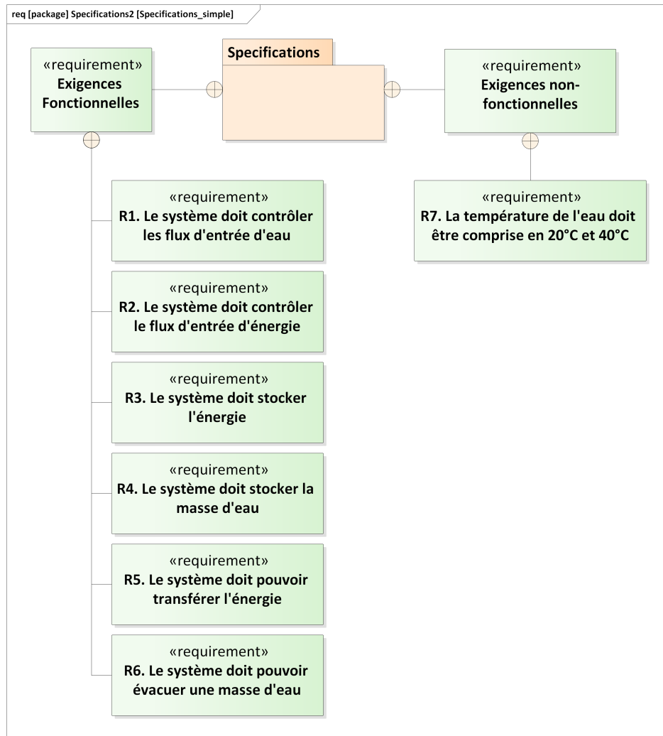
FIGURE 2.5 – Diagramme d'exigences du système DURESS II
