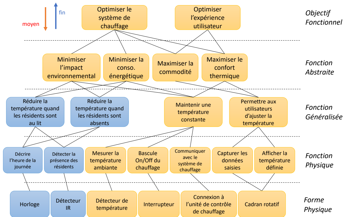
FIGURE 1.3 – Hiérarchie d'abstraction modifiée du thermostat [61]
