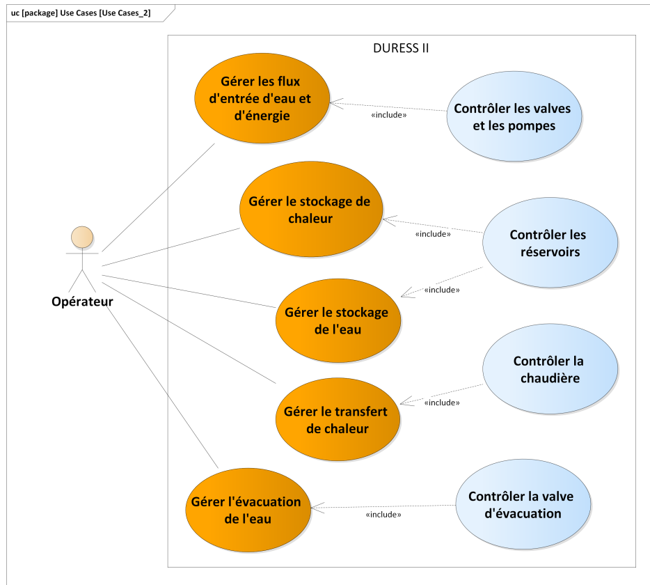
FIGURE 2.6 – Diagramme de cas d'utilisation pour le système DURESS II
