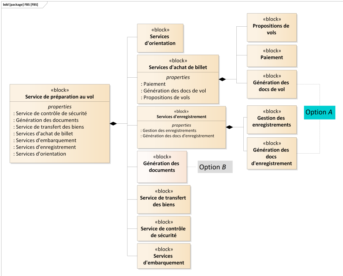
FIGURE 1.13 – Modèle FBS
