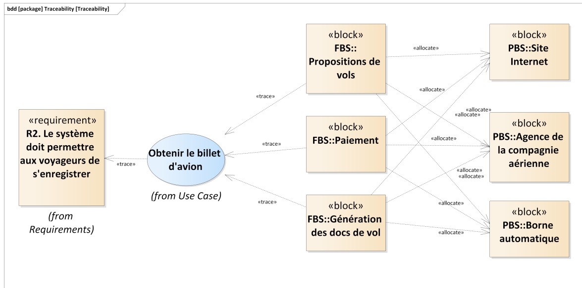
FIGURE 1.17 – Modèle de traçabilité pour l'exigence liée à l'achat de billet
