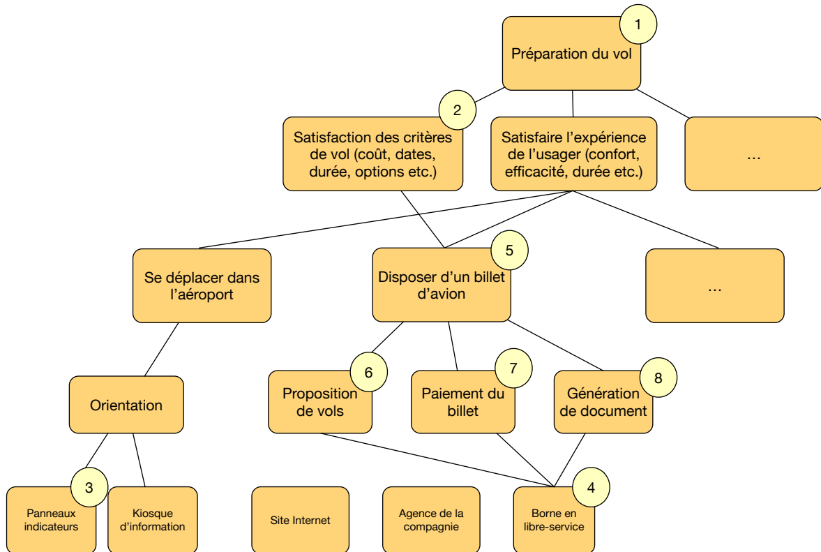
FIGURE 1.9 – Parcours de la hiérarchie d'abstraction
