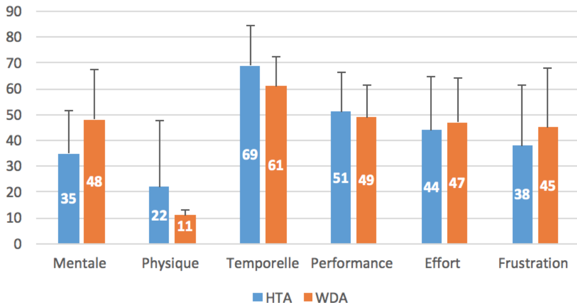
FIGURE 1.8 – Comparaison des résultats du test NASA-TLX
