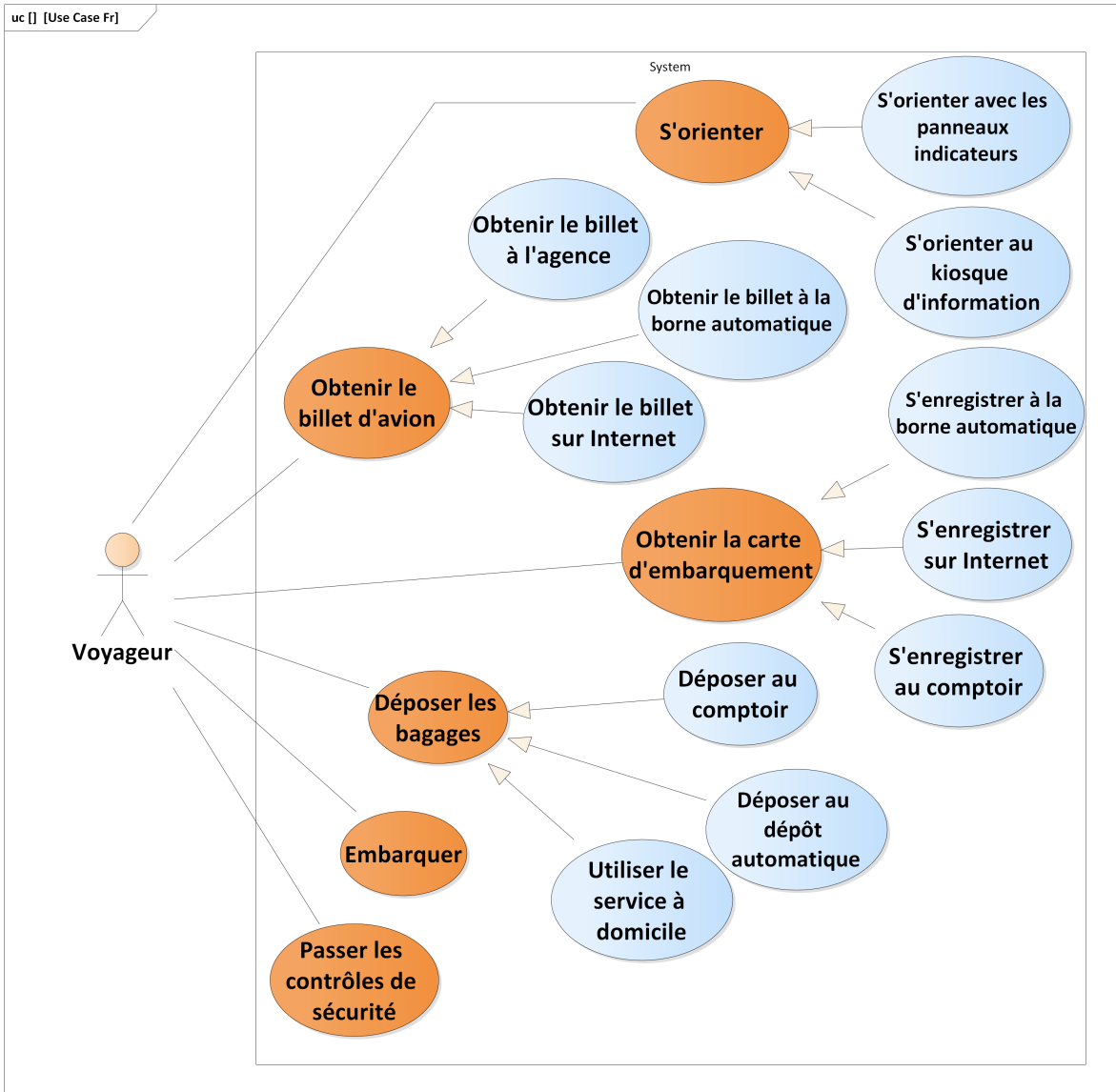
FIGURE 1.8 – Cas d'utilisation de NECTAR
