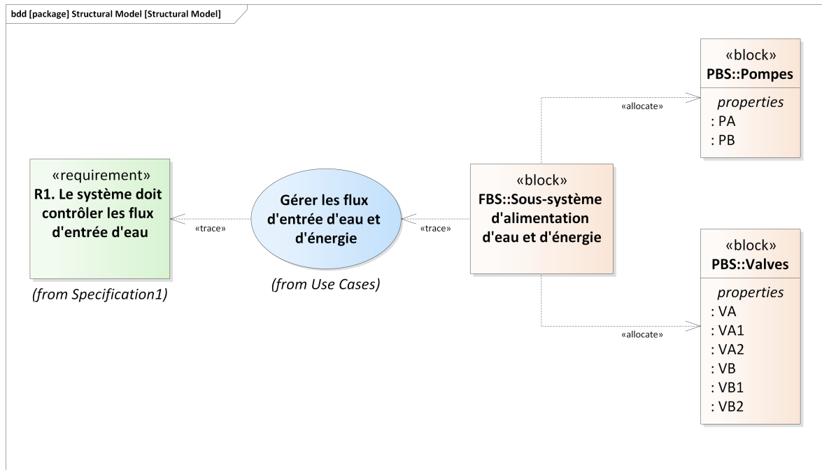
FIGURE 2.14 – Modèle de traçabilité pour l'alimentation du système
