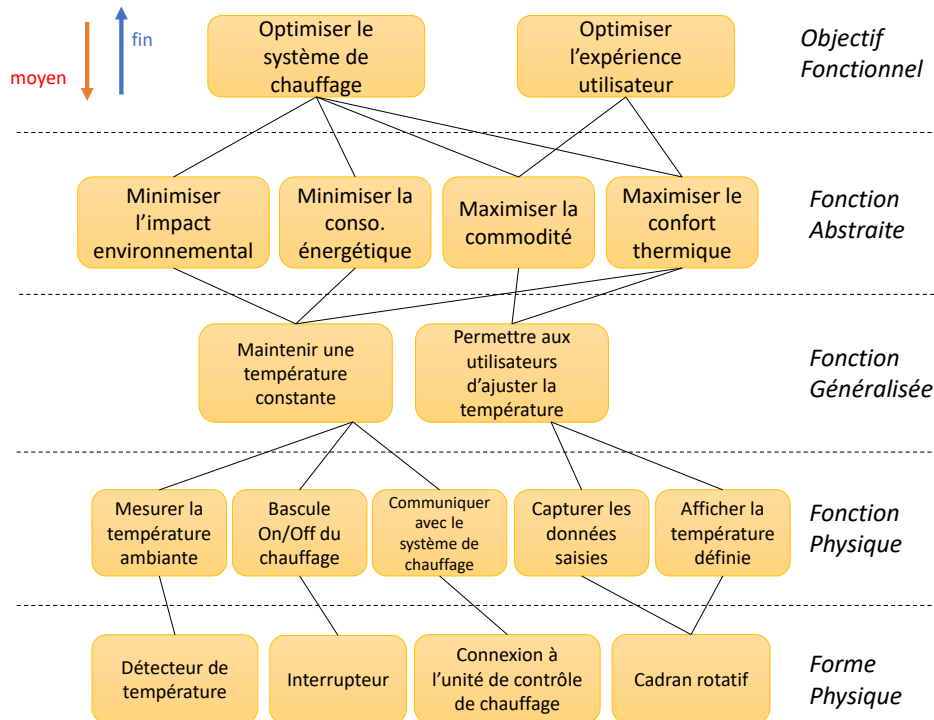
FIGURE 3.2 – Hiérarchie d'abstraction d'un thermostat [61]
