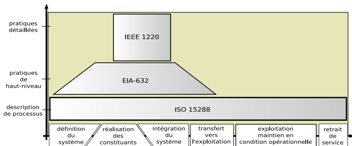
FIGURE 1.9 – Niveaux de détails des normes [35, 96]
