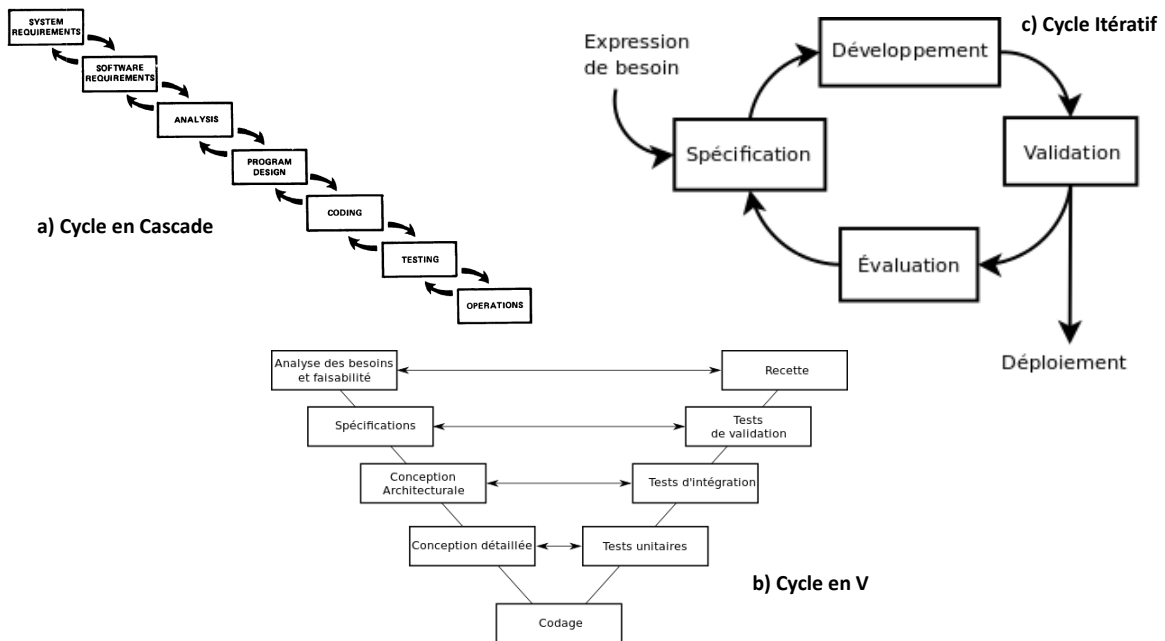
FIGURE 1.3 – Modèles de cycle de vie
