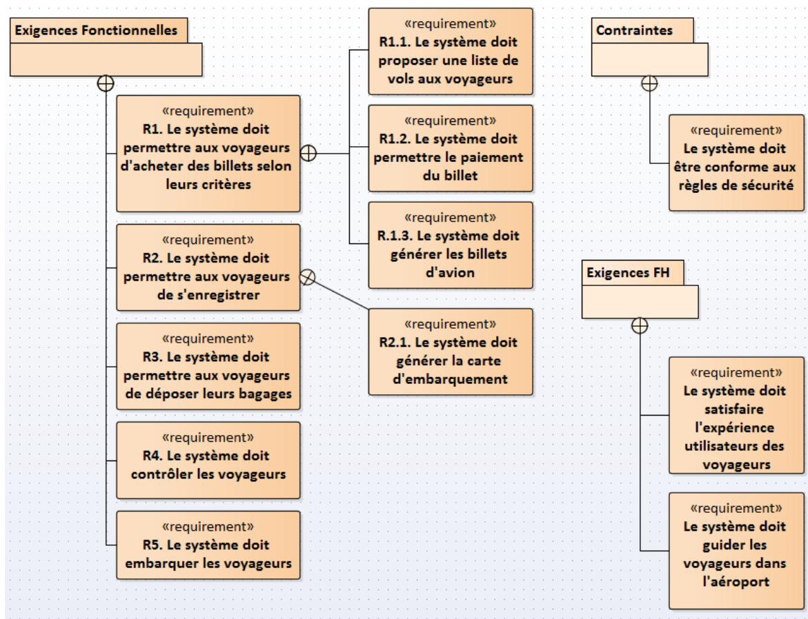
FIGURE 1.7 – Modélisation des exigences
