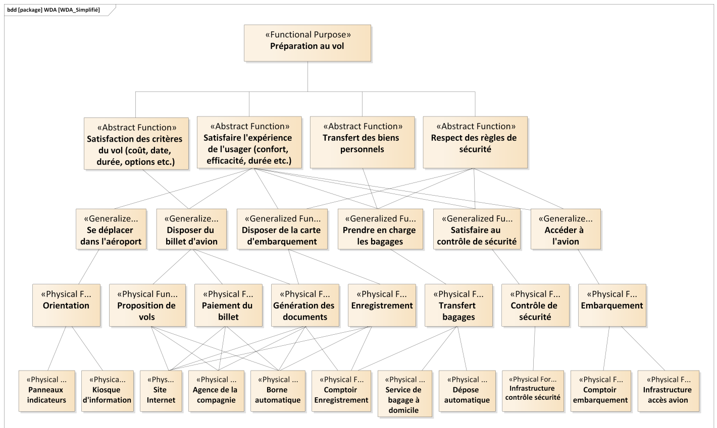
FIGURE 1.6 – Modélisation en SysML de la hiérarchie d'abstraction
