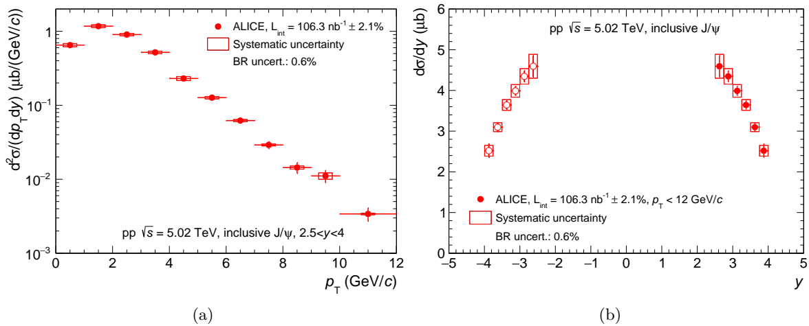
Figure 9.1: Section efficace inclusive de J/\psi différentielle en fonction de (a) p_{\text{T}} et (b) y dans des collisions pp à \sqrt{s} = 5.02 TeV [73].
