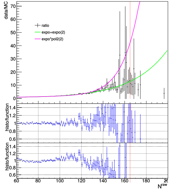
(b) DPMJET Pb-p
