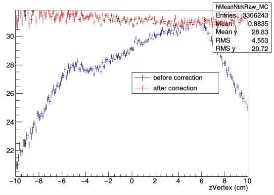
(d) EPOS Pb-p
