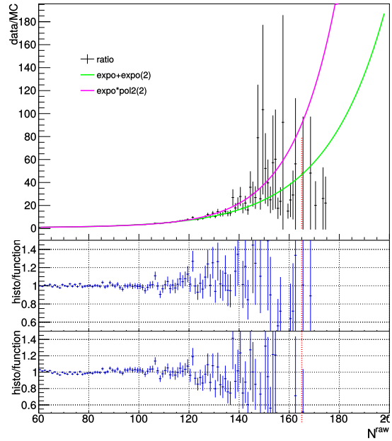
(d) EPOS Pb-p
