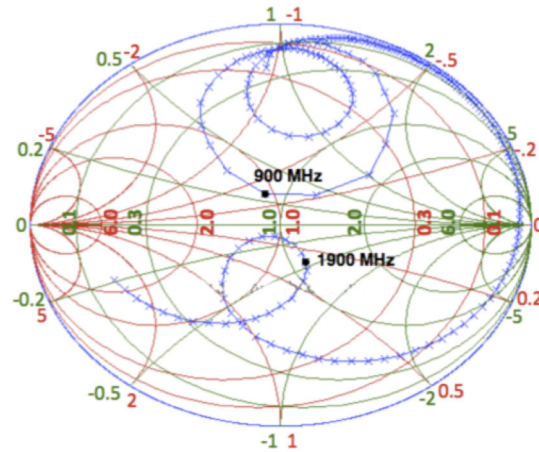
FIGURE 4.32 – Coefficient de réflexion en entrée d'un circuit adapté à 900 et 1900 MHz.
