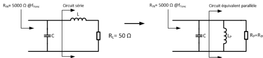
FIGURE 4.19 – Exemple de réseau en L élévateur d'impédance.
