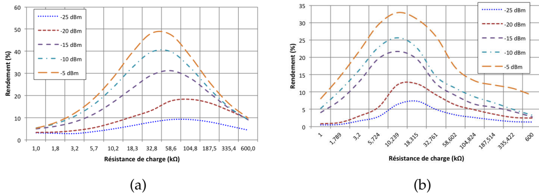
FIGURE 3.30 – Rendement de conversion en fonction de la charge pour différents niveaux de puissance d'entrée à 900 MHz (a) et 2,4 GHz (b) en simulation EM.
