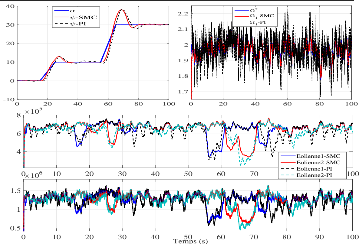
FIGURE 4.11 : Scénario 3. - Haut-gauche - Angle d'orientation \psi ( ^{\circ} ) en fonction du temps ( sec ). Haut-droite - Suivi de la vitesse de rotation \Omega_1 ( rad/s ) en fonction du temps ( sec ). Milieu - Couple électromagnétiques \Gamma_{em1} et \Gamma_{em2} ( N.m ) en fonction du temps ( sec ). Bas - Puissances générées pour l'éolienne 1 et l'éolienne 2 ( W ) en fonction du temps ( sec ).
