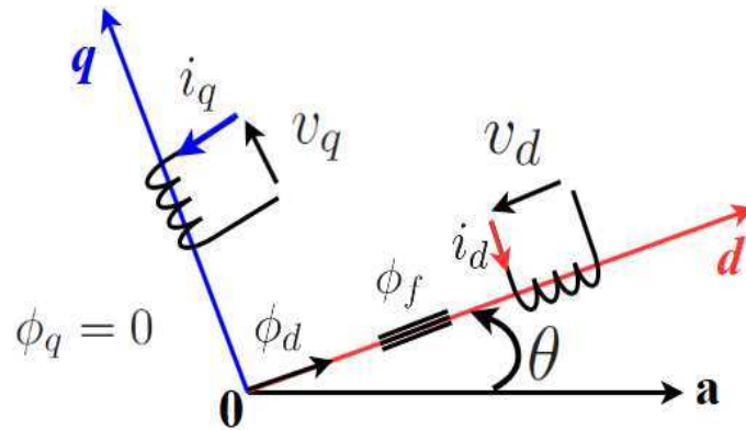
FIGURE 3.8 : Principe de l'orientation du flux [27].
