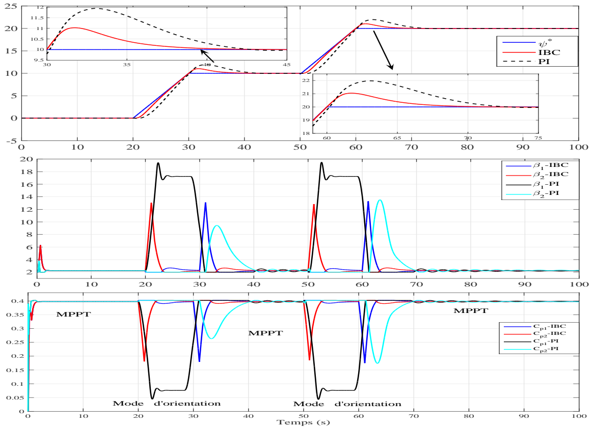
FIGURE 4.21 : Scénario 2. - Haut : angle d'orientation \psi ( ^\circ ) en fonction du temps ( sec ). Milieu : angles de calage \beta_1 et \beta_2 ( ^\circ ) en fonction du temps ( sec ). Bas : Coefficient de puissance C_{p1} et C_{p2} en fonction du temps ( sec ).
