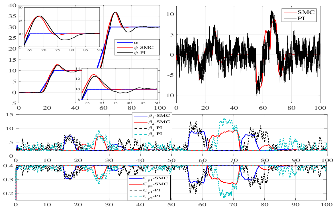
FIGURE 4.9 : Scénario 2-Haut-gauche - Angle d'orientation \psi ( ^\circ ) en fonction du temps ( sec ) . Haut-droite - Entrée de commande \Delta\beta ( ^\circ ) en fonction du temps ( sec ). Milieu - Angles de calages \beta_1 et \beta_2 ( ^\circ ) en fonction du temps ( sec ). Bas - Coefficients de puissance C_{p1} et C_{p2} en fonction du temps ( sec ).
