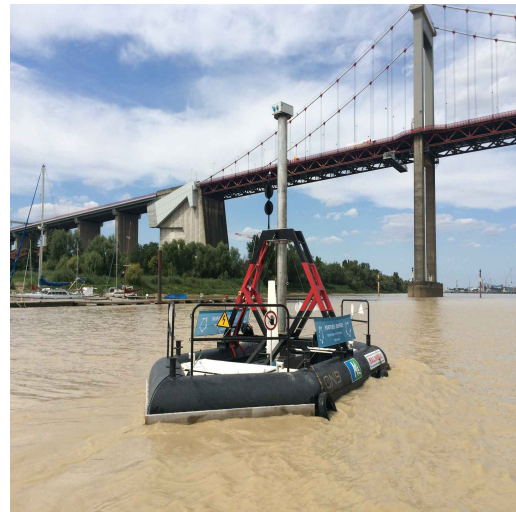
Hydrolienne flottante
