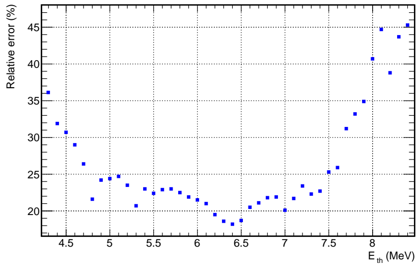
Figure 5 – Incertitude sur le taux de {}^9\text{Li} .
