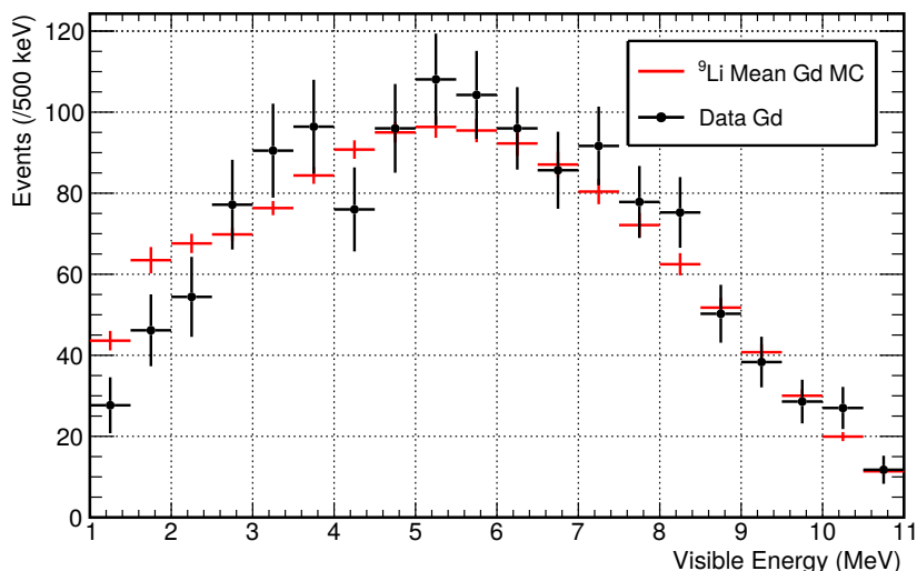
Figure 2 – Ajustement sur les données gadolinium.
