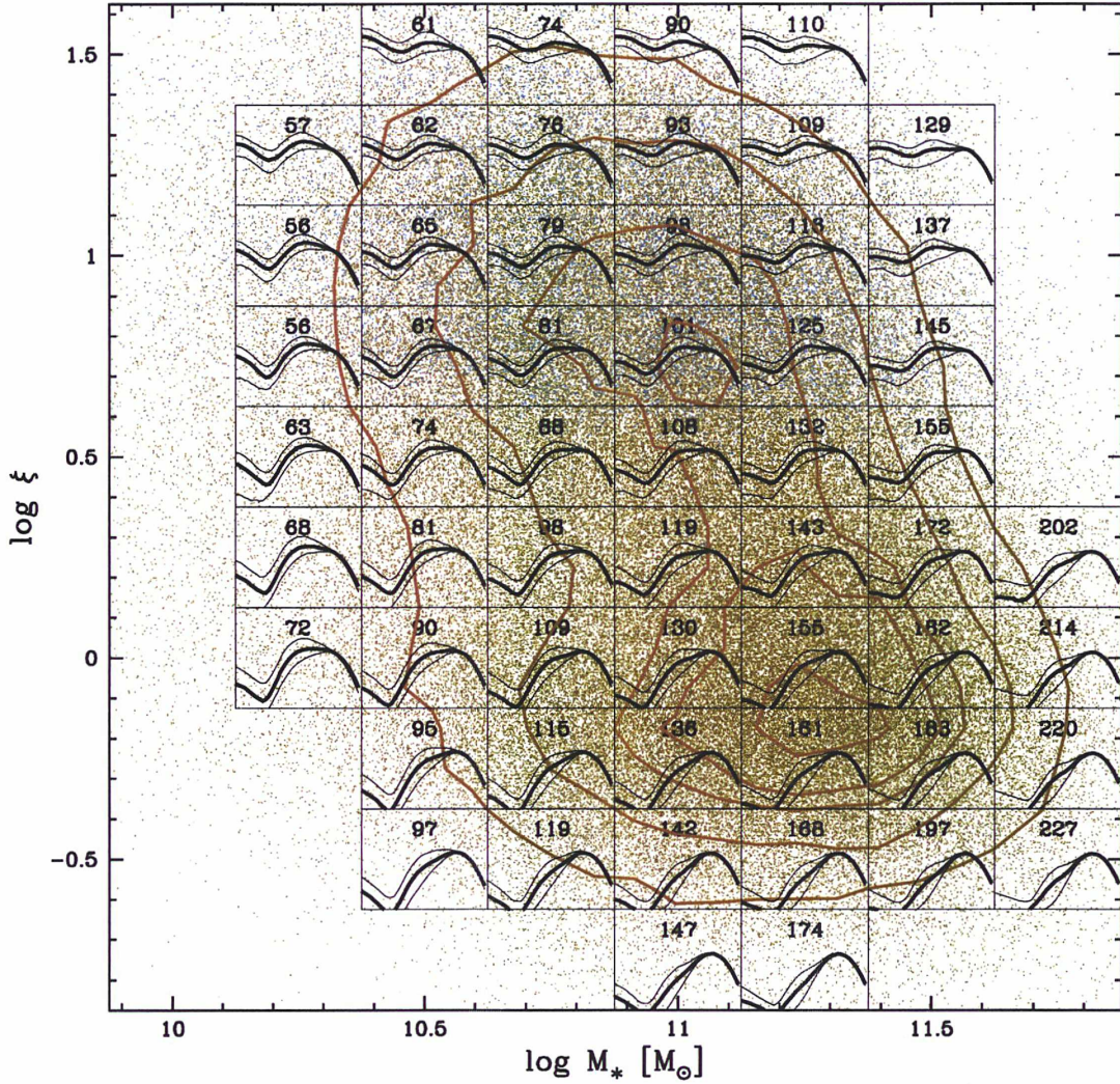
Figura 7.4: Diagrama M_* contra \xi \equiv L(\text{H}\alpha)_{\text{obs}}/[L(\text{H}\alpha)_{\text{exp}}(t > 10^8\text{yr})] para galáxias classificadas como hospedeiras de AGN no diagrama W_{\text{H}\alpha} vs. [\text{N II}]/\text{H}\alpha (critério S06 da figura 8c de Cid Fernandes et al. 2010). As Seyferts ( W_{\text{H}\alpha} > 6 \text{ \AA} ) são representadas por pontos azuis. Cada caixa mostra as curvas para 16, 50 e 84% da distribuição de \text{SSFR}(t) . A escala das abscissas vai de \log t/\text{yr} = 6.5 a 10.5 e a das ordenadas \log \text{SSFR}/\text{yr}^{-1} = -12 a -9 . Os números nas caixas são a mediana da dispersão de velocidades em km/s, usualmente tomada como indicador da massa do buraco negro em AGNs. \xi = 1 indica que todos os fótons \text{H}\alpha podem ser explicados pela ionização por populações velhas. Note como a distribuição é bimodal e a separação ocorre em \xi \sim 1 . Figura por Cid Fernandes et al. (2009b).
