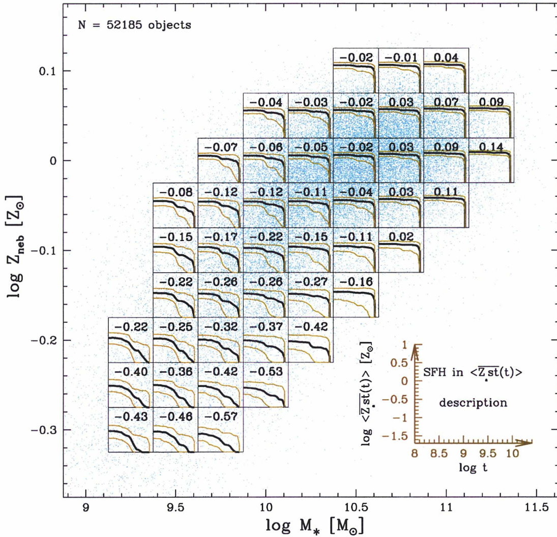
Figura 7.12: Como a Figura 7.5, mas para a evolução da metalicidade estelar \overline{Z}_{\star}(t_{\star}) dada pela Equação 3.3. Os números em cada caixa indicam a mediana da metalicidade estelar média ponderada pela massa (em \log Z_{\odot} ). A evolução química é bem mais rápida quanto mais perto da ponta superior da relação M_{\star} - Z_{\text{neb}} .
