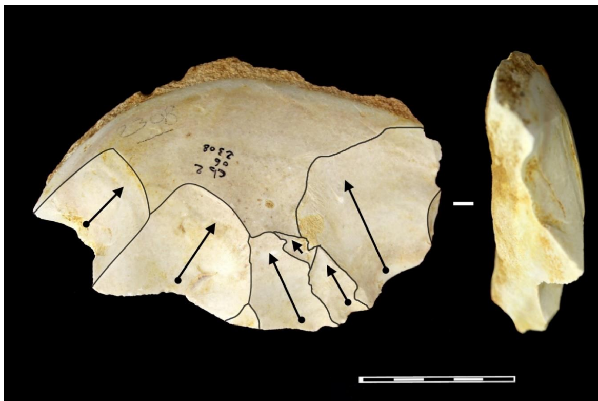
Figure 328 – Débitage Kombewa récurrent, unipolaire depuis la partie proximale de l'éclat-matrice.
