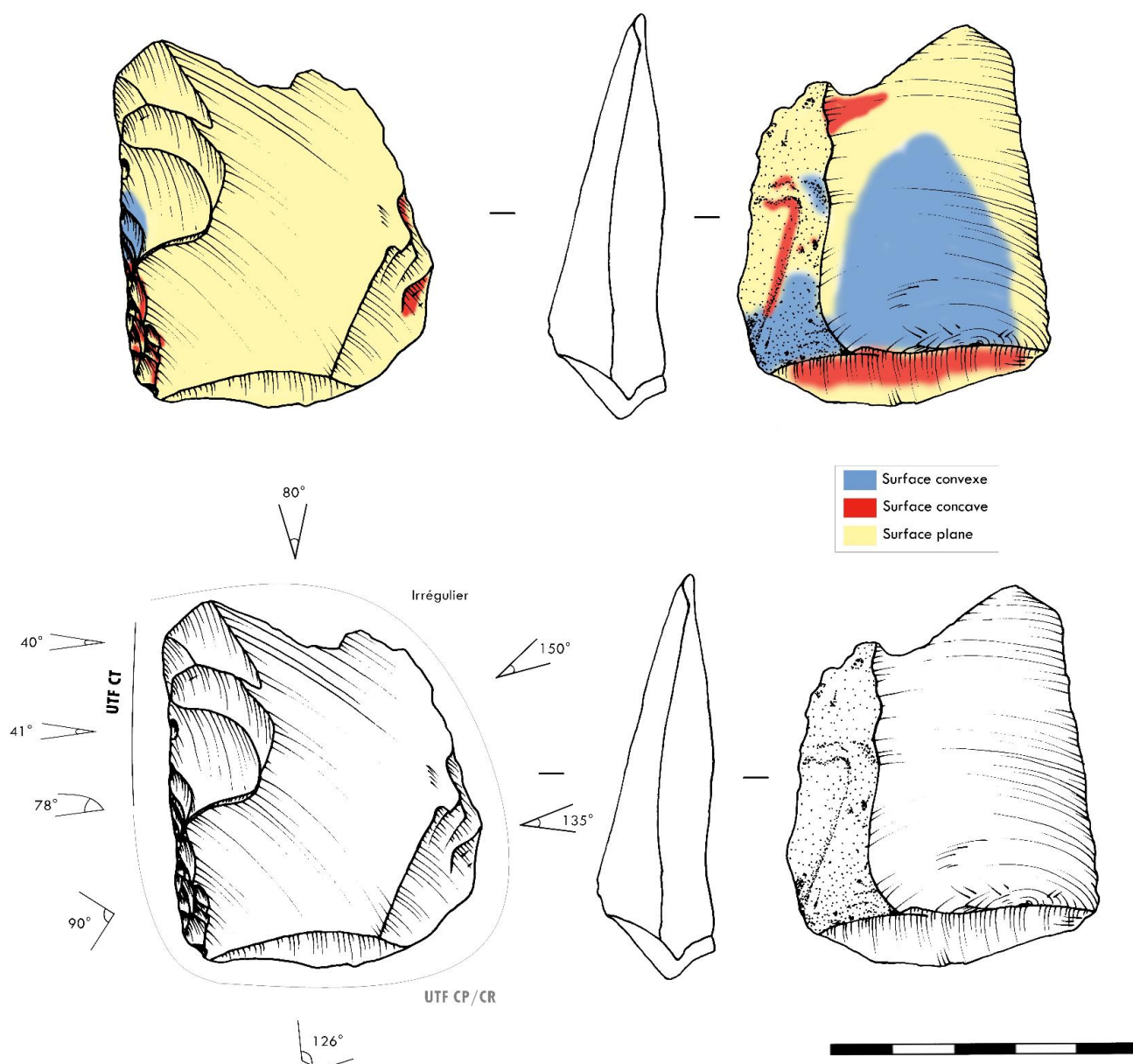
Figure 223 – Morphologie des surfaces et localisation de l'Unité-Techno-Fonctionnelle de Contact Transformatif de type Bord Linéaire Rectiligne (MIC86-O25-701).
