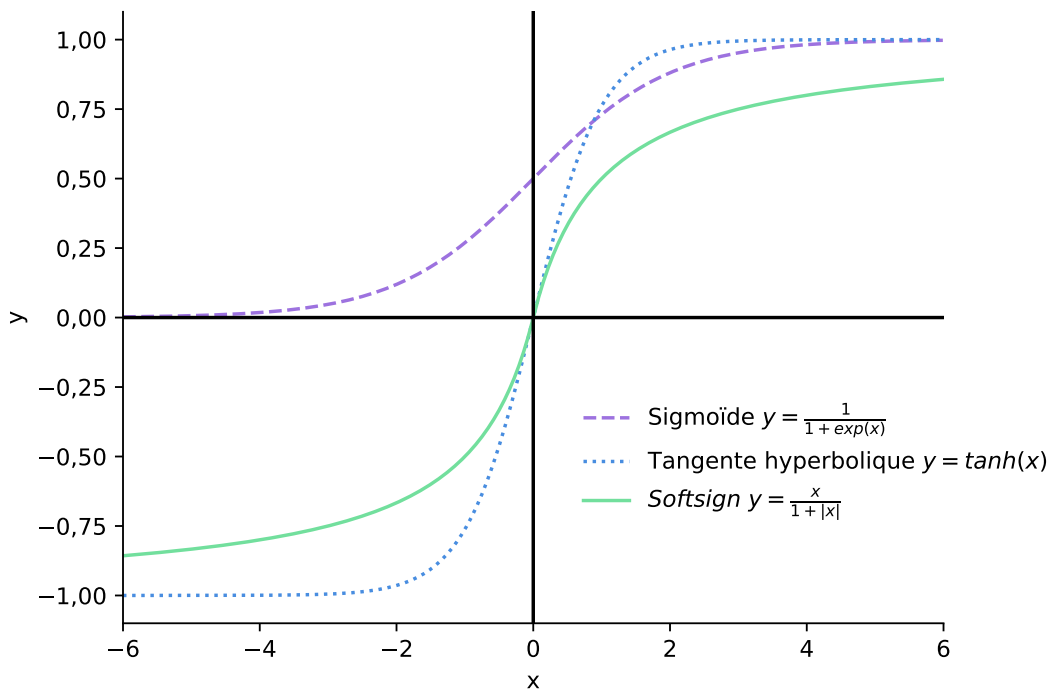
FIGURE 4.3 – Présentation de trois fonctions non-linéaires couramment utilisées par les perceptrons.
