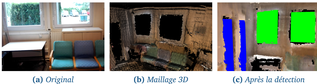
Figure 3.7 – Illustration du processus de reconstruction et de détection de la structure d'un bâtiment, de la construction du maillage la détection des ouvrants.
