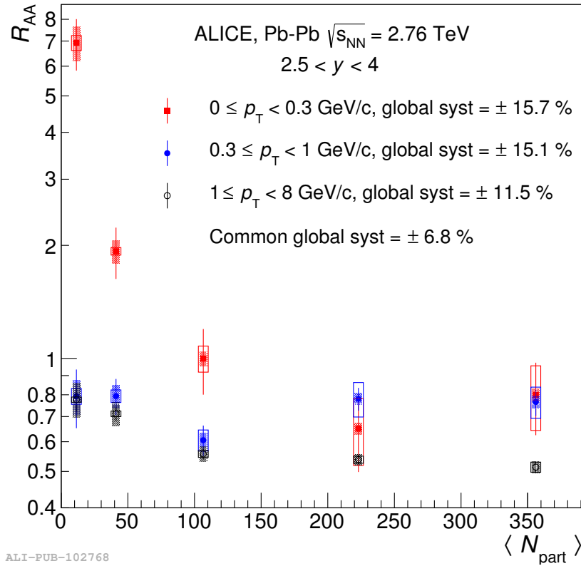
FIGURE 1.20 – R_{AA} en fonction de \langle N_{part} \rangle pour plusieurs intervalles en p_T mesuré par ALICE dans les collisions Pb–Pb à \sqrt{s_{NN}} = 2.76 TeV.
