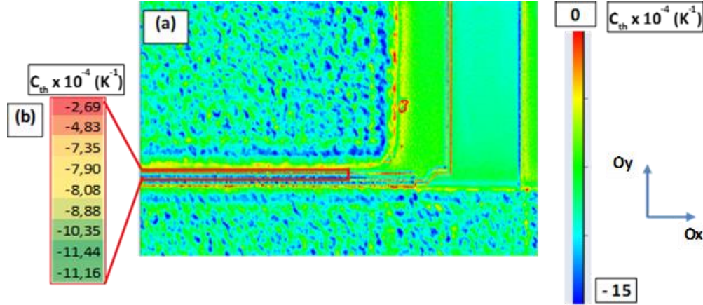
Figure II-9 : (a) Cartographie du coefficient de thermoréfectance sur la région 6 ; la plaque de champ est encadrée en rouge et compte 9 \times 500 pixels ( \lambda = 530 \text{ nm} ). (b) Moyennes des 500 valeurs de C_{th} obtenues sur chacune des 9 lignes de la plaque de champ.
