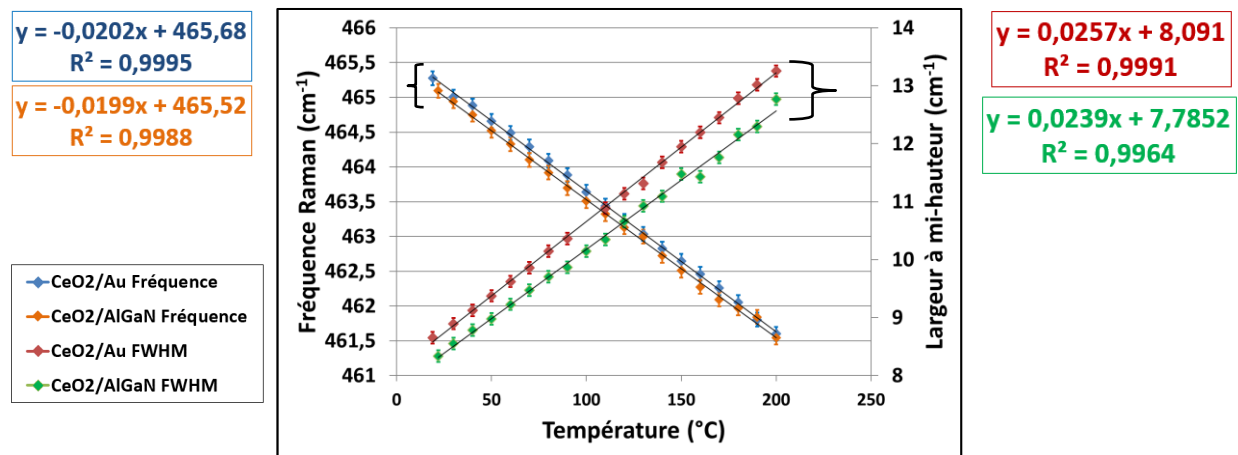
Figure III-32 : Courbes de calibration en température de \delta et \Gamma de particules de \text{CeO}_2 déposées sur de l'or (points bleus et rouges) et sur une couche d'AlGaIn/GaN sur un substrat de saphir (points jaunes et verts).
