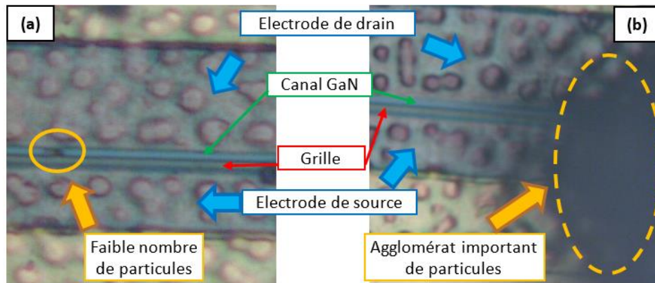
Figure III-33 : Micrographies du composant après saupoudrage du \text{CeO}_2 . Les cercles jaunes représentent les zones montrant (a) un faible amas et (b) un amas important à la surface du GaN.
