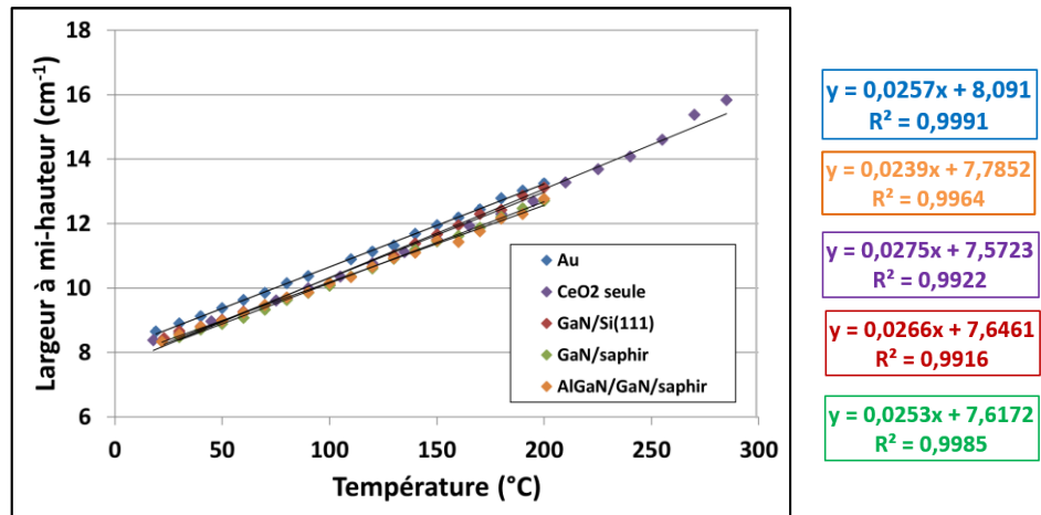
Figure III-37 : Courbes de calibration de \Gamma du \text{CeO}_2 déposé sur plusieurs types de surface en fonction de la température.
