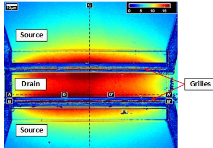
Figure I-30 : Cartographie thermique obtenue par thermorélectance sur un HEMT AlGaIn/GaN sur SiC à P_{diss} = 1,3 \text{ W} [96].
