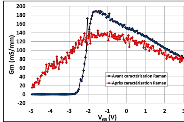
Figure III-56: Transconductance G_m ( V_{GS} , V_{DS} = 15 \text{ V} ) d'un HEMT AlInN/GaN sur un substrat de saphir, avant (en bleu) et après l'étude N°4 (en rouge).
