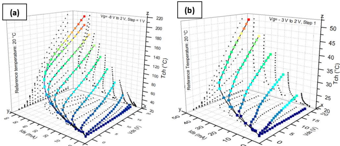
Figure I-16 : Caractéristiques I_{DS}-V_{DS}-T_{ch} pour des HEMTs AlGaN/GaN (a) sur substrat saphir et (b) SiC [51].
