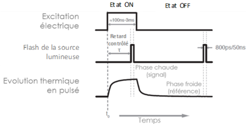
Figure II-1 : Principe de la mesure par thermoréfectance en mode pulsé. Le retard \tau du flash de la DEL est synchronisé avec l'excitation électrique afin de caractériser le composant à différents stades du pulse. L'élévation de température est déterminée en calculant le rapport des réflectivités entre les phases chaude et froide [22].
