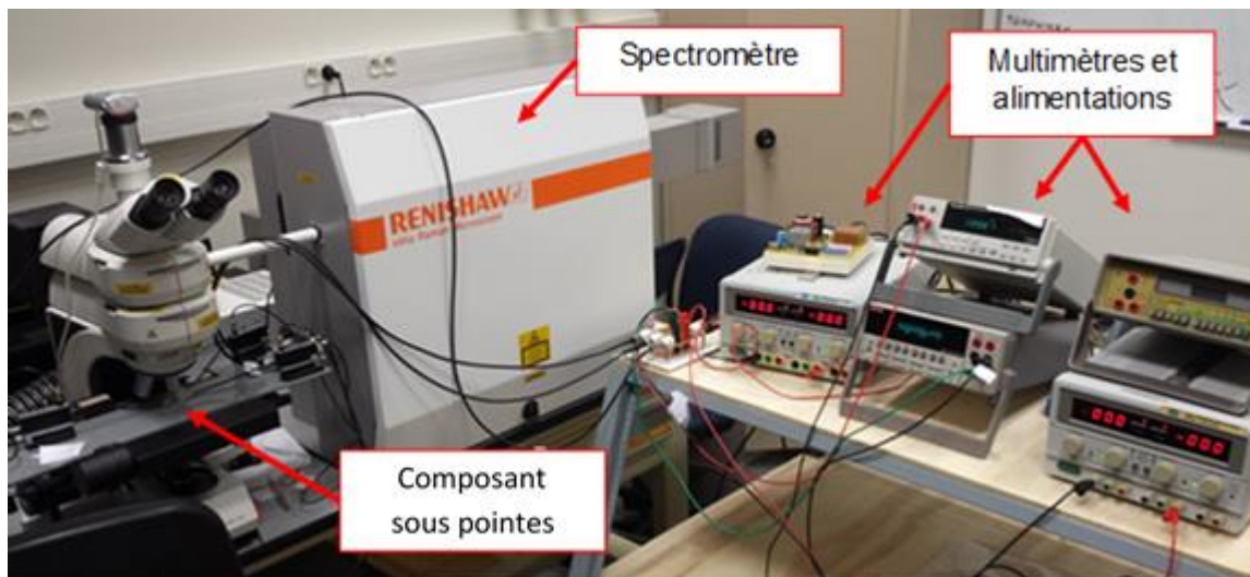
Figure III-4 : Banc de mesure de caractérisation thermique des transistors en fonctionnement.
