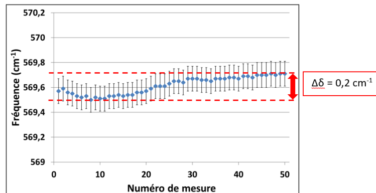
Figure III-5 : Résultat de l'itération de 50 mesures de fréquence Raman sur du GaN/saphir. Conditions de mesure : 25 °C, temps d'acquisition = 120 s, P_{\text{laser}} = 10 \text{ mW} , \lambda_{\text{inc}} = 514 \text{ nm} , objectif x50 et mode Extended .
