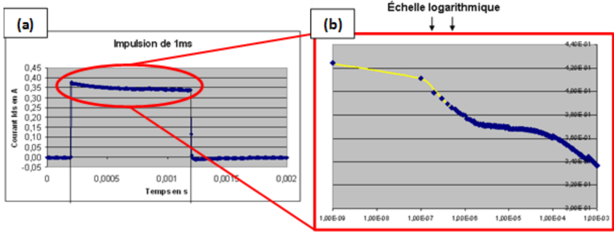
Figure I-24 : Forme temporelle d'une impulsion du courant I_{ds} lors de la caractérisation d'un transistor en régime dynamique (pulsé) [78].
