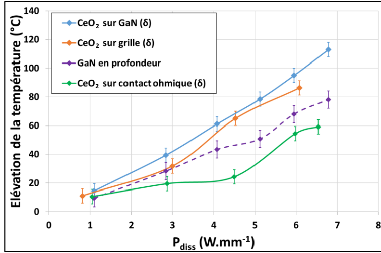
Figure III-44 : Élévation de la température mesurée sur les particules de \text{CeO}_2 déposées sur le GaN, la grille et un contact ohmique, ainsi que du GaN en profondeur. Les mesures sur le \text{CeO}_2 ont été réalisées par suivi de \delta . Conditions de mesure : \lambda_{\text{inc}} = 633 \text{ nm} , P_{\text{laser}} = 5 \text{ mW} , temps d'acquisition = 20 s, objectif x50 LDF et en mode Static .
