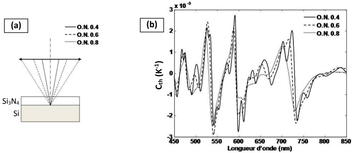
Figure II-13 : (a) Schéma des trois objectifs d'ouvertures numériques différentes utilisés collectant la lumière selon des cônes variables. (b) Spectres de thermoréflectance C_{th} en fonction de \lambda_{inc} mesurés sur une résistance en polysilicium couvert d'une couche de Si 3 N 4 et de polyamide dissipant une puissance de 0,12 \text{ mW.mm}^2 ( \Delta T_{\text{surface}} = 100^\circ\text{C} ). [92].
