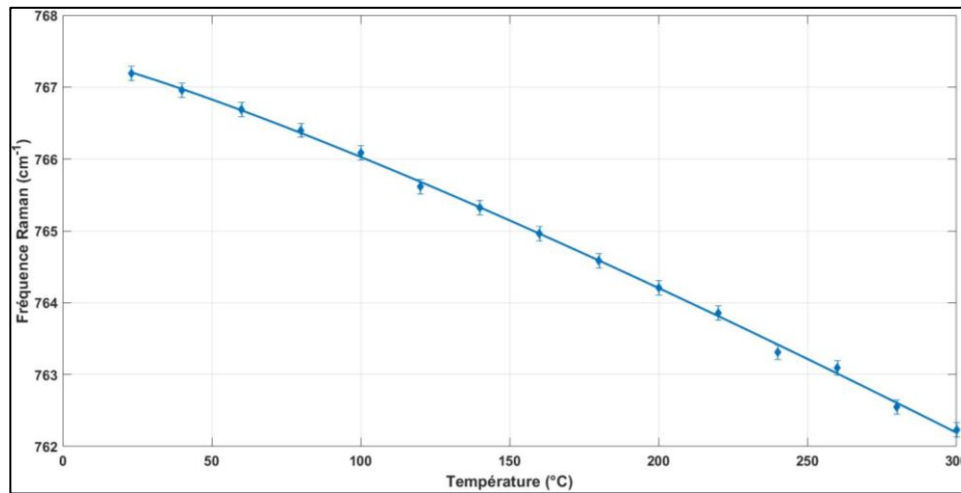
Figure III-26 : Courbe de calibration du mode \delta (E 2 low) du SiC-6H du Golden Unit. Conditions : \lambda_{\text{inc}} = 633 nm, temps d'acquisition = 60 s, P_{\text{laser}} = 10 mW, objectif x50 et en mode Static .
