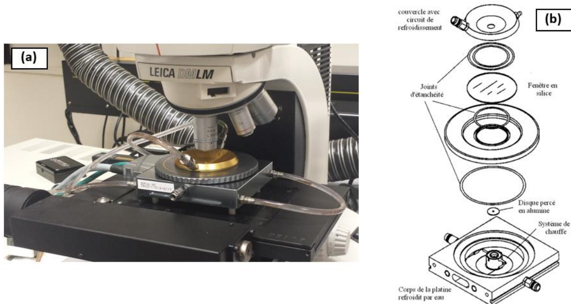
Figure III-3 : (a) Platine chauffante Linkam TS 1500 placée sous le spectromètre Raman. (b) Schéma des éléments constitutifs de la cellule [181].
