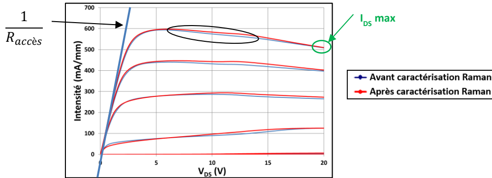
Figure III-49 : Caractéristiques I_{DS} ( V_{DS} , V_{GS} ) d'un HEMT AlInN/GaN avant (en bleu) et après l'étude N°1 (en rouge). V_{DS} varie de 0 à 20 V par pas de 200 mV et V_{GS} évolue de -6 à 1 V par pas de 1 V.
