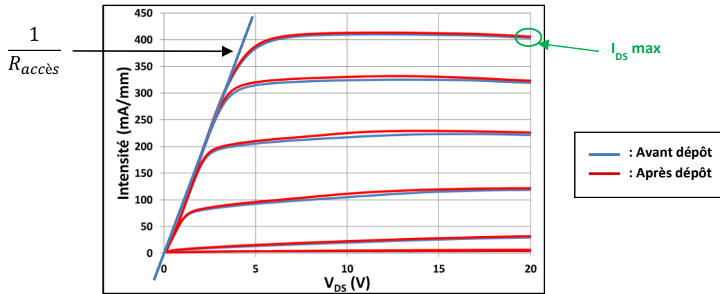
Figure III-42 : Caractéristiques I_{DS} ( V_{DS} , V_{GS} ) d'un HEMT AlGaIn/GaN sur substrat saphir avant (en bleu) et après dépôt de particules de \text{CeO}_2 par spin-coating (en rouge). V_{DS} varie de 0 à 20 V par pas de 200 mV et V_{GS} évolue de - 6 à 1 V par pas de 1 V.
