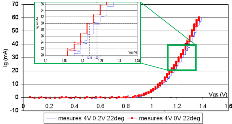
Figure I-22 : Mesure de I_g en fonction de V_{gs} pour deux polarisations de repos différentes ( V_{DS0} = 4 V et V_{GS0} = 0 V en rouge et V_{DS0} = 4 V et V_{GS0} = 0,2 V en bleu) avec une température de semelle de 22 °C [78].
