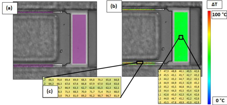
Figure II-10 : (a) Étape de sélection des régions d'intérêt et de masque des valeurs. (b) Thermographie pixel par pixel des zones d'intérêt présélectionnées. (c) Capture d'écran des valeurs \Delta T extraites sous format Excel. Les valeurs à gauche et à droite correspondent respectivement à des zones sur la plaque de champ et sur l'interconnexion de grilles.
