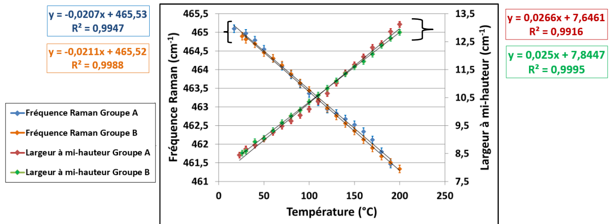
Figure III-34 : Courbes de calibration des paramètres \delta et \Gamma des particules de \text{CeO}_2 déposées sur du GaN sur un substrat de Si (111), à faible amas (points jaunes et verts) et pour un amas plus important (points bleus et rouges).
