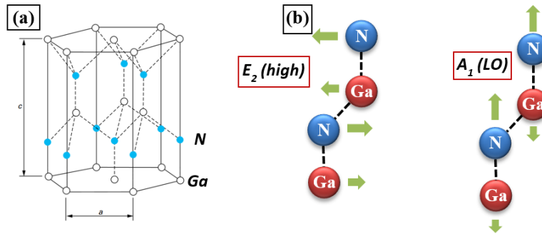
Figure I-33 : (a) Structure hexagonale (wurtzite) du GaN [24] et (b) schéma des modes de vibration atomique (phonons optiques) E_2h et A_1\text{LO} .
