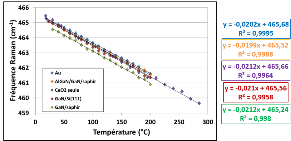
Figure III-36 : Courbes de calibration du \delta de \text{CeO}_2 déposé sur plusieurs types de surface en fonction de la température.
