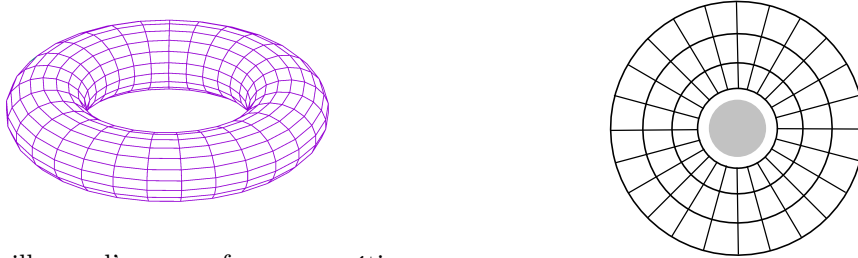
(b) Maillage du plan poloïdal.
