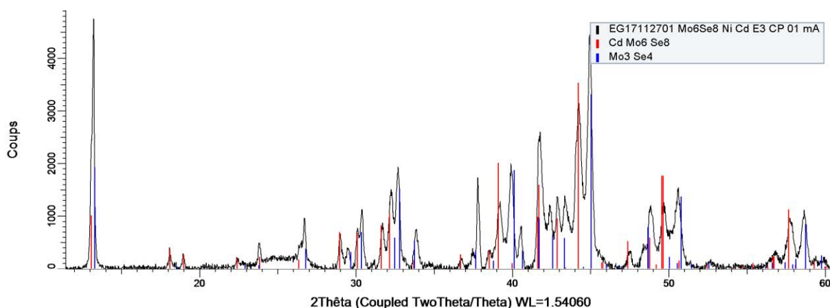
Figure IV-XV : diagramme de DRX après intercalation par chronopotentiométrie à -0,1 \text{ mA} de \text{Ni}^{2+}/\text{Co}^{2+} dans \text{Mo}_6\text{Se}_8
