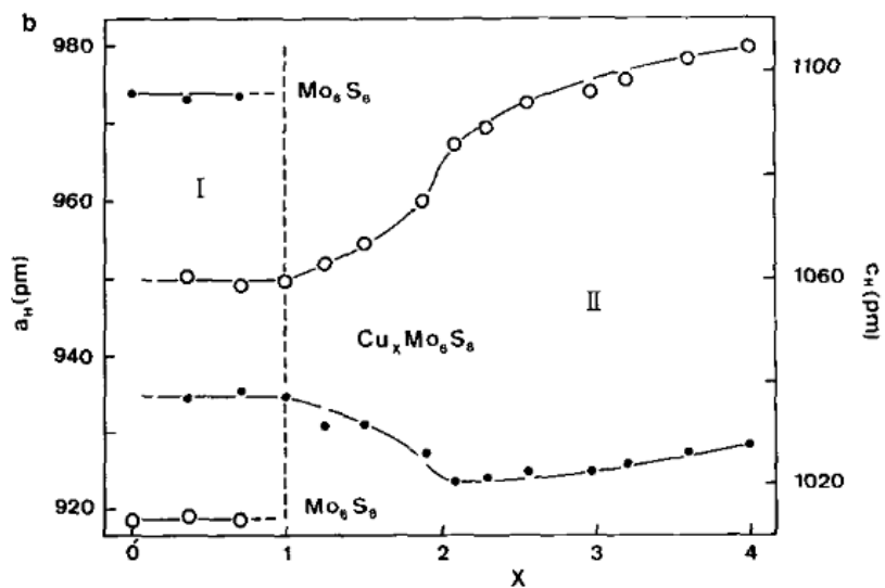
Figure I-XIV : évolution des paramètres de maille hexagonaux ( a_H = \circ , c_H = \bullet ) en fonction de x [Fisc. 1993]
