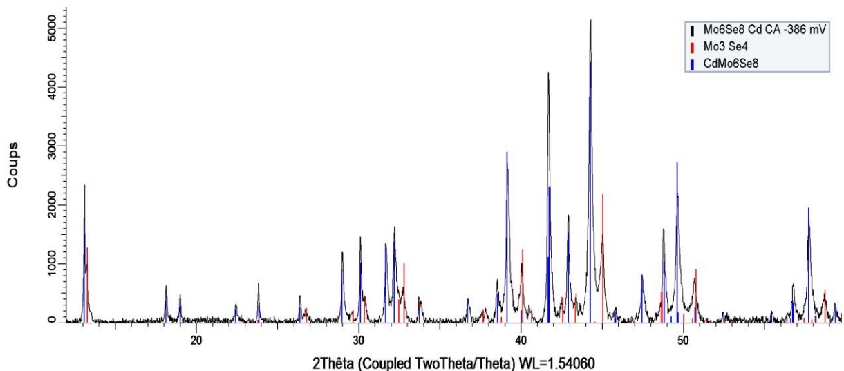
Figure III-IX : diagramme DRX après intercalation de Cd^{2+} à 0,1 M Mo_6Se_8 à -0,386 V vs. Ag/AgCl à T_{amb}
