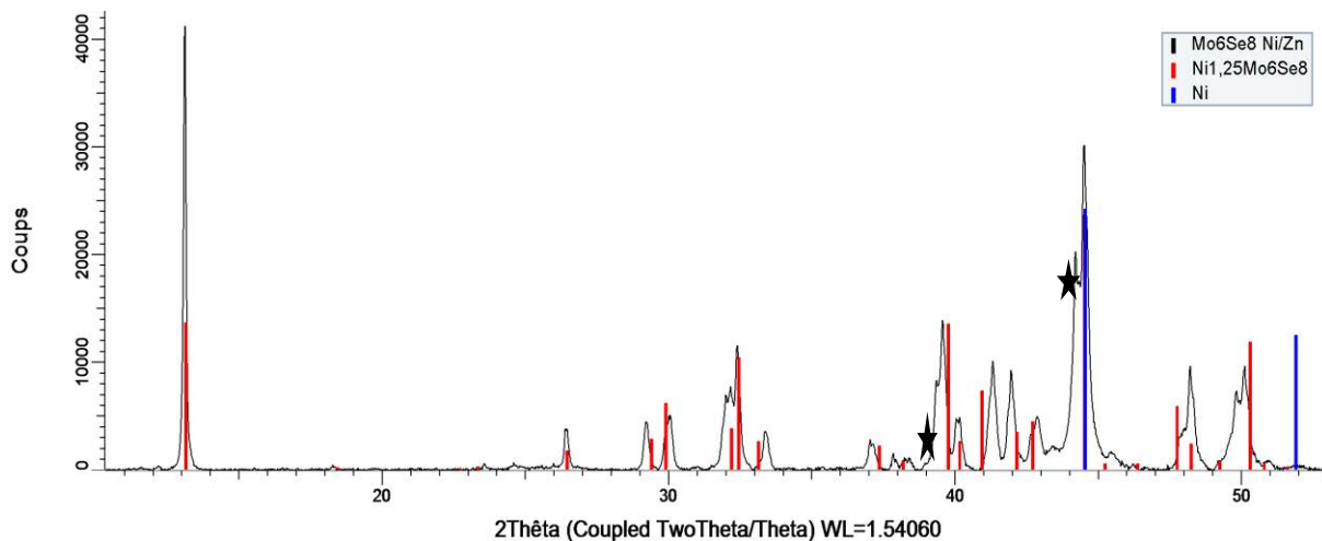
Figure IV-XXXIV : diagramme de DRX après intercalation par chronoampérométrie à -0,630 V de Ni 2+ /Zn 2+ à 0,1 M dans Mo 6 Se 8 à T amb . Les pics signalés par * correspondent au porte-échantillon
