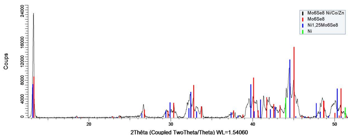
Figure V-XIII : diagramme de DRX après chronopotentiométrie de \text{Ni}^{2+}/\text{Co}^{2+}/\text{Zn}^{2+} à -0,1 mA dans \text{Mo}_6\text{Se}_8
