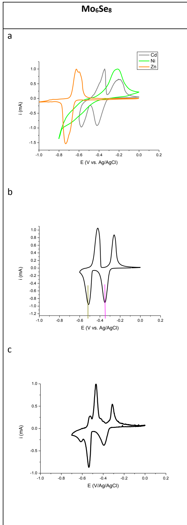
Figure V-XVIII : intercalation d'un électrolyte tri-cationique Ni 2+ /Cd 2+ /Zn 2+ dans Mo 6 Se 8 à 0,1 M et à 0,1 mV/s; a – superposition des signaux enregistrés sur des solutions mono-cationiques ; b – courbe expérimentale obtenue avec les solutions tri-cationiques pour l'électrode A et c- électrode B
