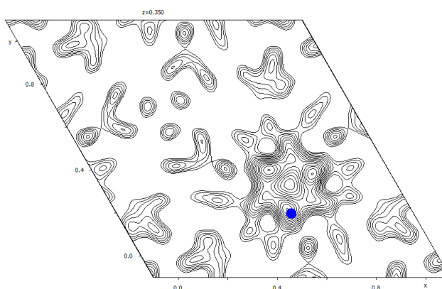
Figure VI-XXV : Carte de Fourier différence du composé Cd_2Mo_6S_8 pour la phase pauvre, exprimée en densité électronique du cadmium ; le point bleu correspond à la position du cadmium dans Cd_1Mo_6S_8 d'après Levi et al. [Levi 2009]
