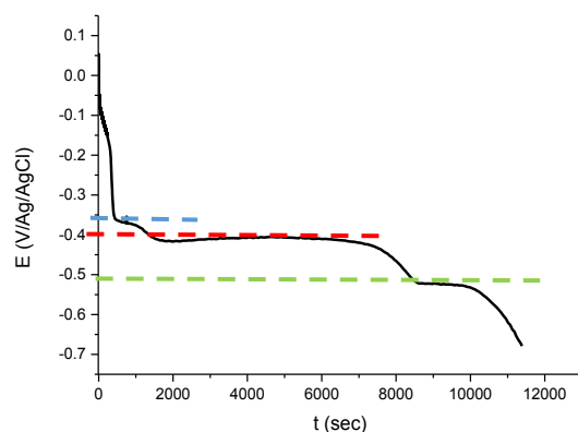
Figure IV-XIV : chronopotentiométrie d'intercalation de \text{Ni}^{2+}/\text{Cd}^{2+} dans \text{Mo}_6\text{Se}_8 à -0,1\text{mA}
