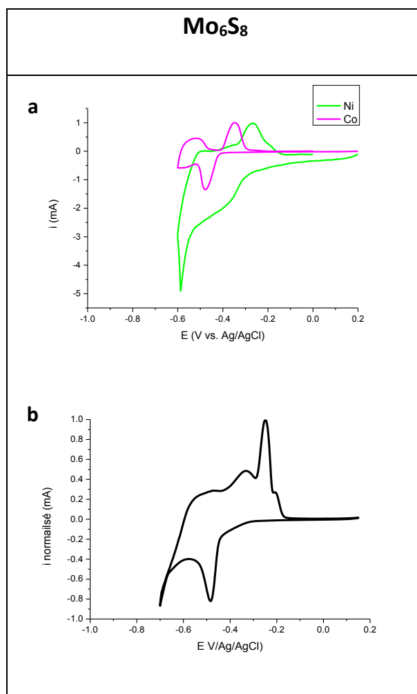
Figure IV-XVII : intercalation d'un électrolyte bi-cationique Ni 2+ /Co 2+ à 0,1 M dans Mo 6 S 8 et Mo 6 Se 8 à 0,1 mV/s: a superposition des signaux enregistrés sur des solutions mono-cationiques; b courbes expérimentales obtenues avec les solutions bi-cationiques à 0,1 M à 0,1 mV/s à T amb
