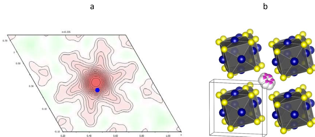
Figure VI-XXIV : \text{CdMo}_6\text{S}_8 . Partie a) Carte de Fourier différence de la cavité 1, plan x,y , z=0,335 dans la maille hexagonale, position affinée de Cd représentée par un point bleu [Levi 2009], positive cutoff 14,2 \text{ e}/\text{\AA}^3 , positive contour 0,5 \text{ e}/\text{\AA}^3 . Partie b) Représentation graphique de la structure \text{CdMo}_6\text{S}_8 dans la maille rhomboédrique
