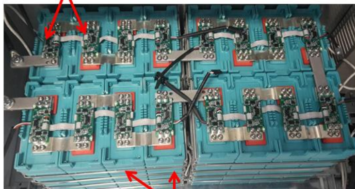
Figure V-27: Cellules de batteries reliées en série
