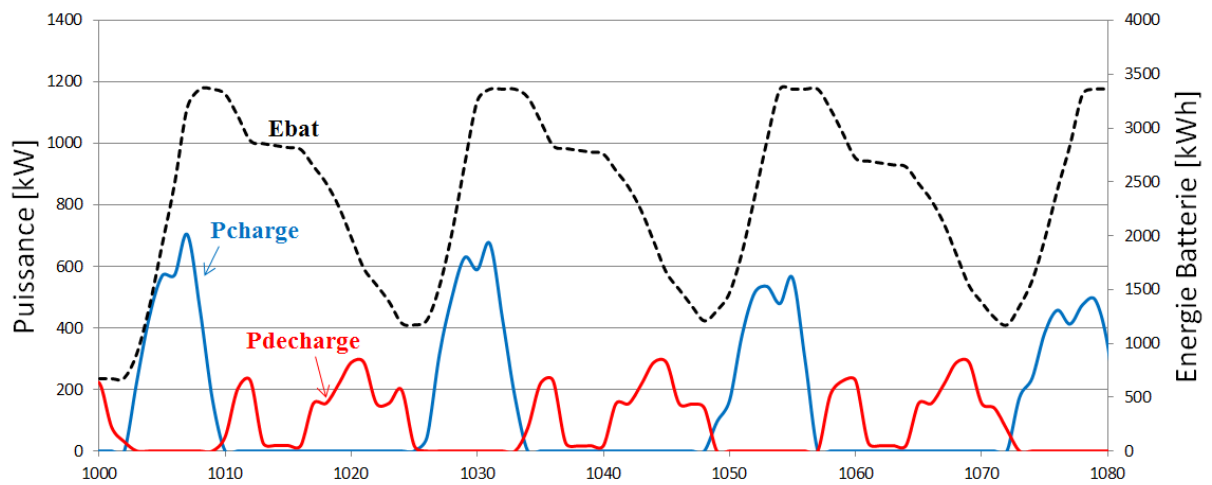
Figure V-13: Flux énergétique dans la batterie
