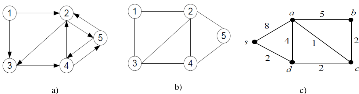
Figure IV-13 : Graphes a) orienté, b) non orienté, c) pondéré
